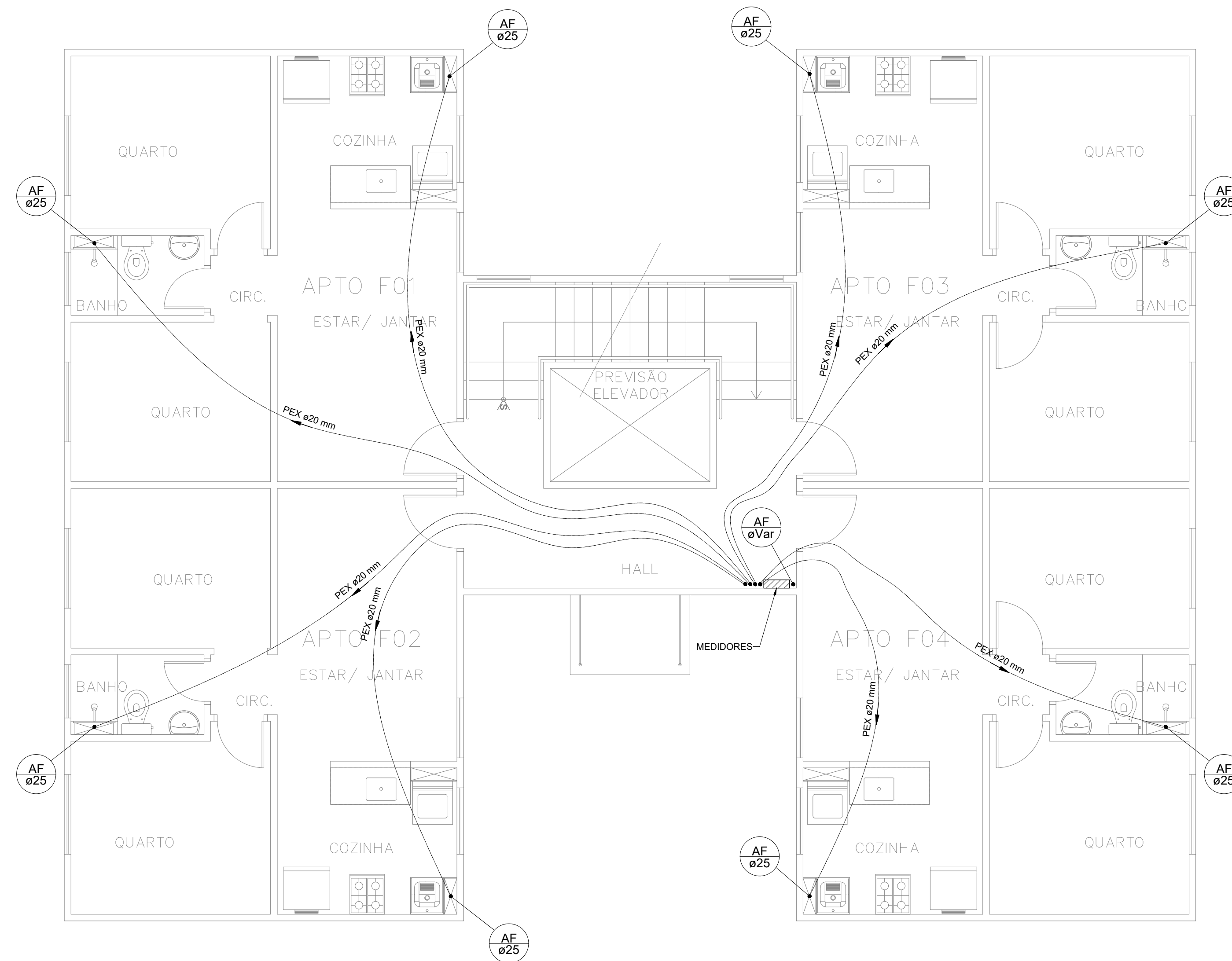
PLANTA DE DISTRIBUIÇÃO HIDRÁULICA - PAV. TIPO BLOCOS 01 AO 15 ESCALA 1:50
