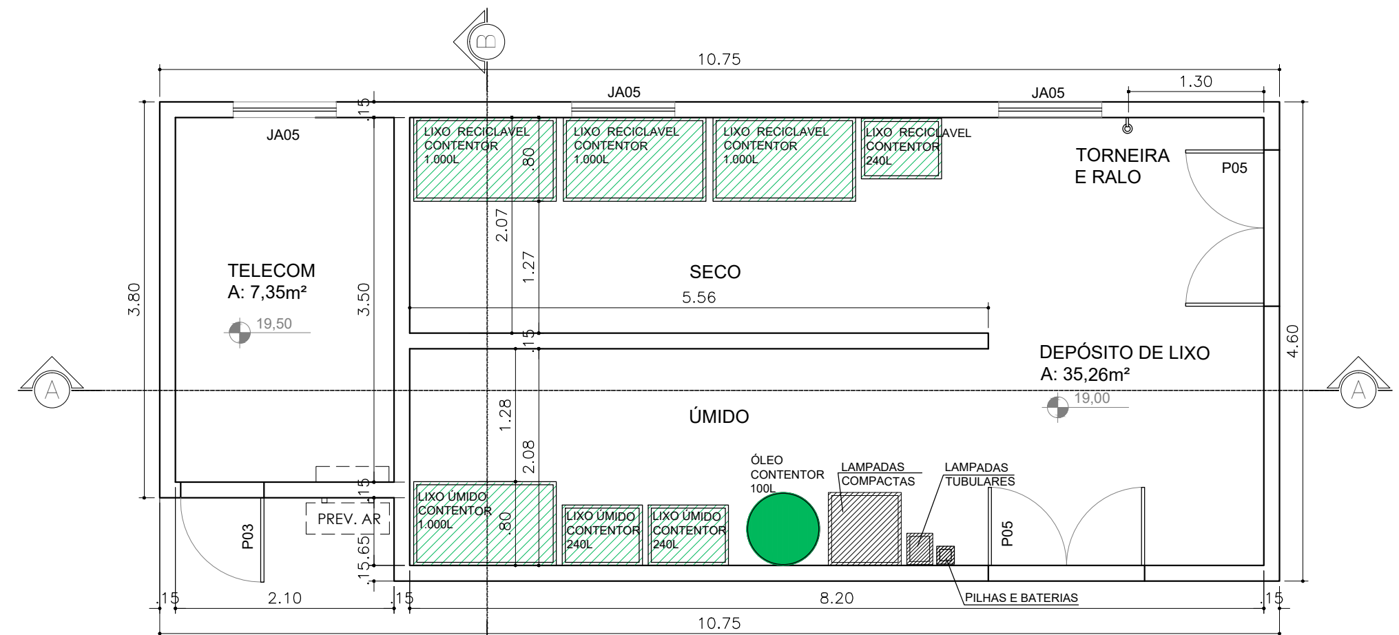
PLANTA - SALA TELECOM E DEPÓSITO DE LIXO
