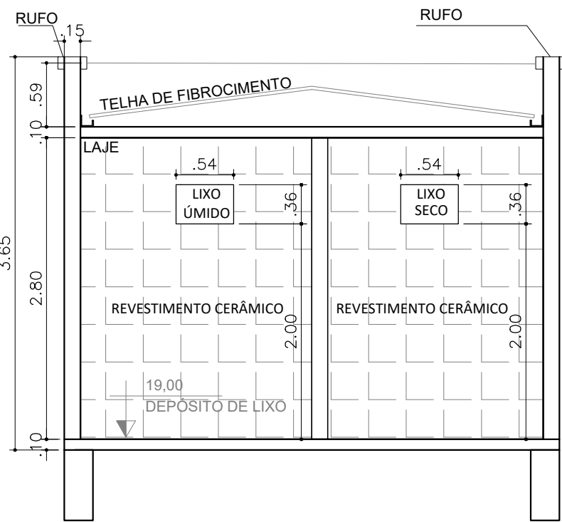
CORTE BB - DEPÓSITO DE LIXO
