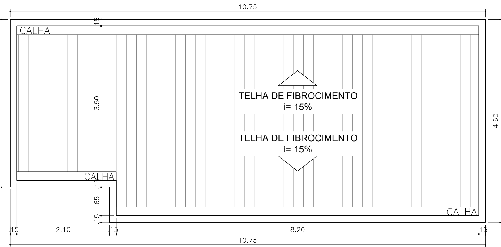
PLANTA COBERTURA - TELECOM E DEPÓSITO DE LIXO
