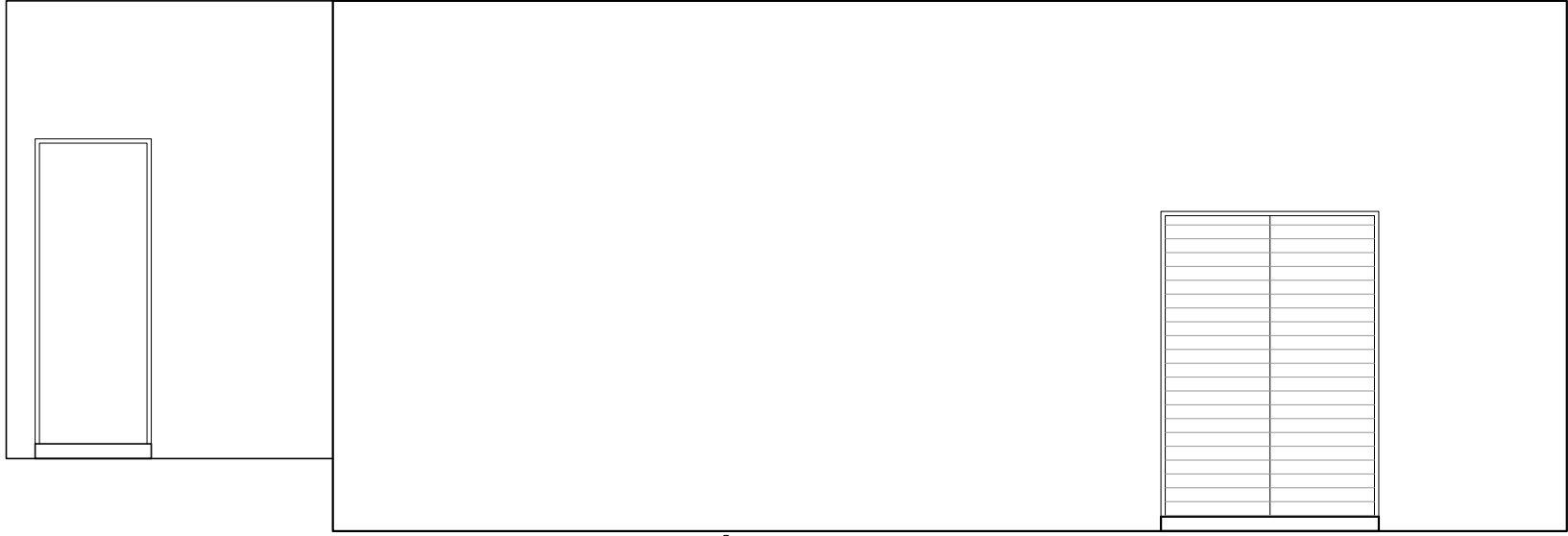
ELEVAÇÃO A - TELECOM E DEPÓSITO DE LIXO
