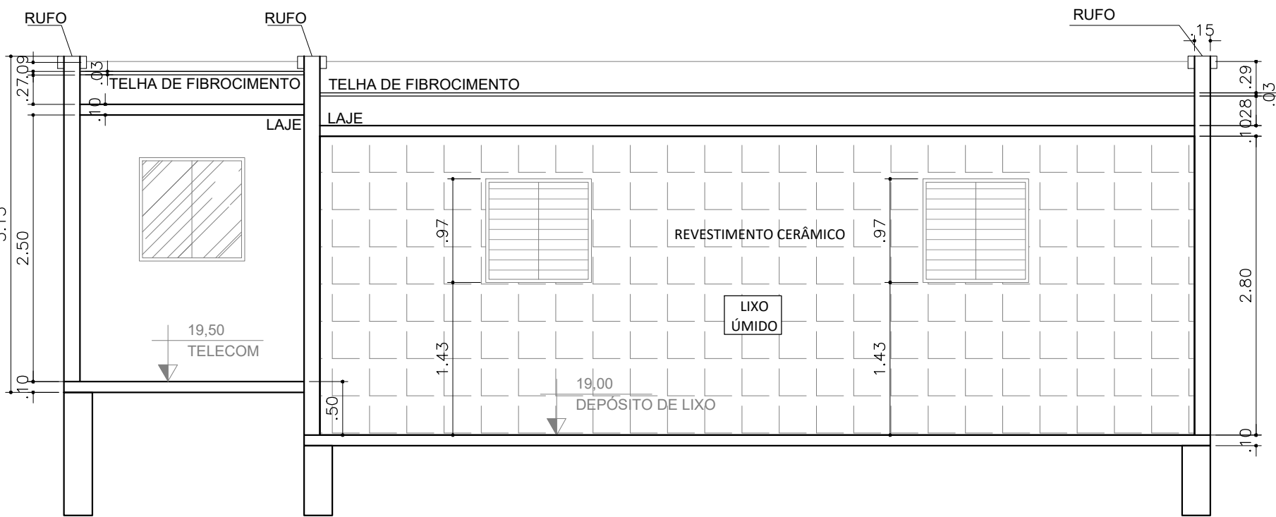
CORTE AA - TELECOM E DEPÓSITO DE LIXO
