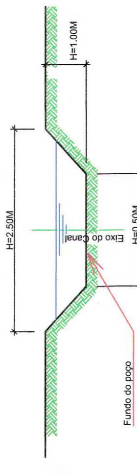
CORTE TRANSVERSAL POÇO DE SECATAÇÃO
