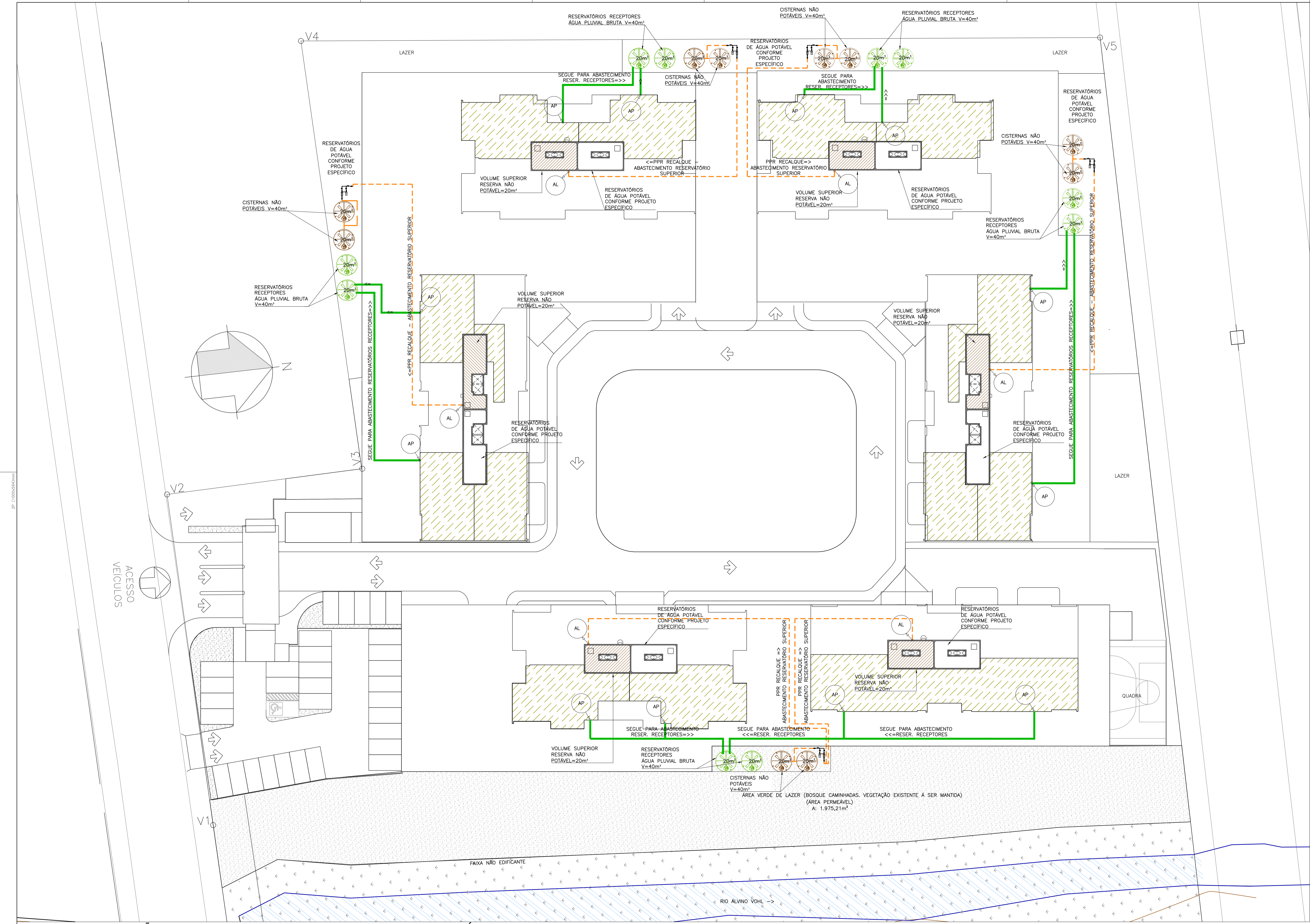
PLANTA DE IMPLANTAÇÃO - CROQUI GERAL DO SISTEMA DE REAPROVEITAMENTO DE ÁGUA DA CHUVA
