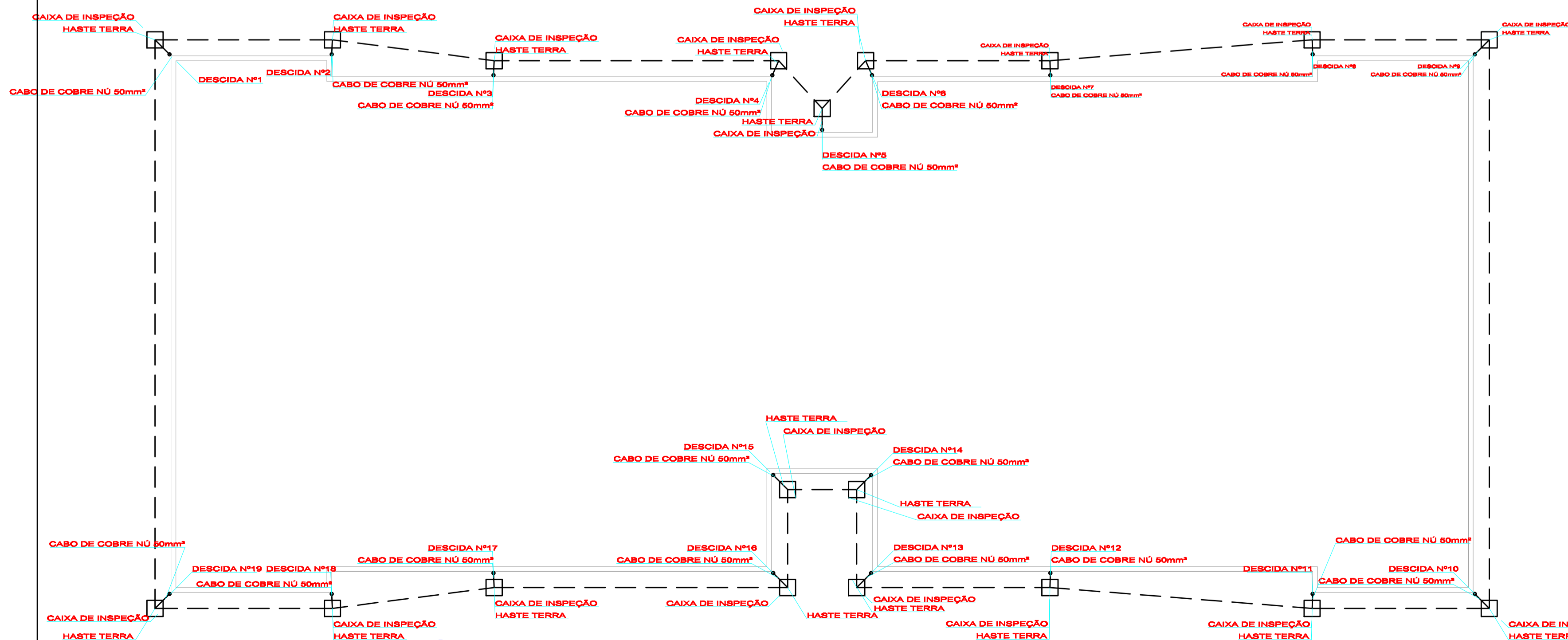
TÉRREO bloco 01, 02 e 03 escala 1/200
