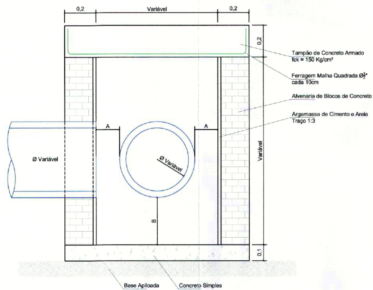
Corte BB'
