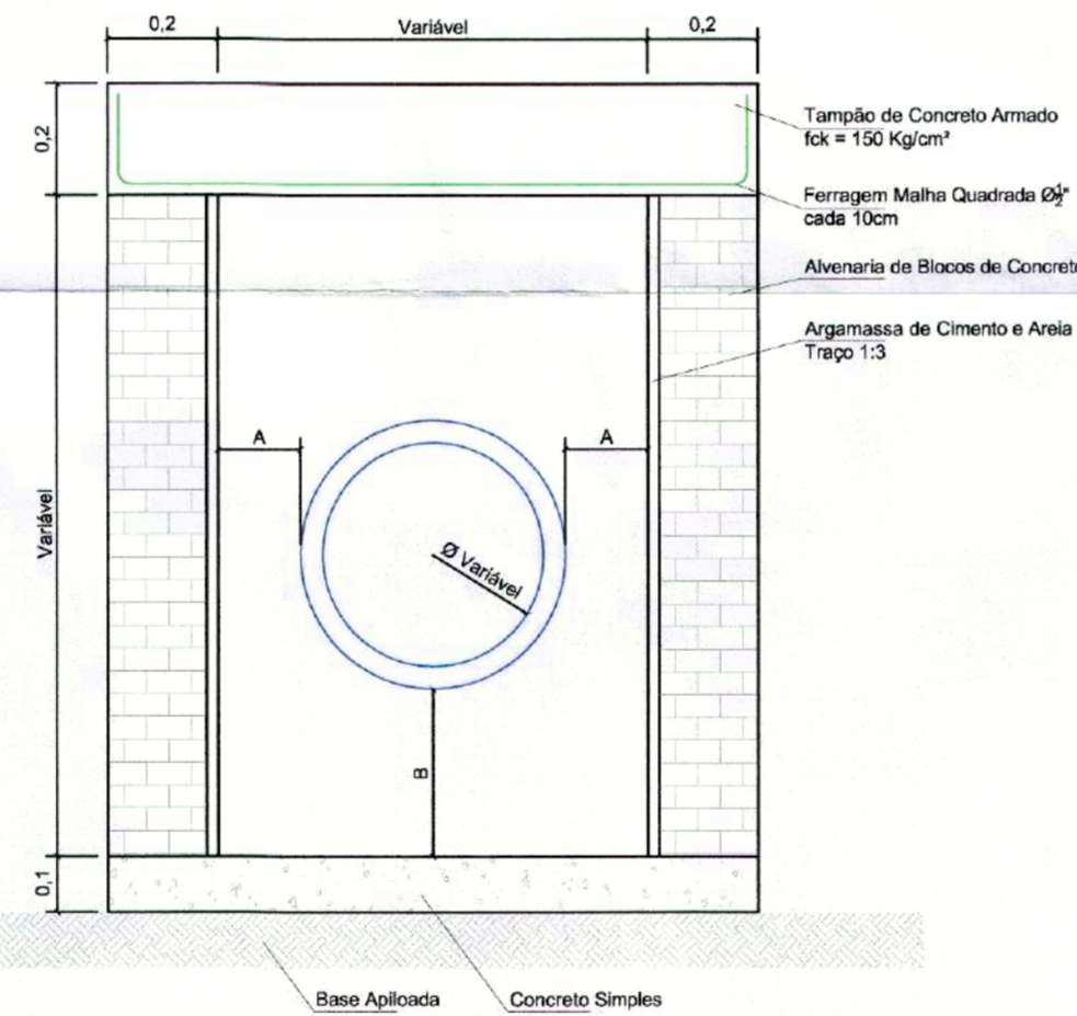
Corte BB'
