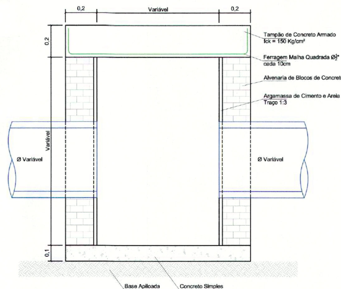
Corte BB'
