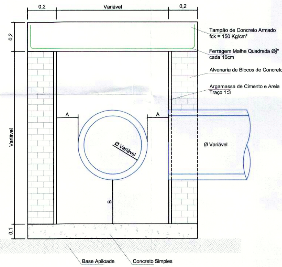
Corte BB'
