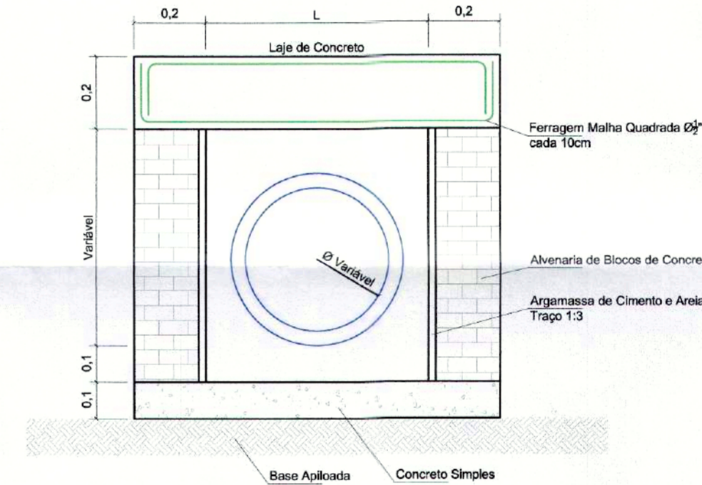
Corte AA'
