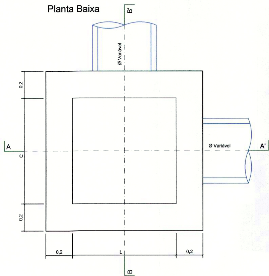
Corte AA'
