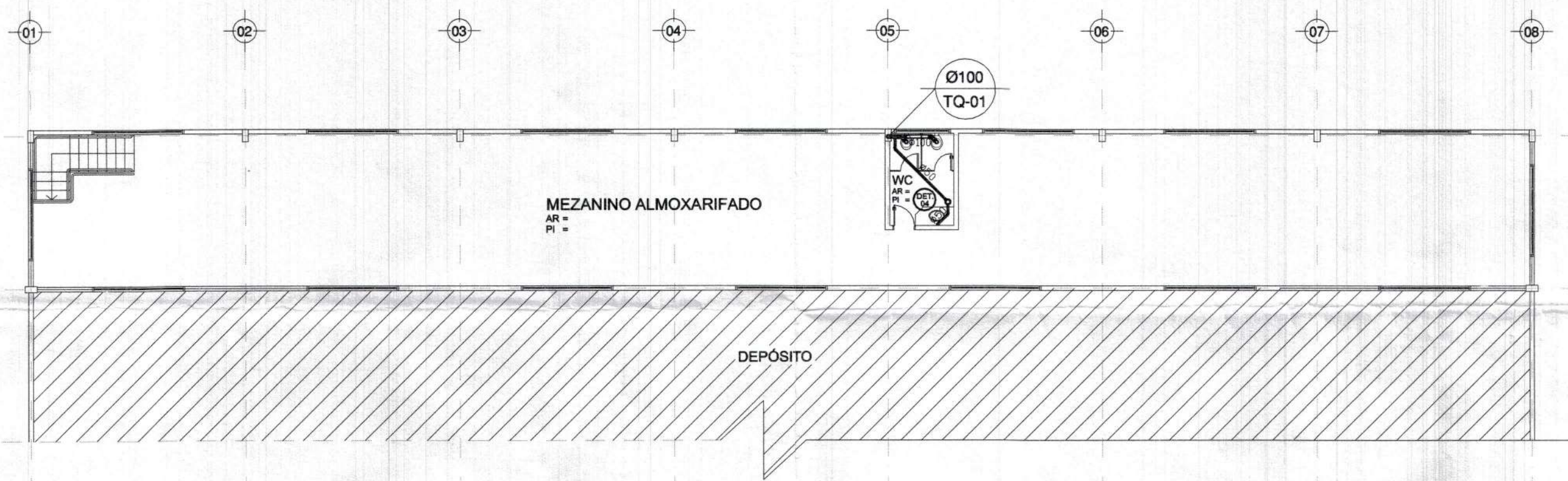
PLANTA BAIXA MEZANNO DISTRIBUIÇÃO REDE ESGOTO ESCALA: 1/150
