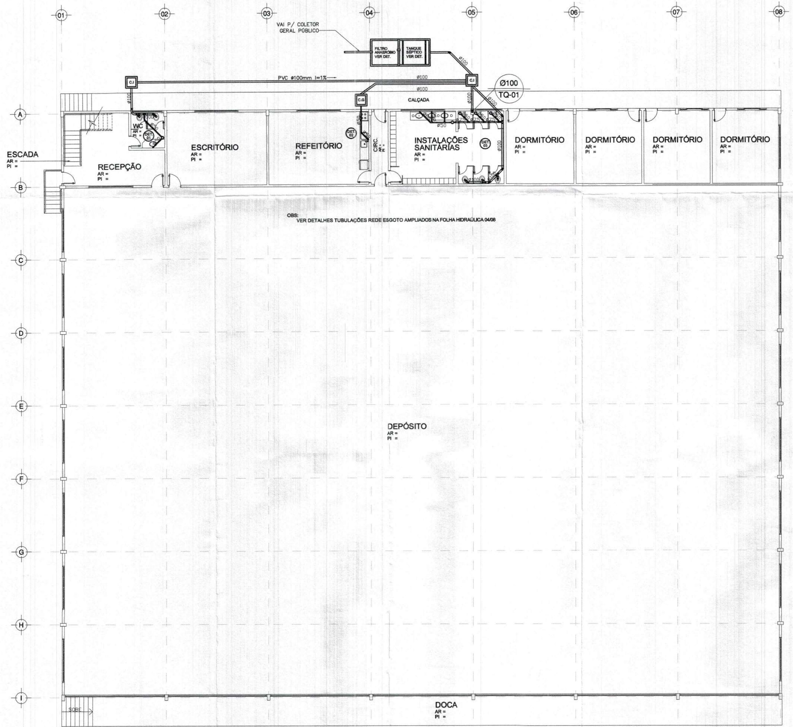
PLANTA BAIXA GALPÃO DISTRIBUIÇÃO REDE ESGOTO ESCALA: 1/150
