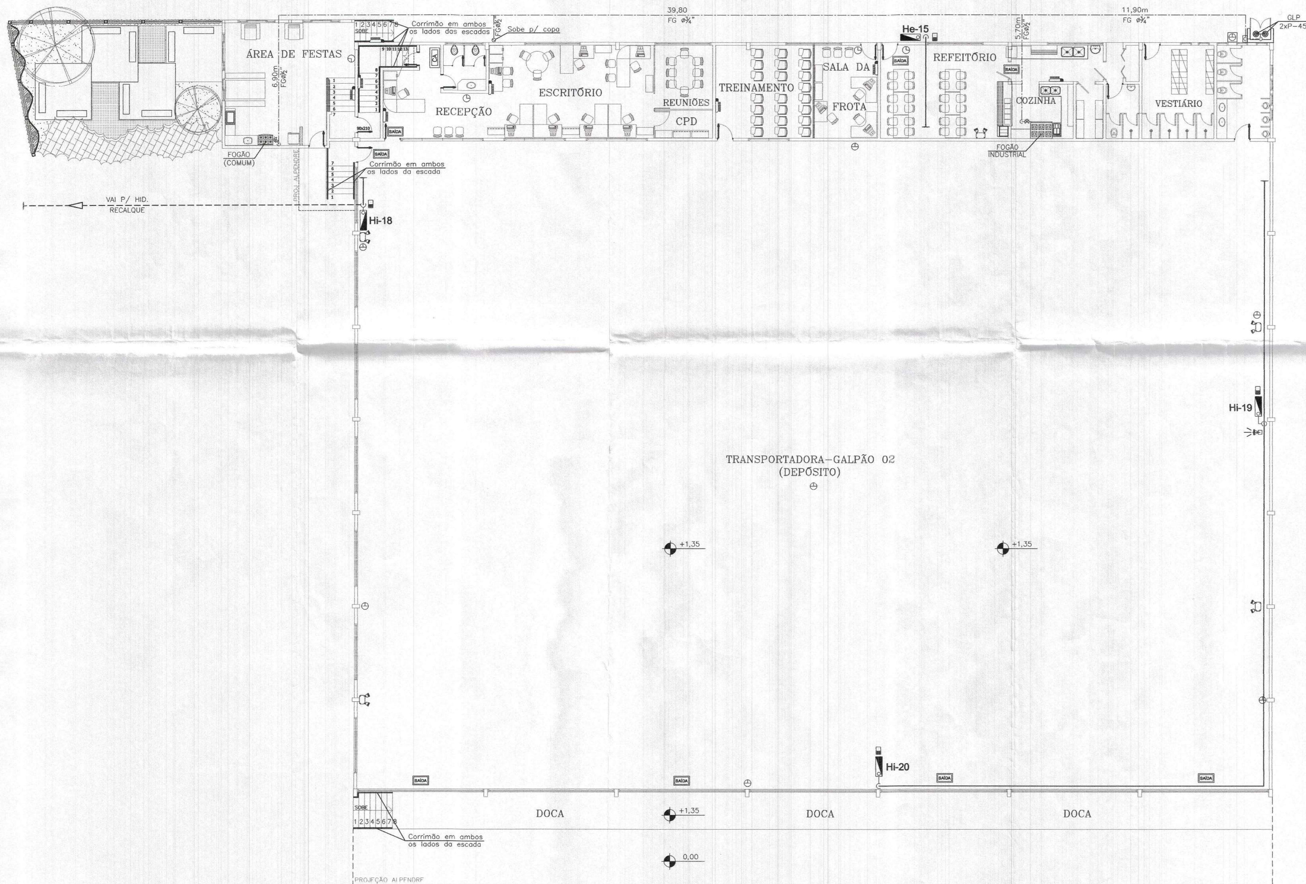
PLANTA BAIXA TÉRREO ESC 1/125
