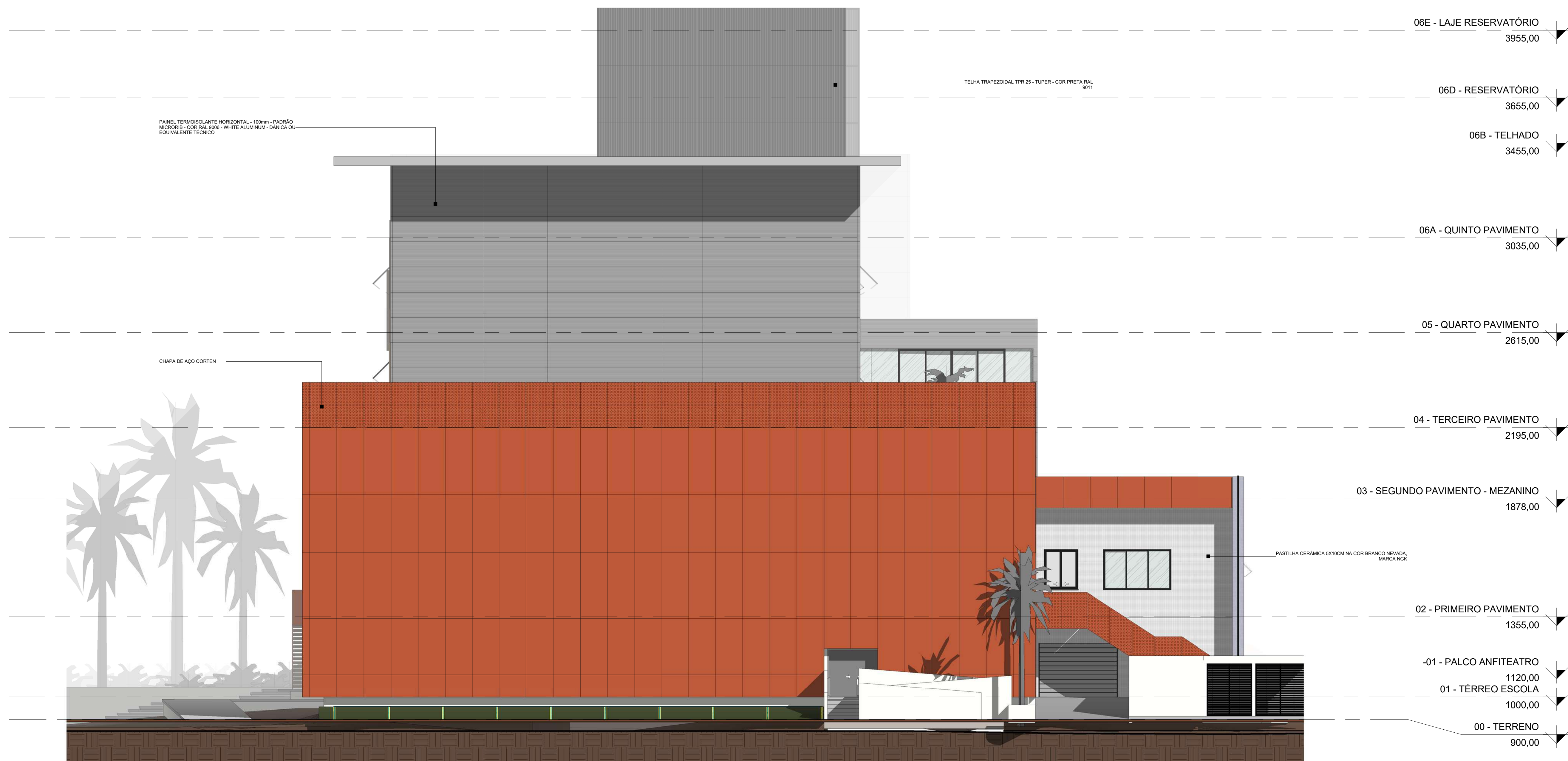
2 ELEVÇÃO SUDESTE Escala 1 : 100
