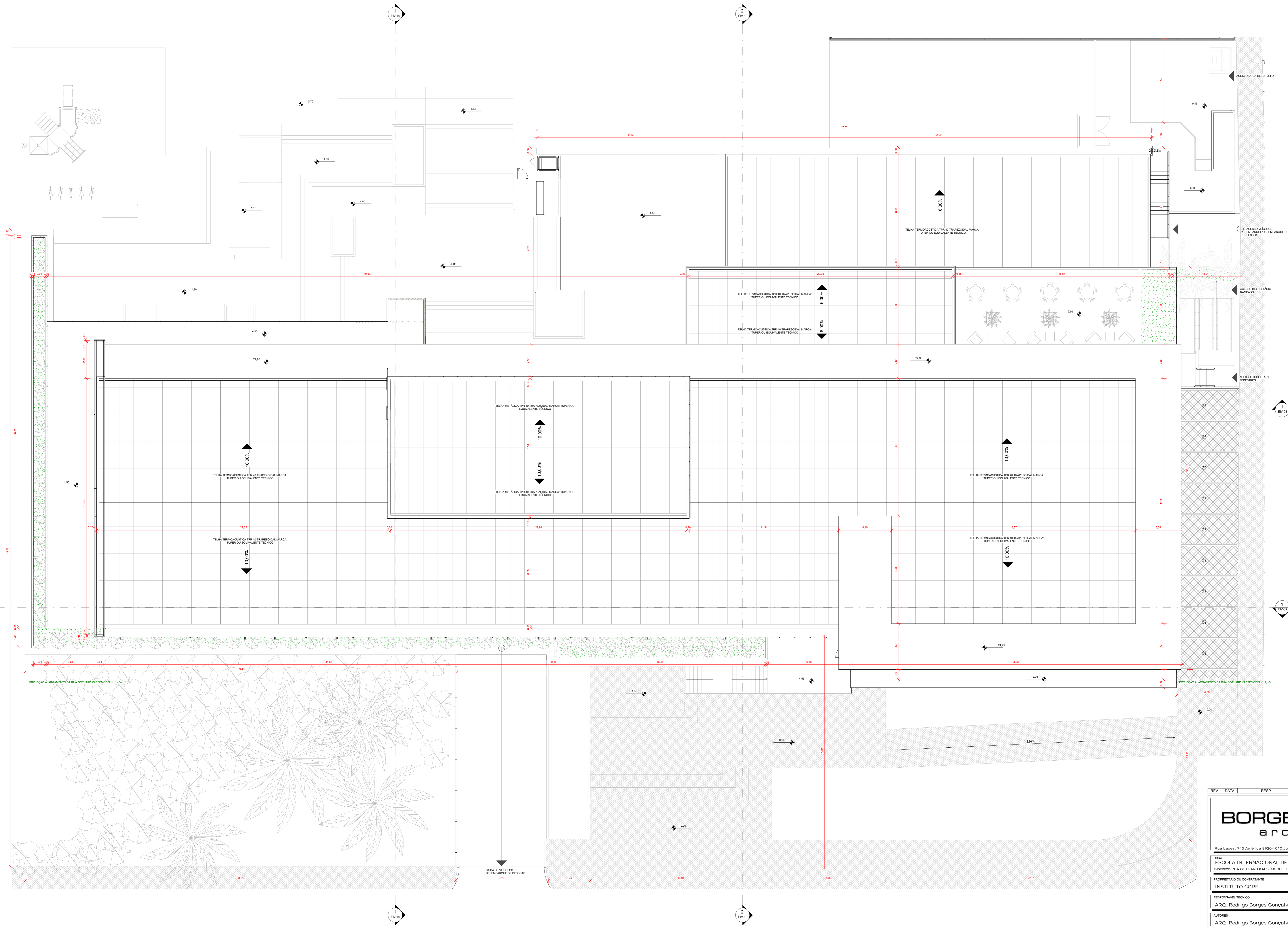
PLANTA ESQUEMÁTICA - COBERTURA Escala 1:100
