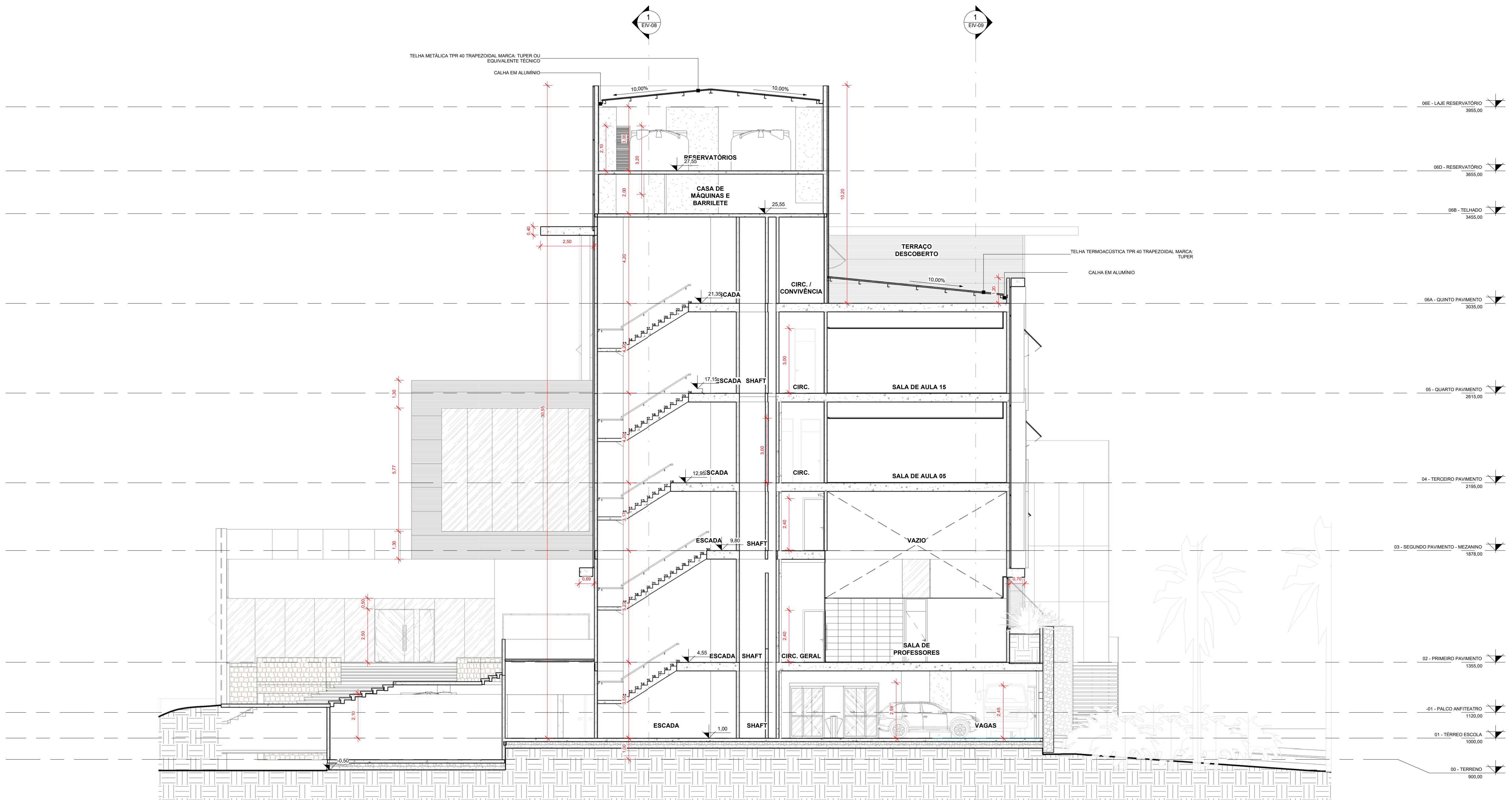
CORTE ESQUEMÁTICO TRANSVERSAL 01 Escala 1 : 100
