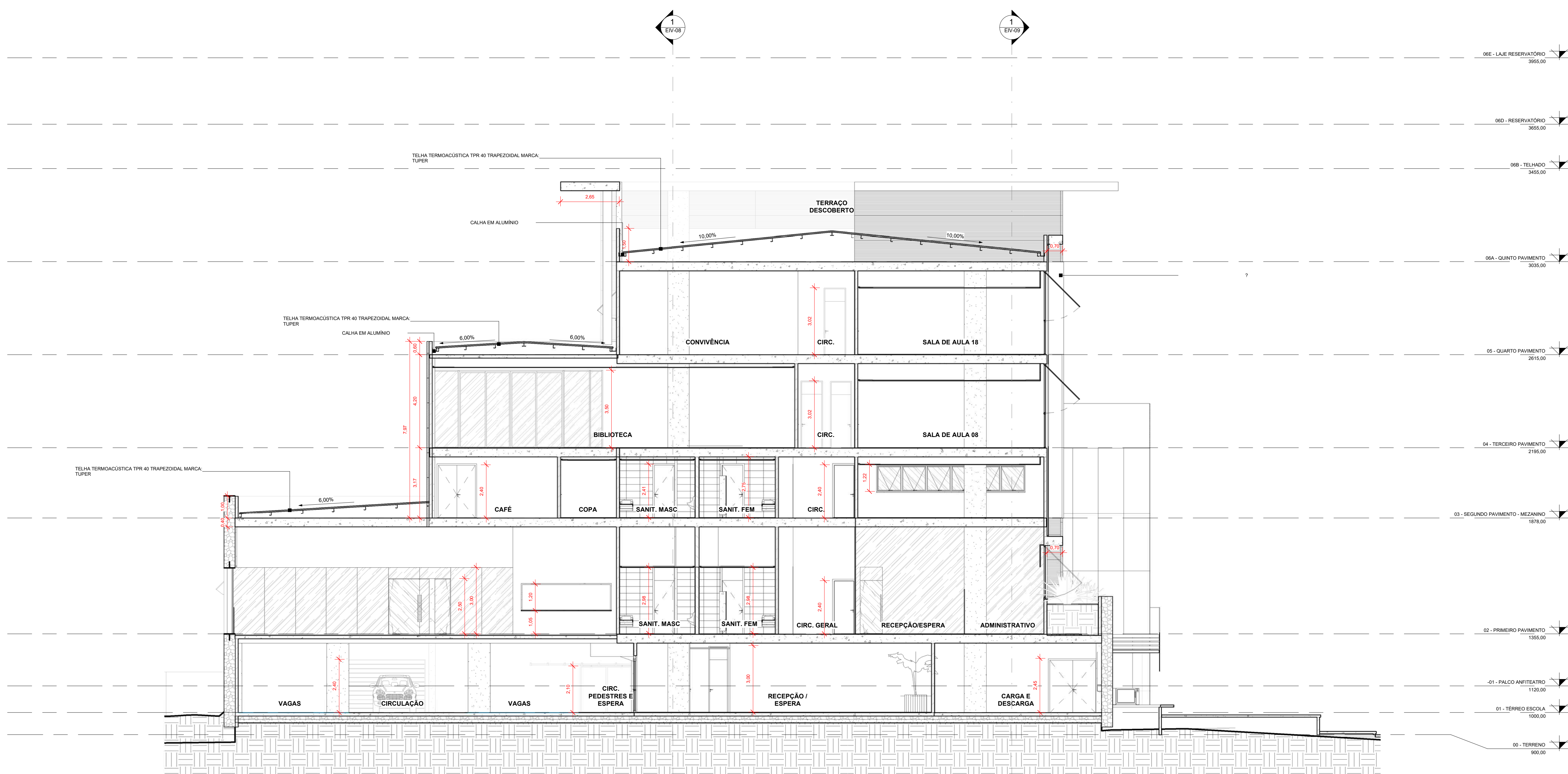
CORTE ESQUEMÁTICO TRANSVERSAL 02 Escala 1 : 100
