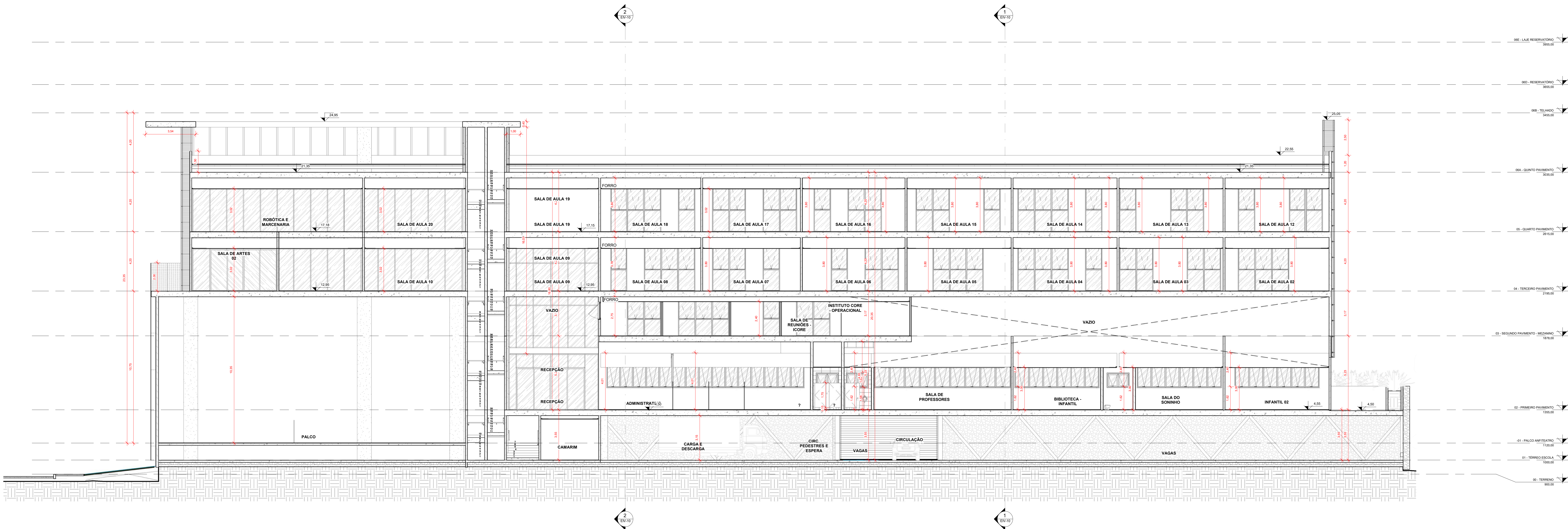
1 CORTE ESQUEMÁTICO LONGITUDINAL 02 Escala 1 : 100
