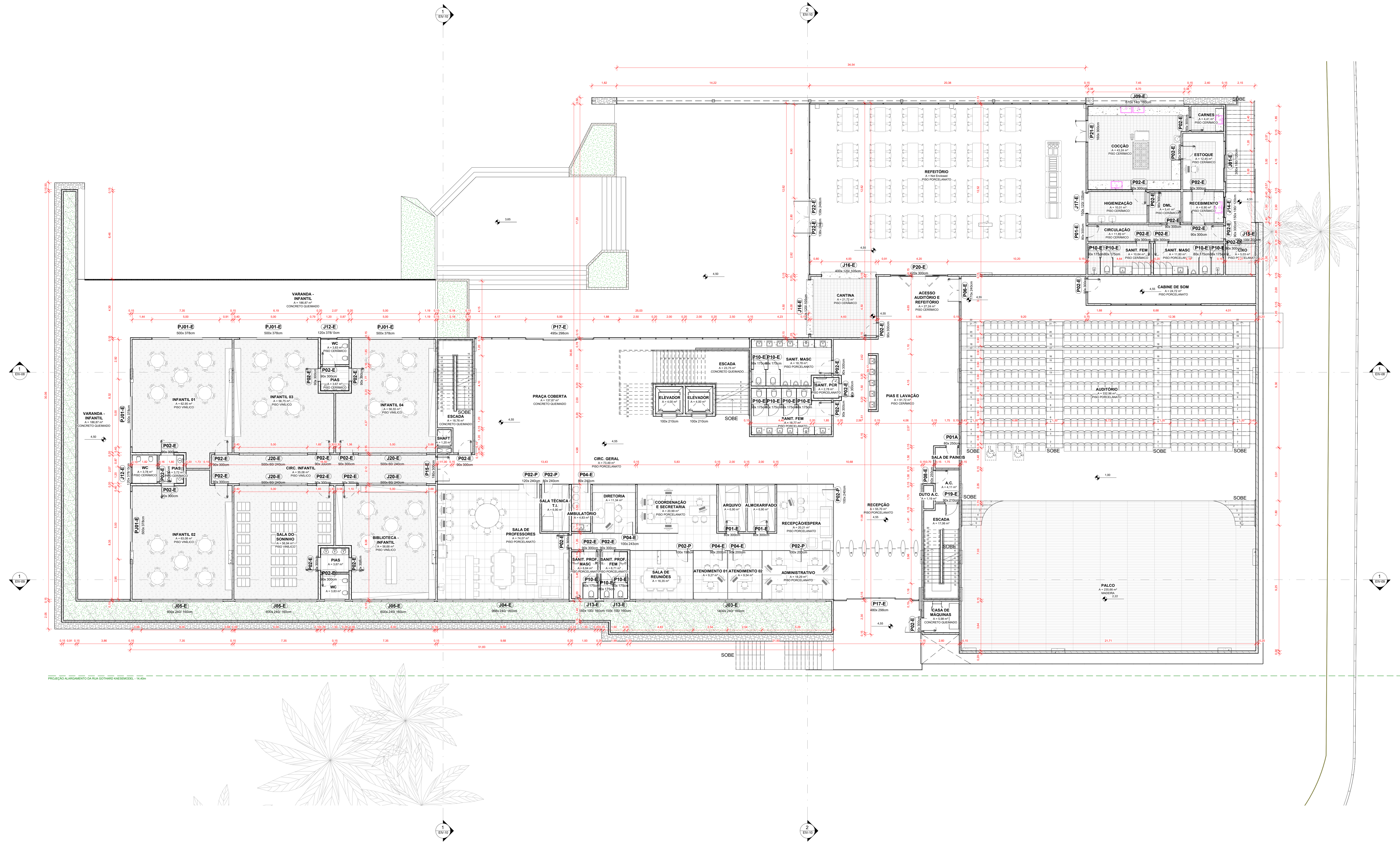
1 PLANTA BAIXA - PRIMEIRO PAVIMENTO Escala 1:100
