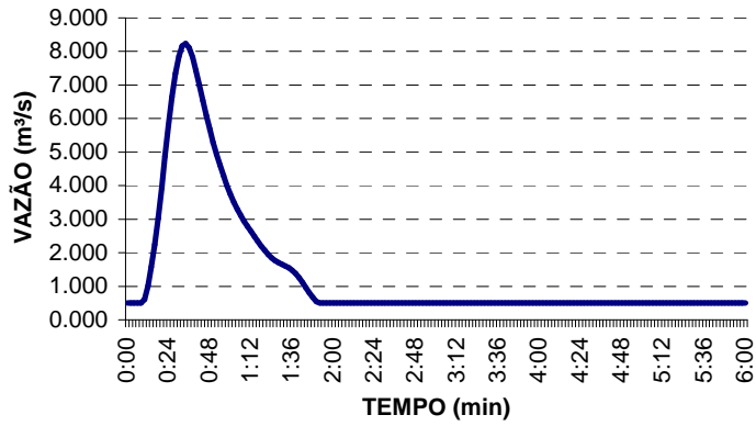
HIDROGRAMA 07
