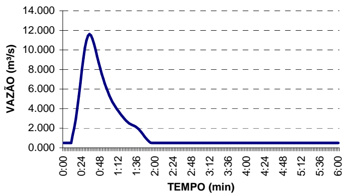
HIDROGRAMA 06
