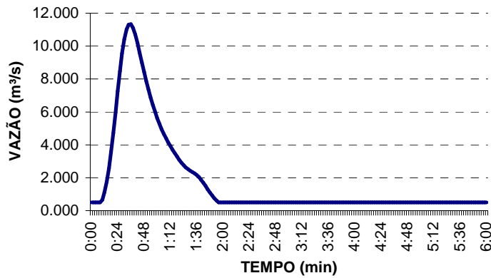
HIDROGRAMA 05
