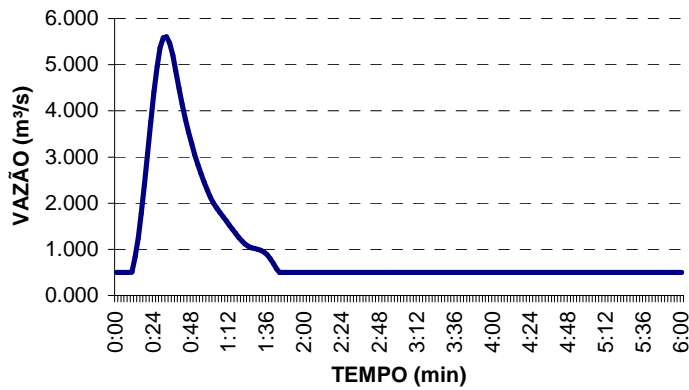
HIDROGRAMA 02
