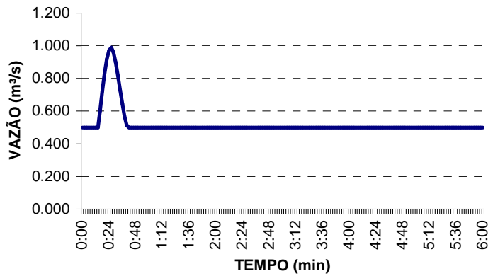
HIDROGRAMA 08
