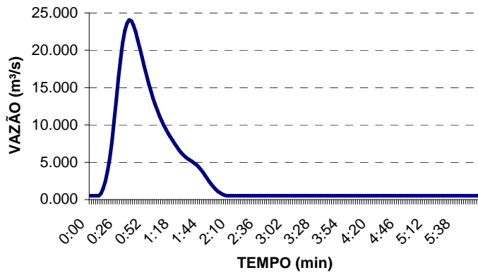
HIDROGRAMA 04
