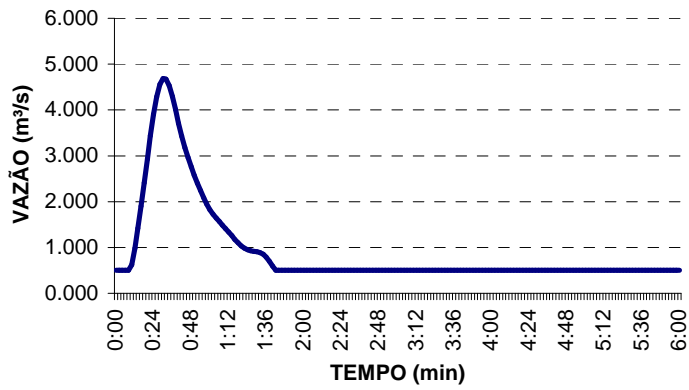
HIDROGRAMA 01
