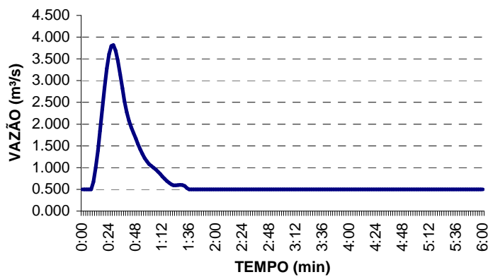
HIDROGRAMA 03
