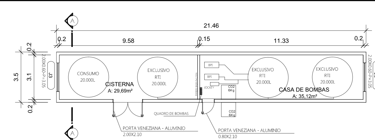
PLANTA BAIXA - CISTERNA / CASA DE BOMBAS
