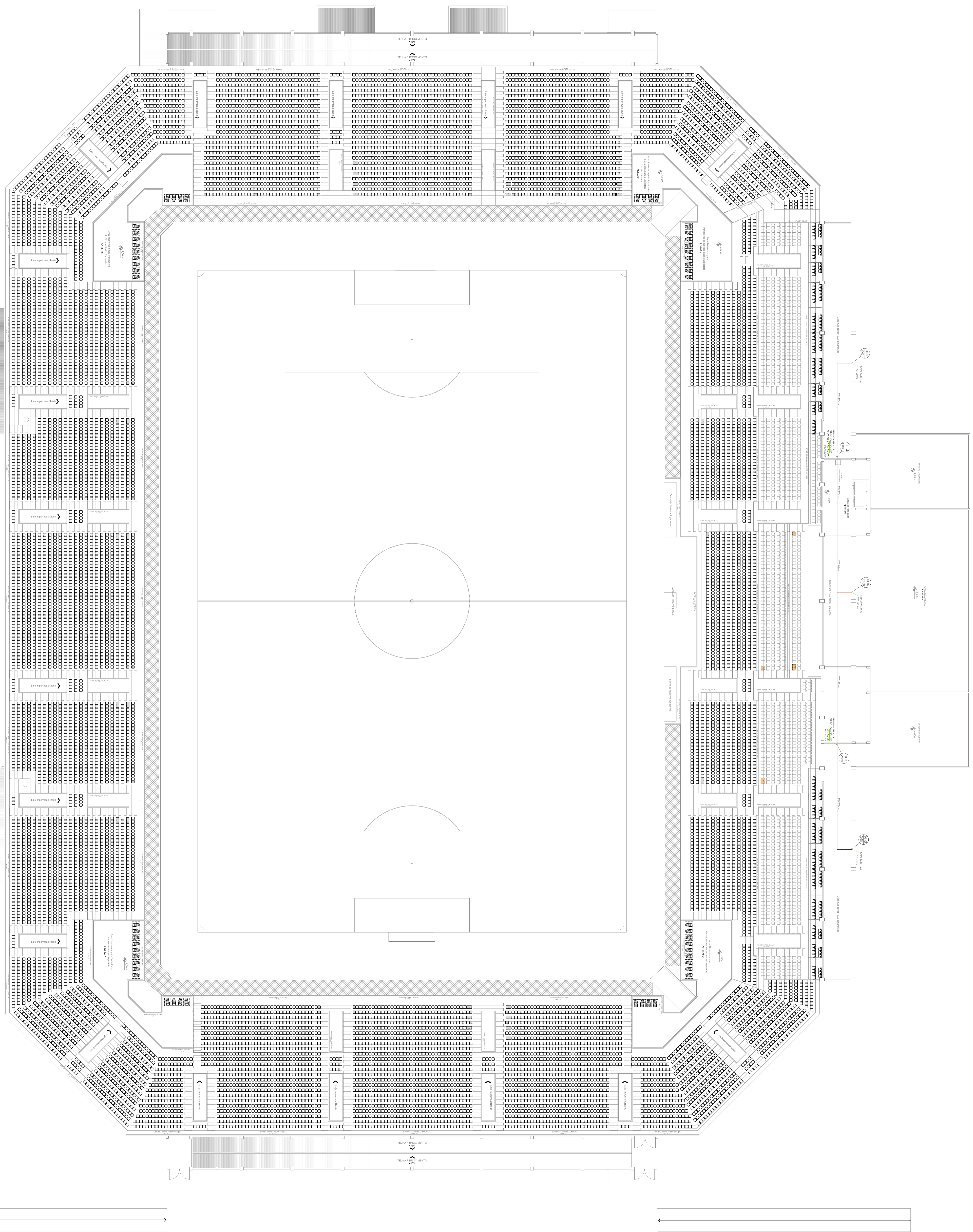
PLANTA BAIXA - NÍVEL 5 (19.50m Casa de Máquinas)
