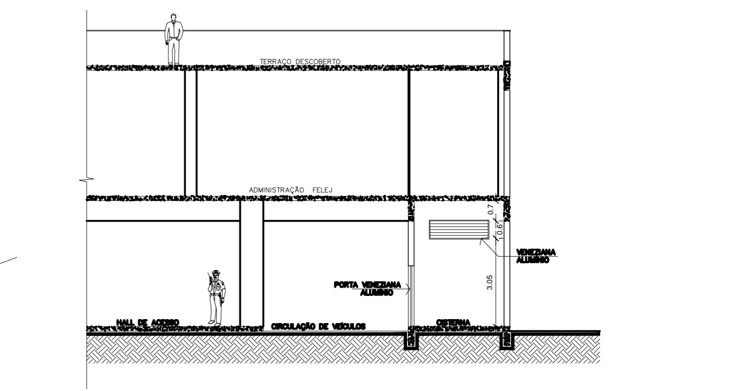
CORTE AA' - CISTERNA / CASA DE BOMBAS
