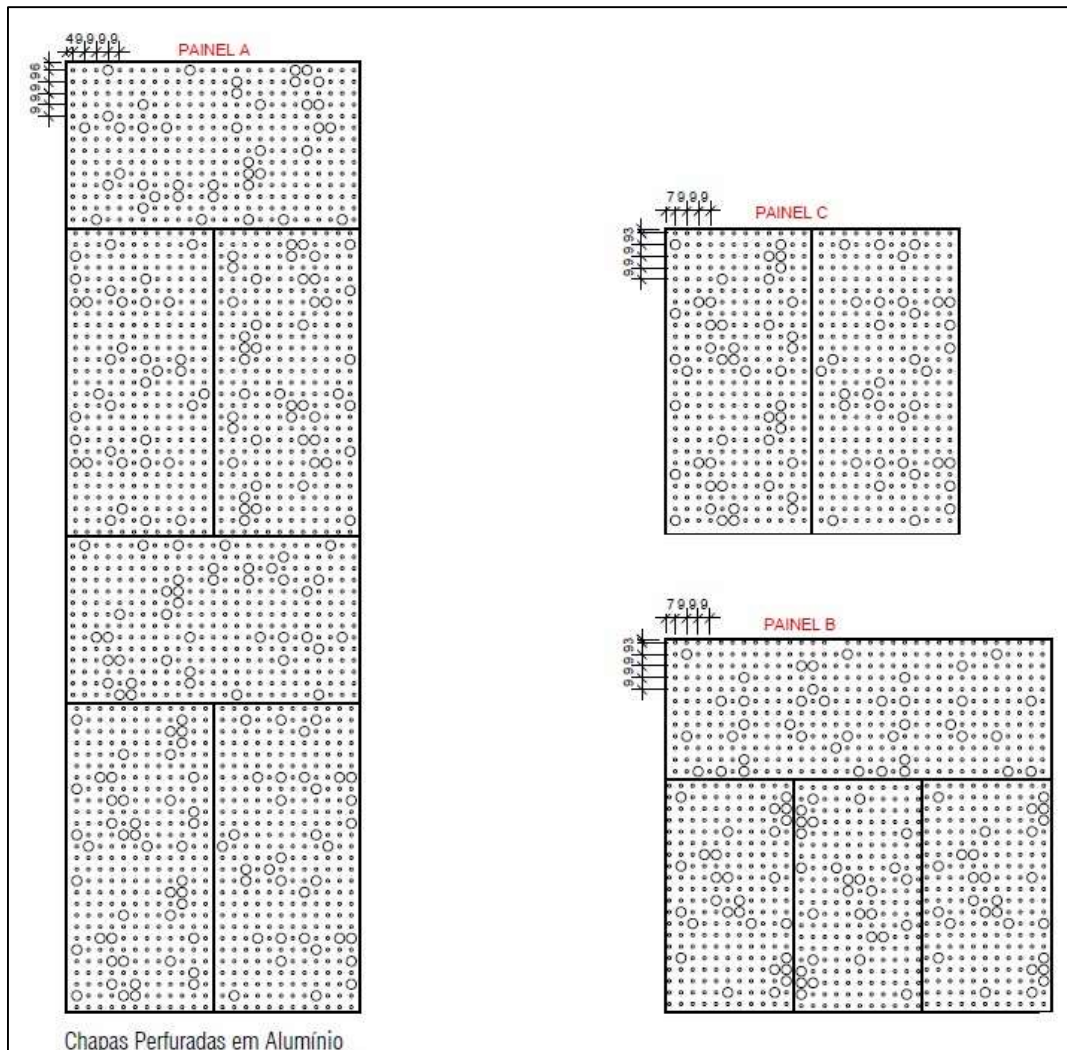
Figura 6 - Chapa perfurada p/ fechamento das Áreas Técnicas
