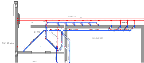
Detalhe - 6 E.S.PNE E.S.F. E.S.M.
