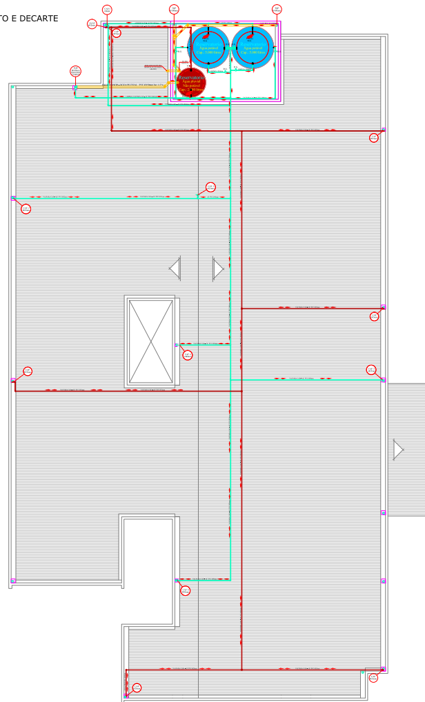
PLANTA DE COBERTURA ESCALA 1:75
