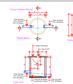
Corte A-A' Escala 1:10
