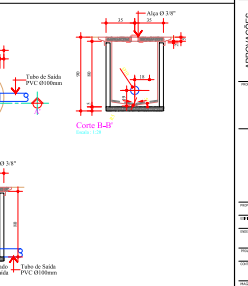
Corte B-B' Escala 1:10
