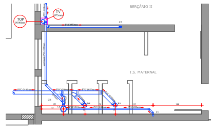
Detalhe - 7 E.S.F. E.S.M.
