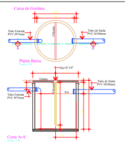
Corte A-A' Escala 1:10
