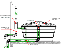
SISTEMA DE ARMAZENAMENTO E DECARTE Escala 1:25
