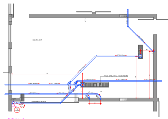
Detalhe - 2 E.S.F.
