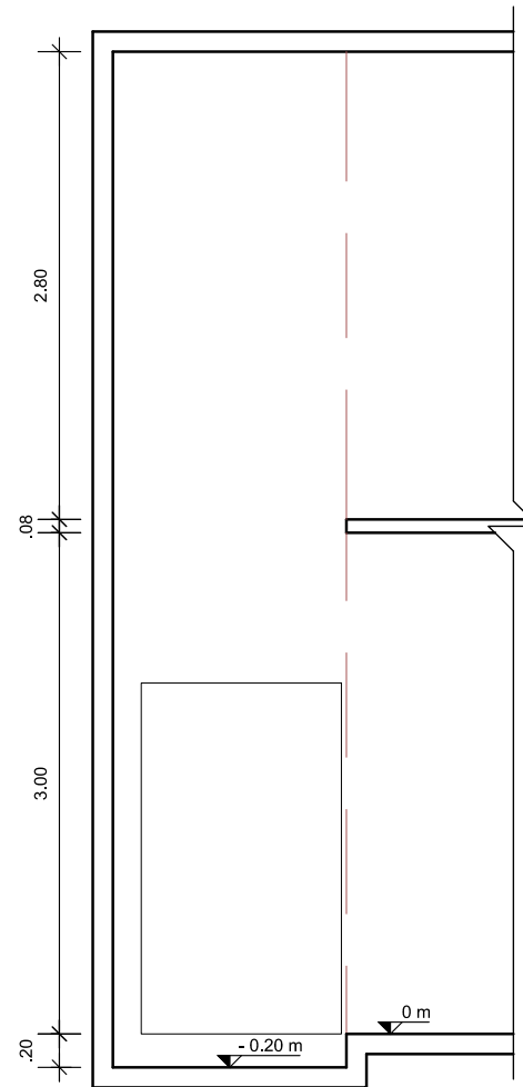
CORTE FOSSO ELEVADOR ESC. 1:50
