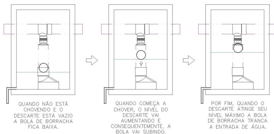
Figura 01: Detalhe do dispositivo que impede o refluxo.
