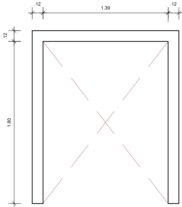
PLANTA BAIXA FOSSE ELEVADOR
