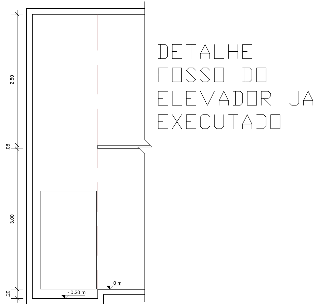
CORTE FOSSE ELEVADOR ESC. 1:50
