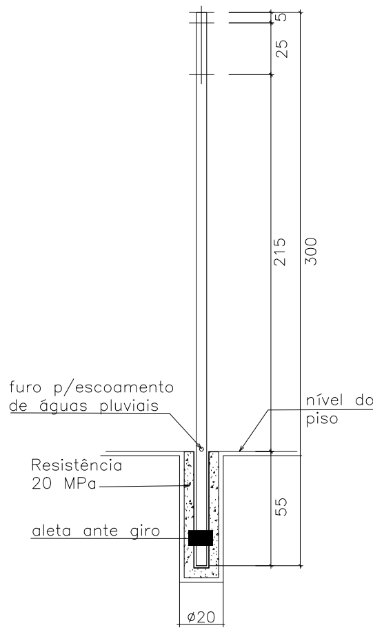
DETALHE DO POSTE
