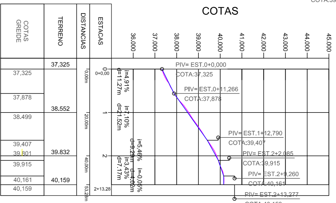
PERFIL LONGITUDINAL Escala HORIZONTAL 1:1.000 Escala VERTICAL 1:100
