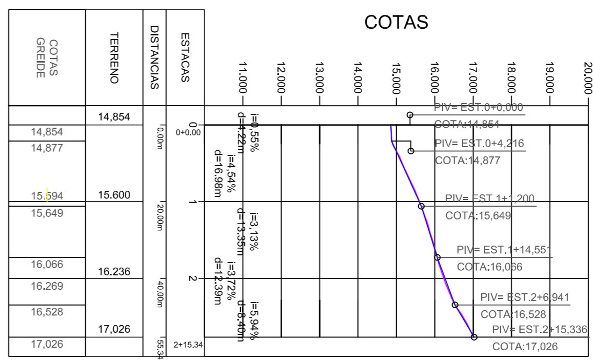
PERFIL LONGITUDINAL Escala HORIZONTAL 1:1.000 Escala VERTICAL 1:100
