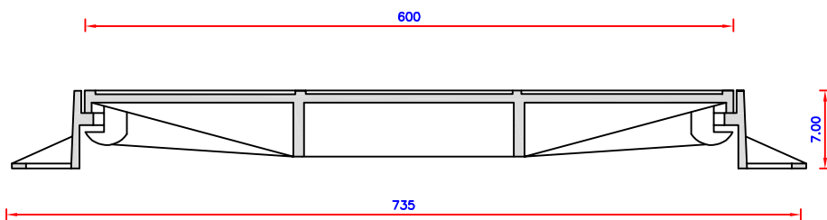
CORTE AA S/ESCALA
