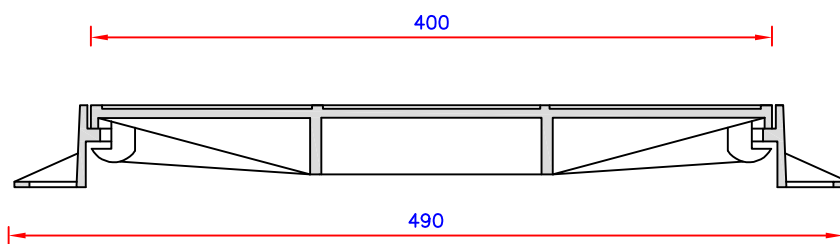
CORTE AA S/ESCALA
