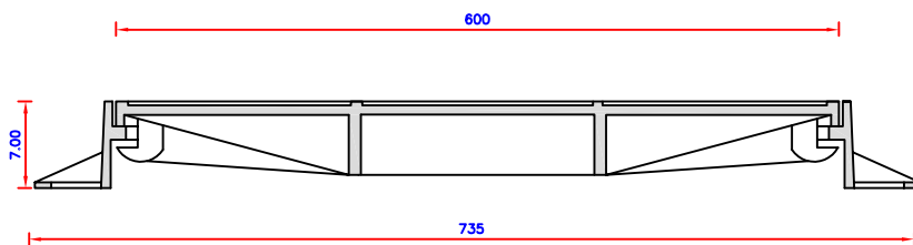
CORTE AA ESCALA
