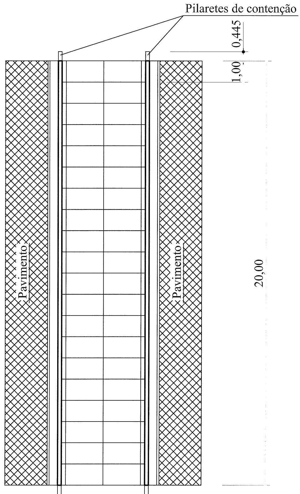
Planta Baixa - Trecho 1
