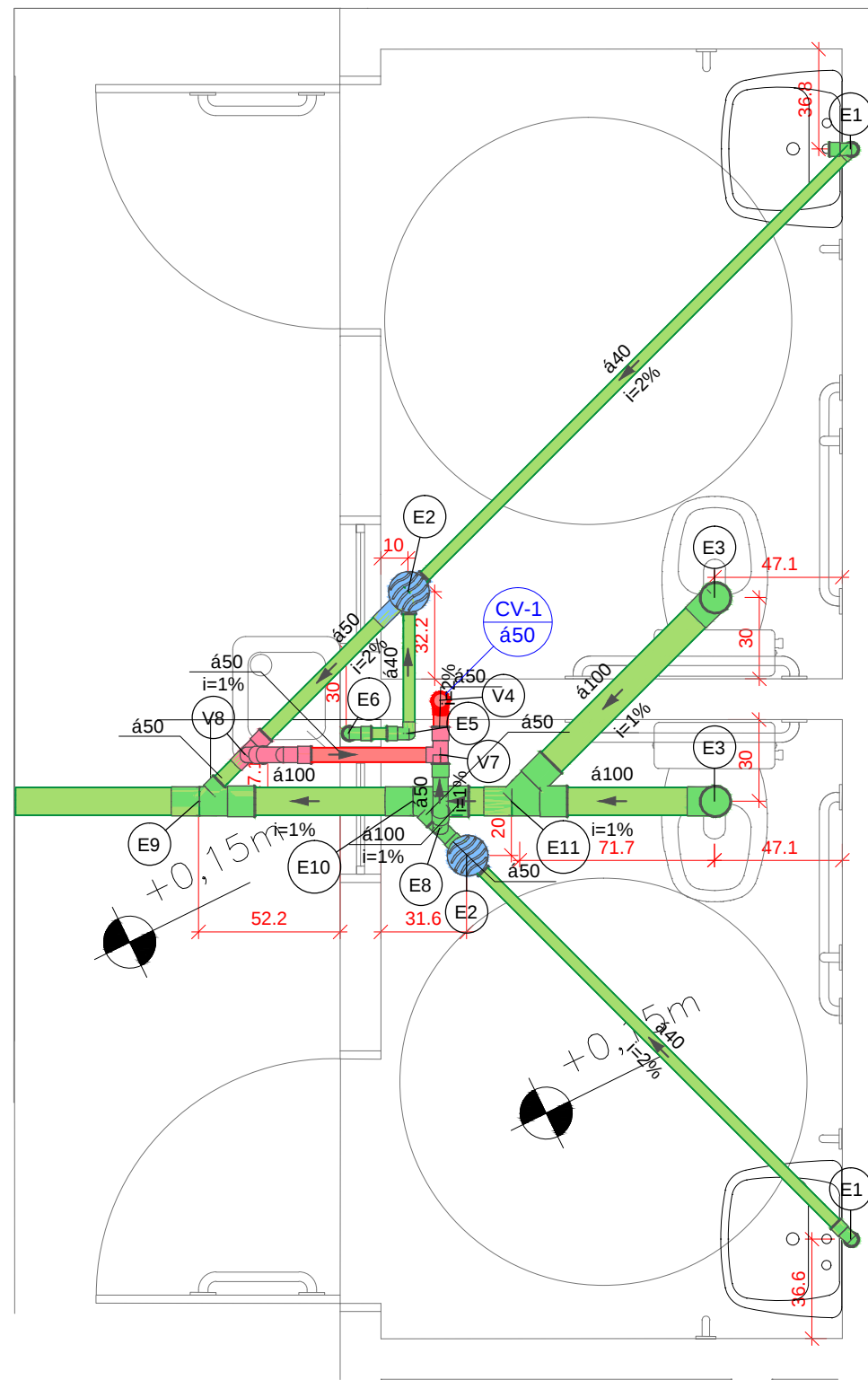
Detalhe Sanit' rio2 Escala 1:25
