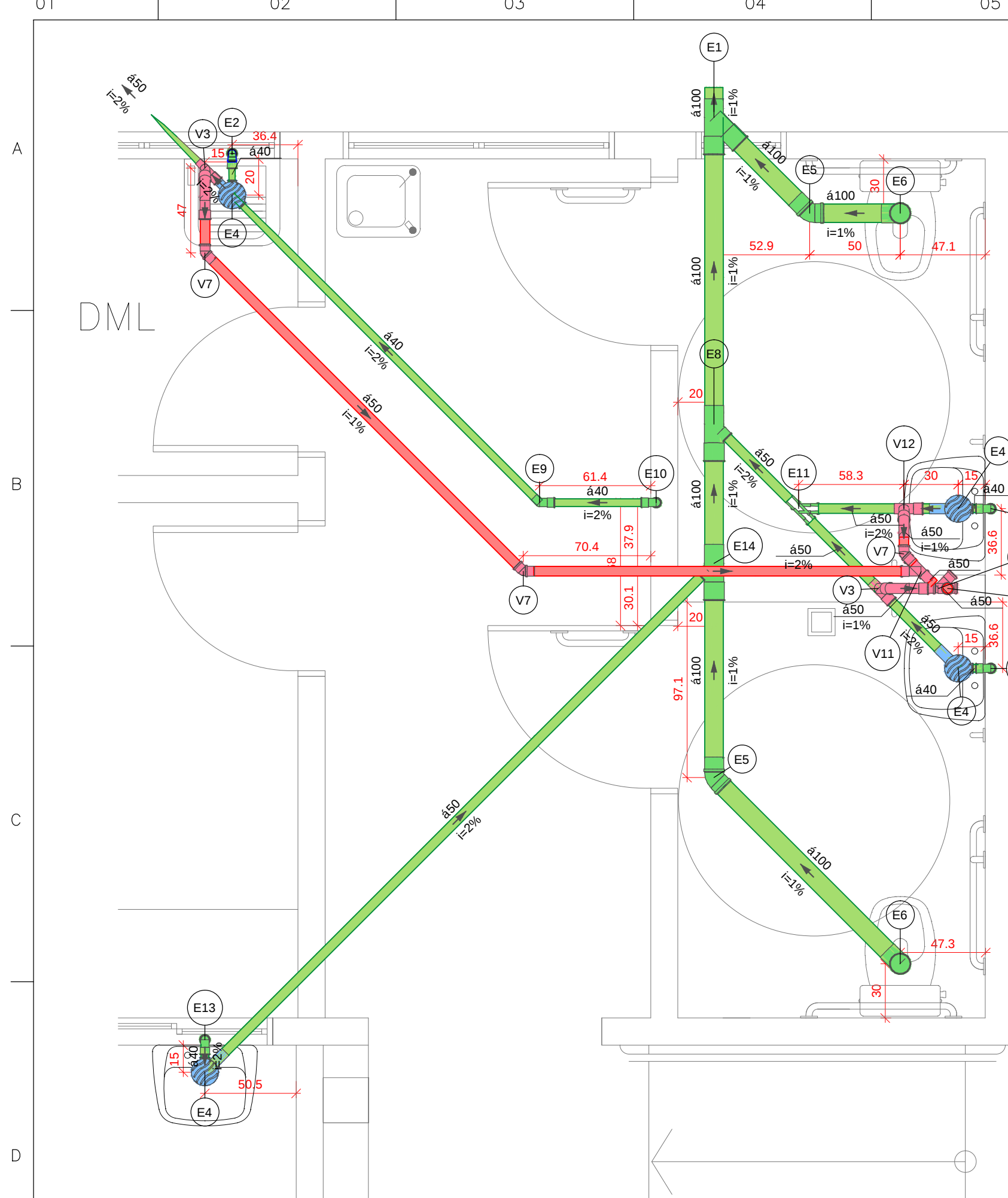
Detalhe Sanit' rio1 Escala 1:25
