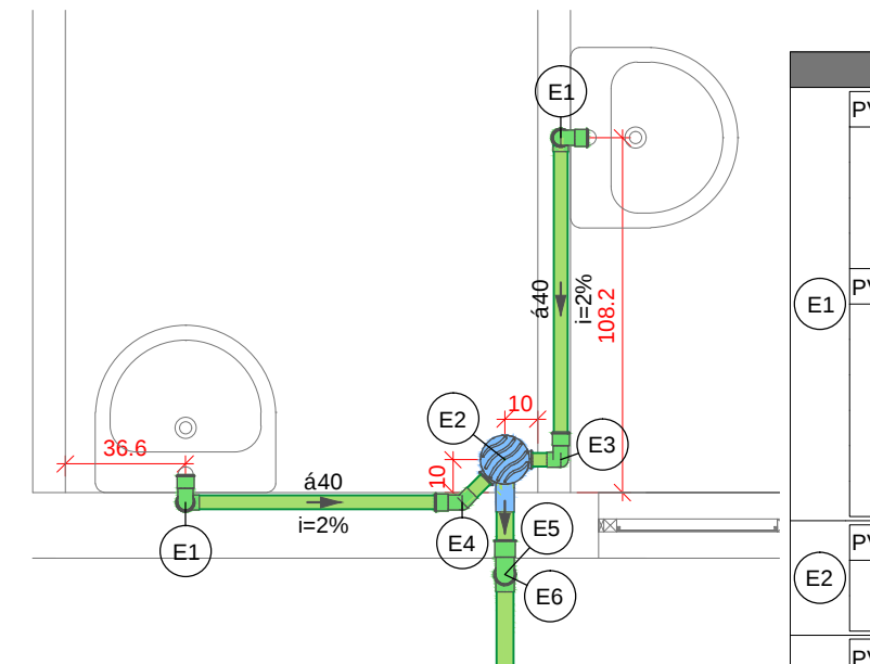
Detalhe Sanit' rio9 Escala 1:25
