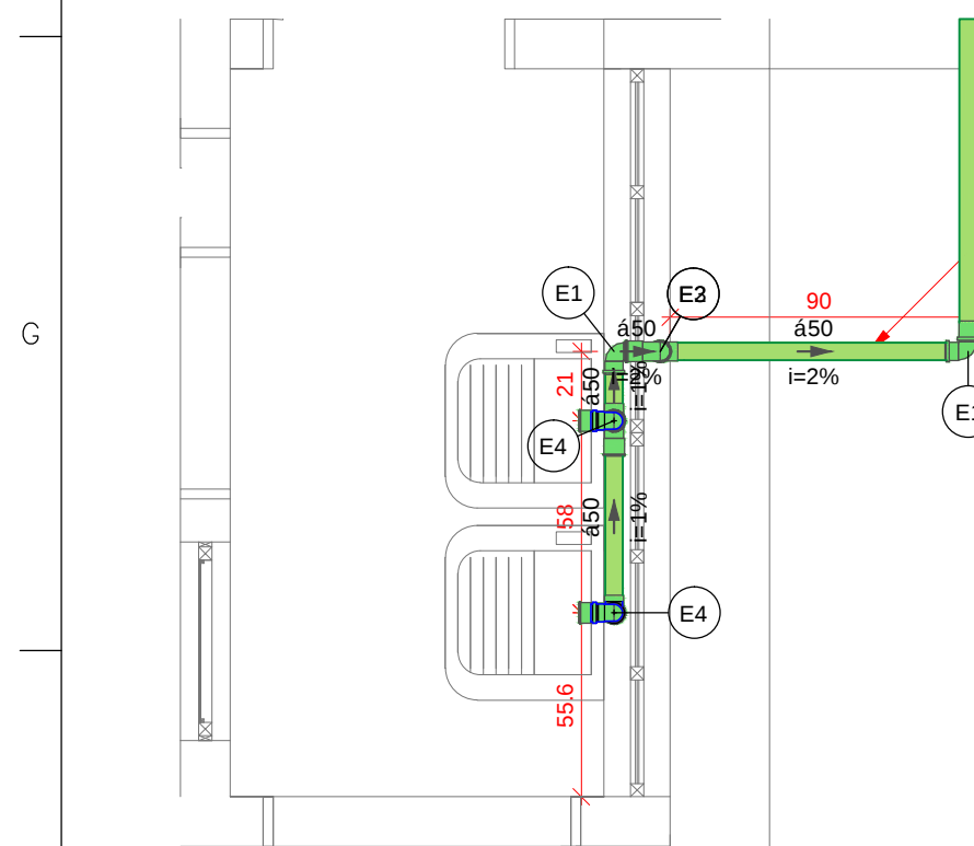
Detalhe Sanit' rio6 Escala 1:25
