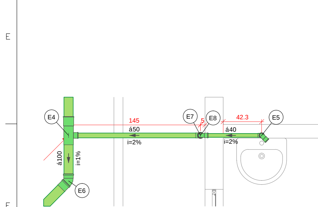
Detalhe Sanit' rio5 Escala 1:25
