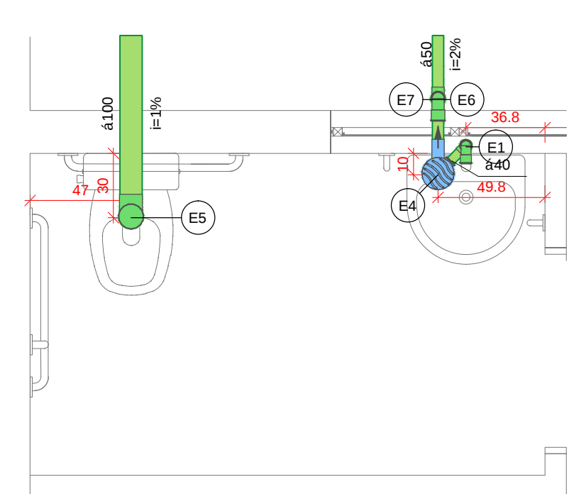
Detalhe Sanit' rio7 Escala 1:25
