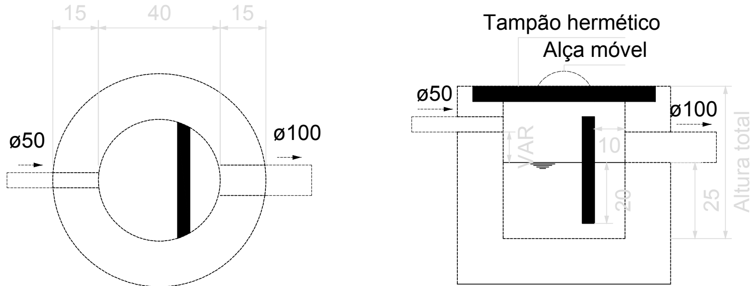
PLANTA BAIXA - CAIXA DE GORDURA Escala 1:25
