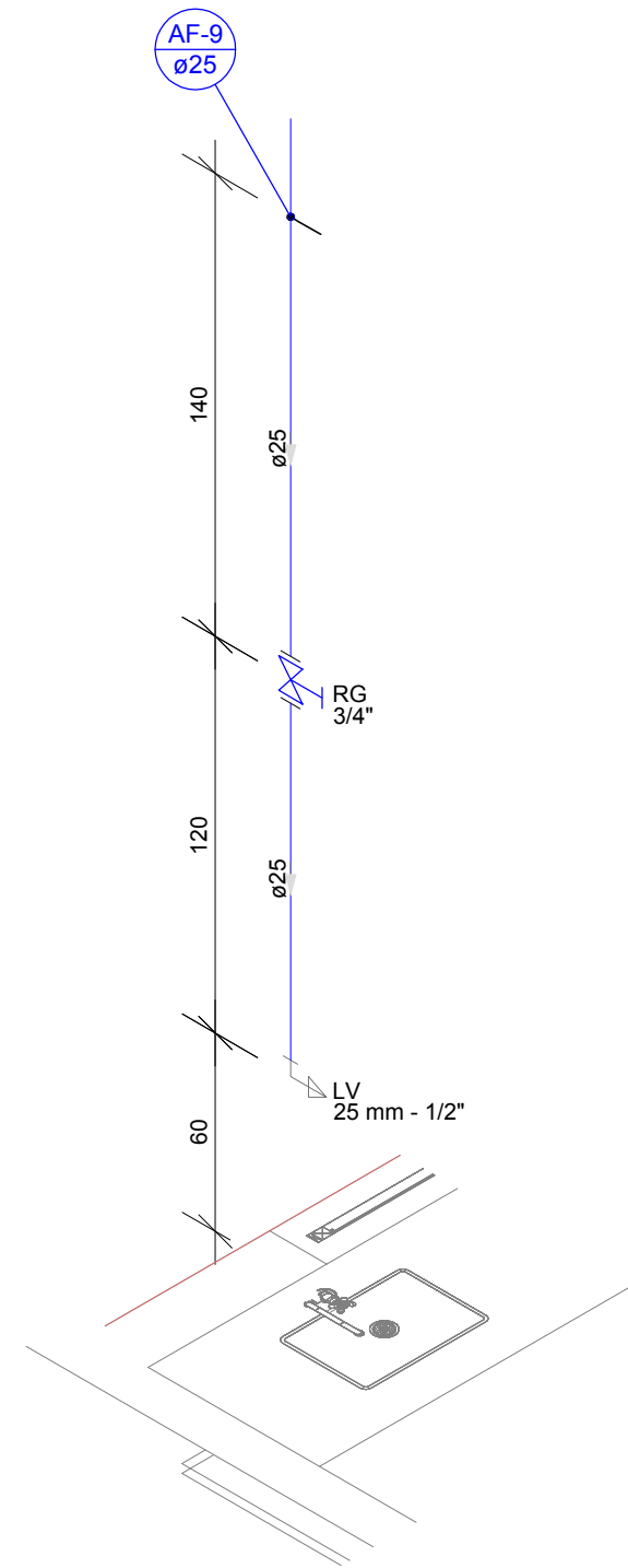
DETALHE H6 Escala 1:25
