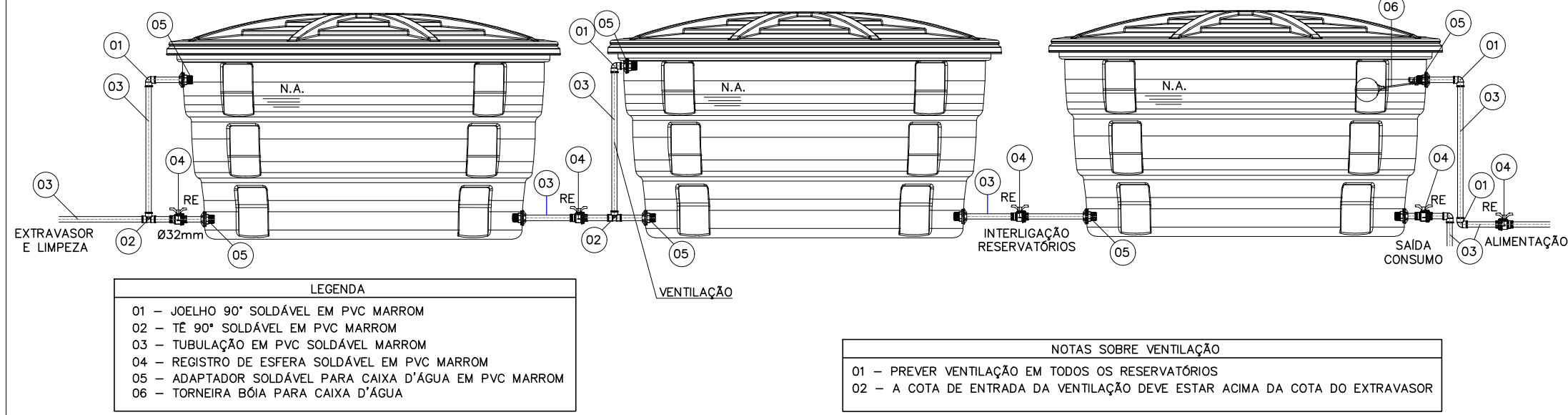
DETALHE RESERVATÓRIOS Escala 1:25
