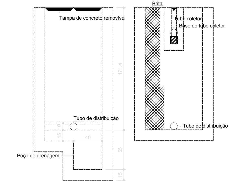
CORTE 2 - FILTRO ANAERÓBIO Escala 1:25
