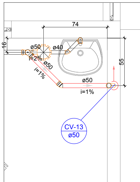
DETALHE S11 Escala 1:25
