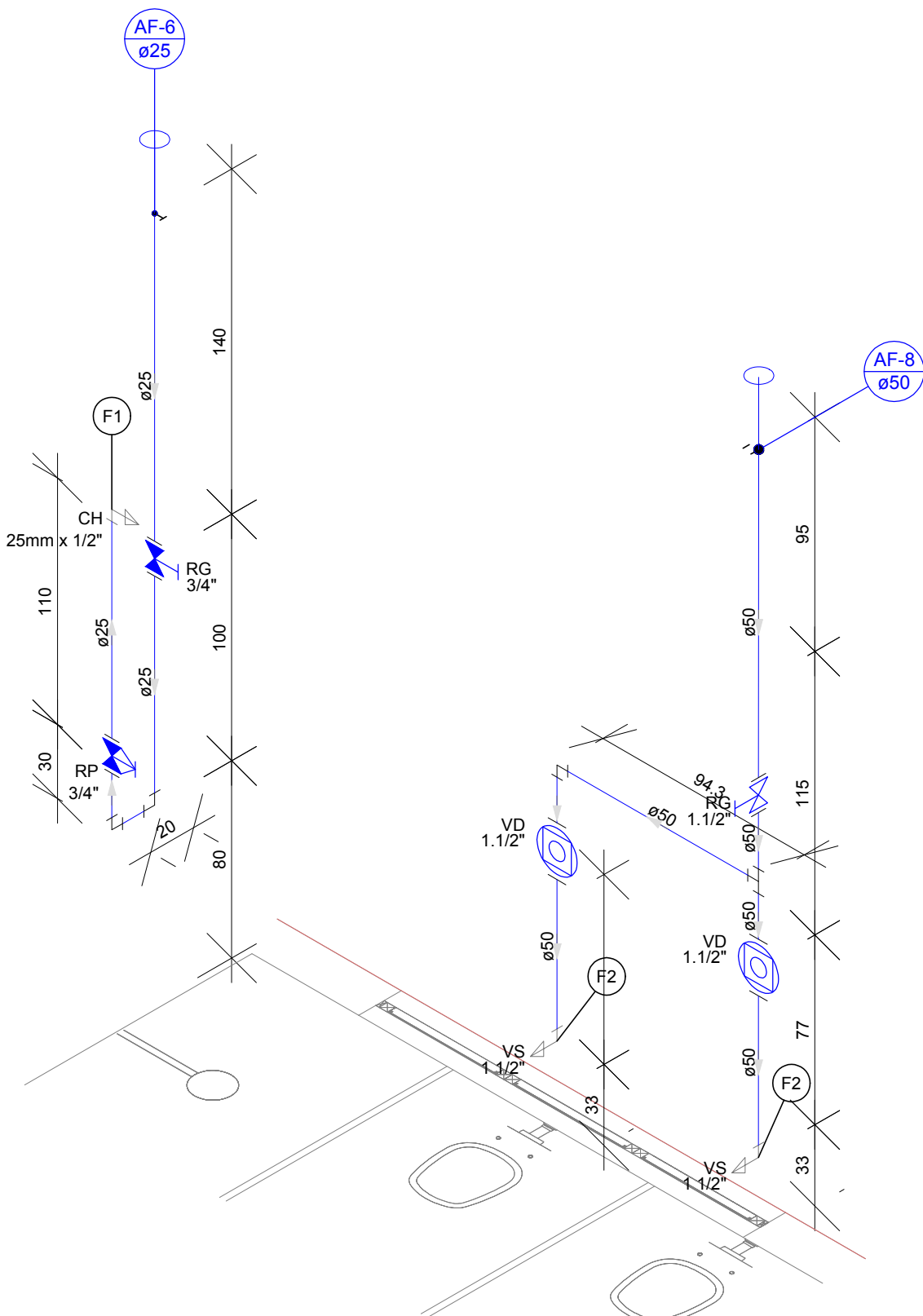
DETALHE H4 Escala 1:25
