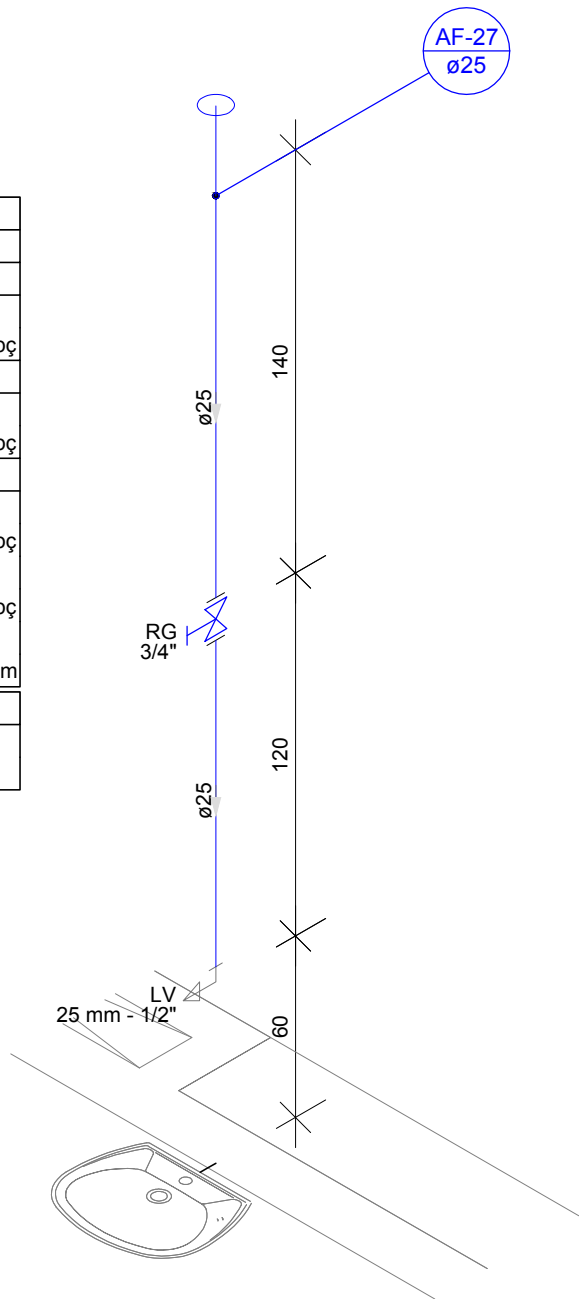
DETALHE H18 Escala 1:25
