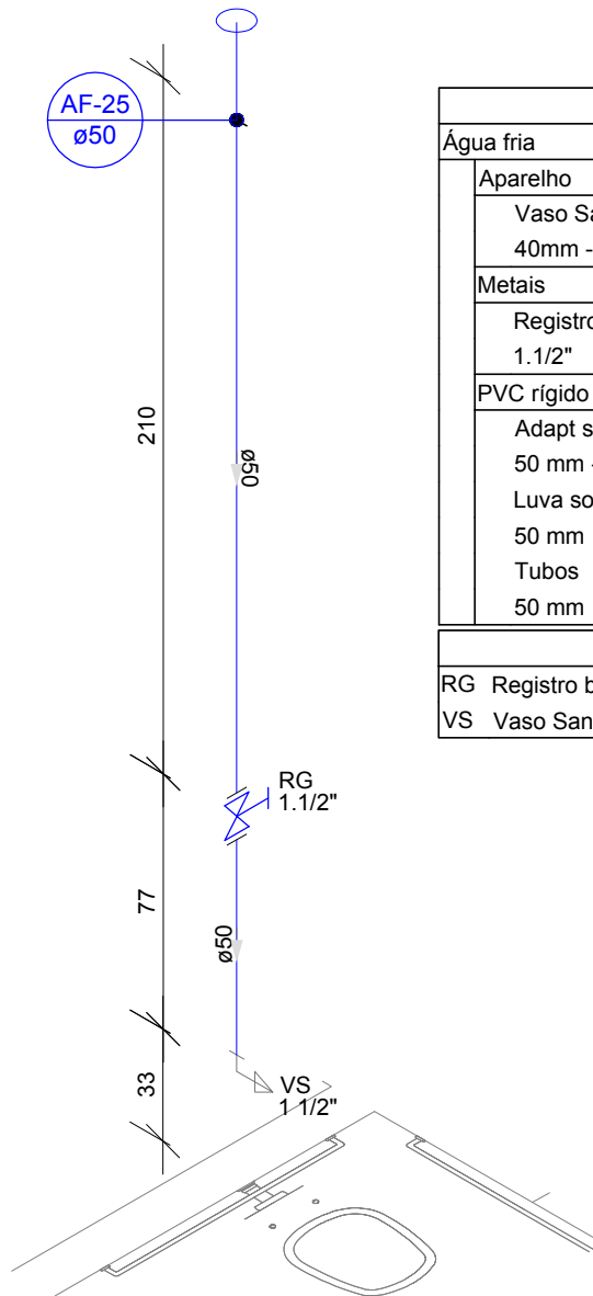
DETALHE H17 Escala 1:25
