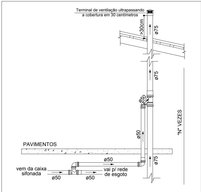
ESQUEMA VERTICAL - VENTILAÇÃO Escala 1:25
