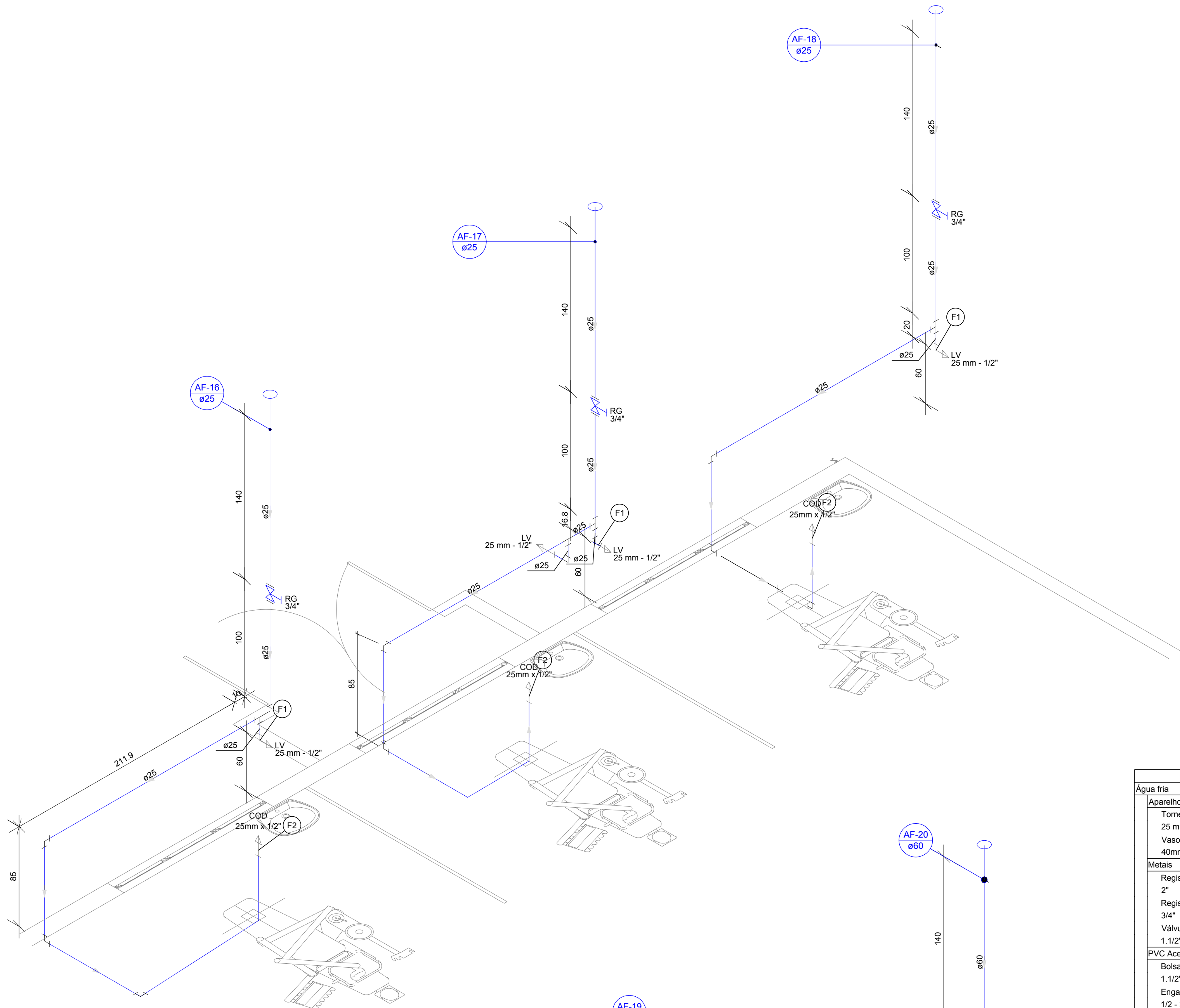
DETALHE H14 Escala 1:25
