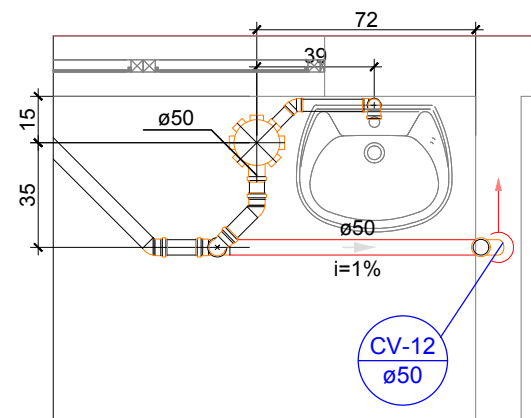
DETALHE S8 Escala 1:25
