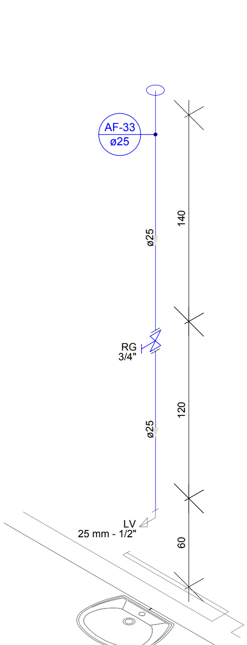
DETALHE H25 Escala 1:25
