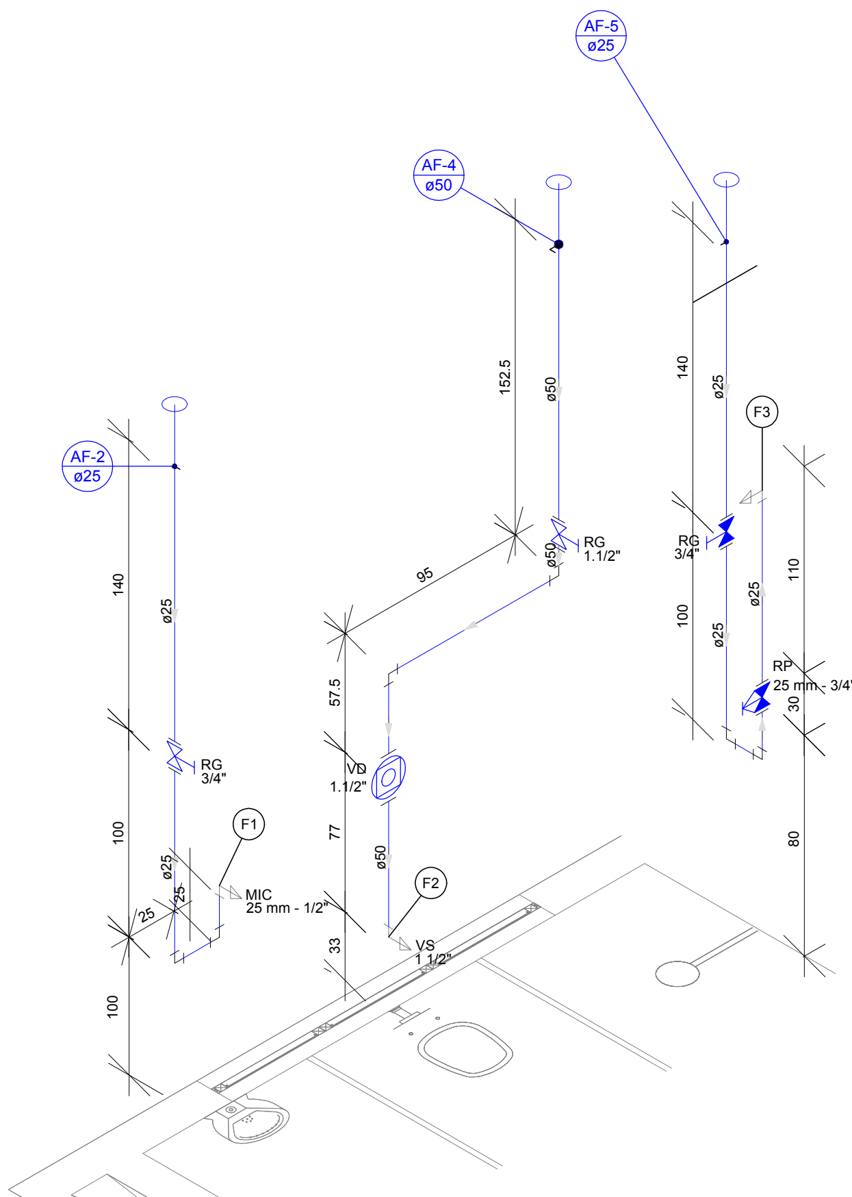
DETALHE H2 Escala 1:25
