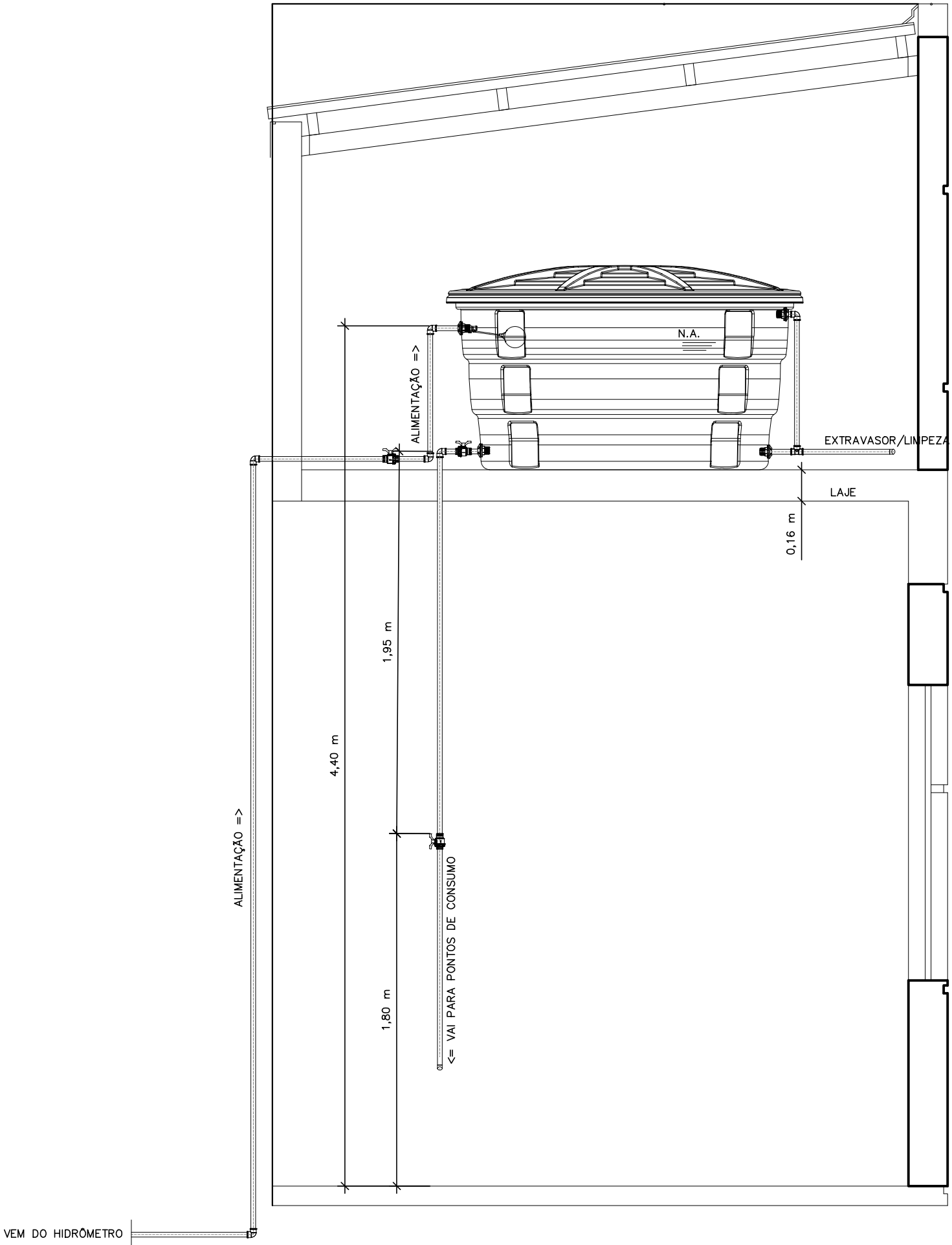
ESQUEMA VERTICAL DO RESERVATÓRIO Escala 1:25
