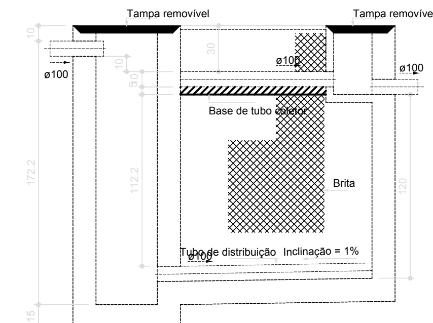
CORTE 1 - FILTRO ANAERÓBIO Escala 1:25
