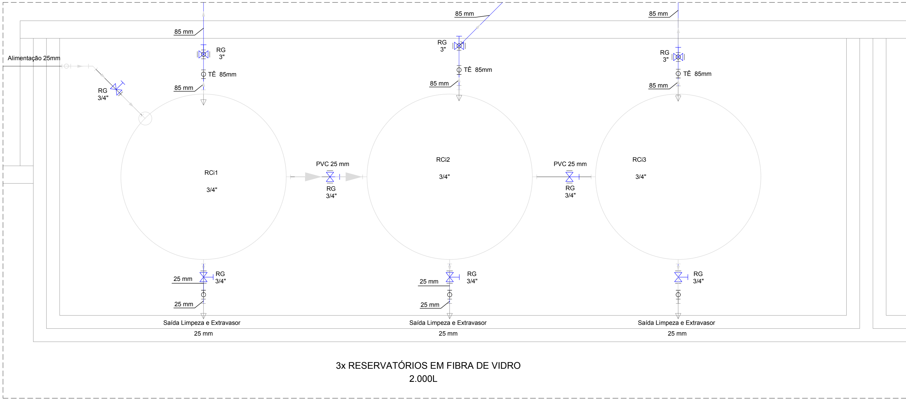
DETALHE H32 Escala 1:25
