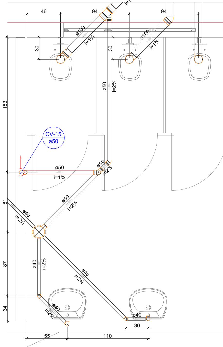
DETALHE S12 Escala 1:25
