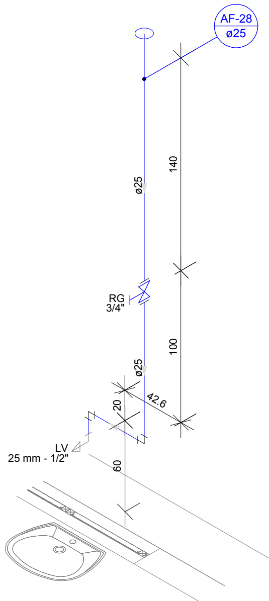
DETALHE H19 Escala 1:25
