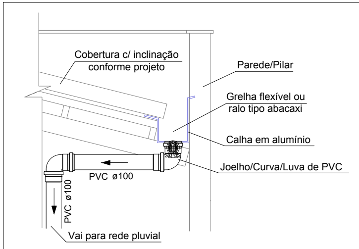
DETALHE INSTALAÇÃO DA CALHA Escala 1:25
