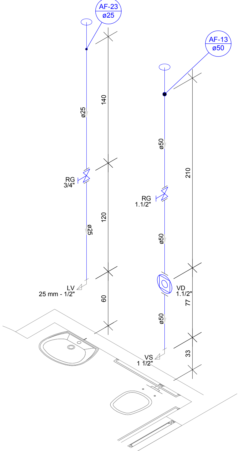
DETALHE H9 Escala 1:25
