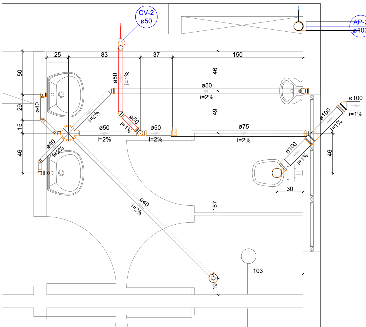
DETALHE S2 Escala 1:25
