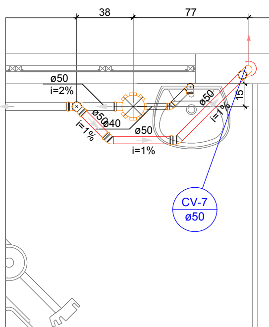
DETALHE S9 Escala 1:25
