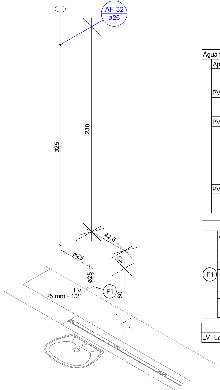
DETALHE H23 Escala 1:25
