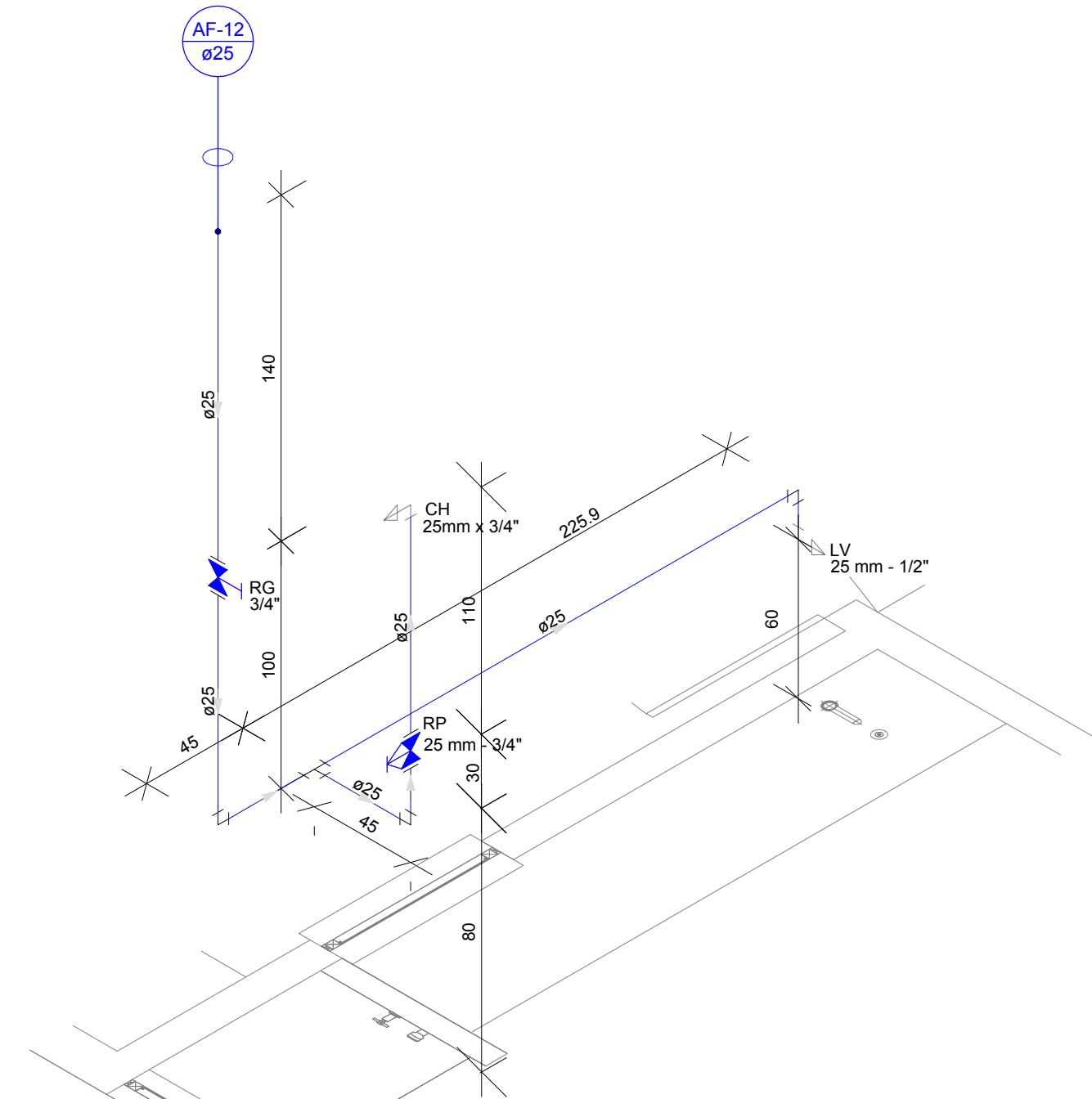
DETALHE H11 Escala 1:25
