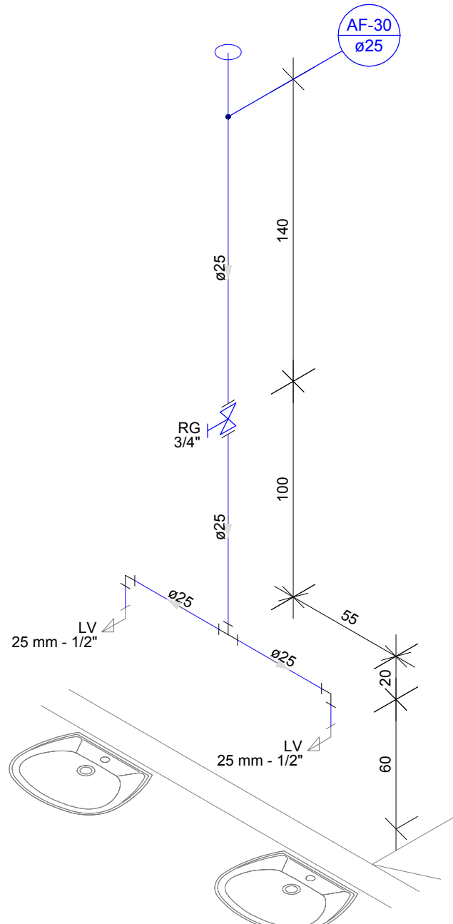
DETALHE H18 Escala 1:25
