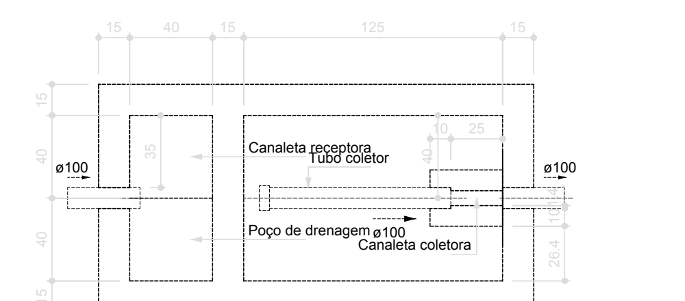
PLANTA BAIXA - FILTRO ANAERÓBIO Escala 1:25
