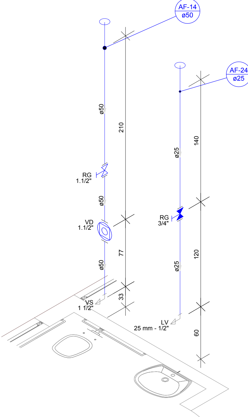
DETALHE H10 Escala 1:25
