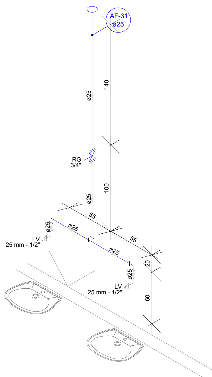
DETALHE H22 Escala 1:25
