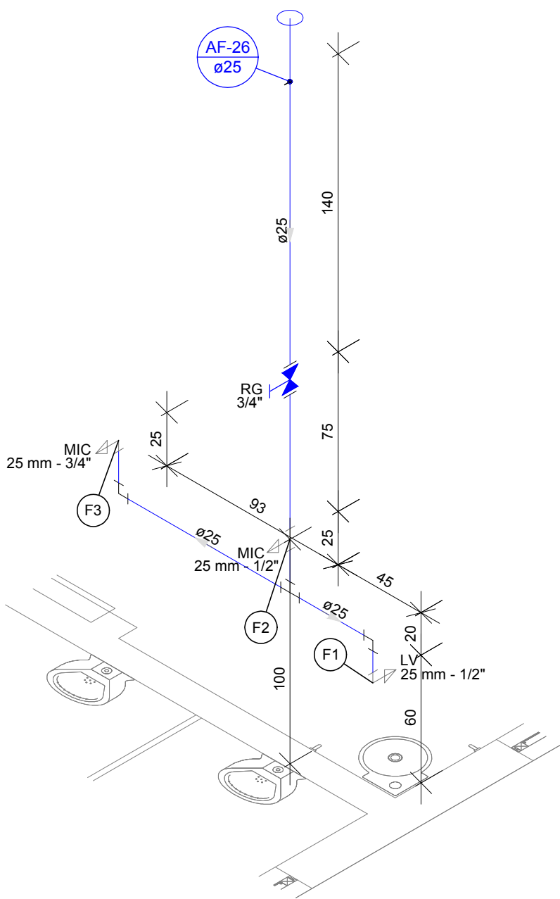
DETALHE H16 Escala 1:25
