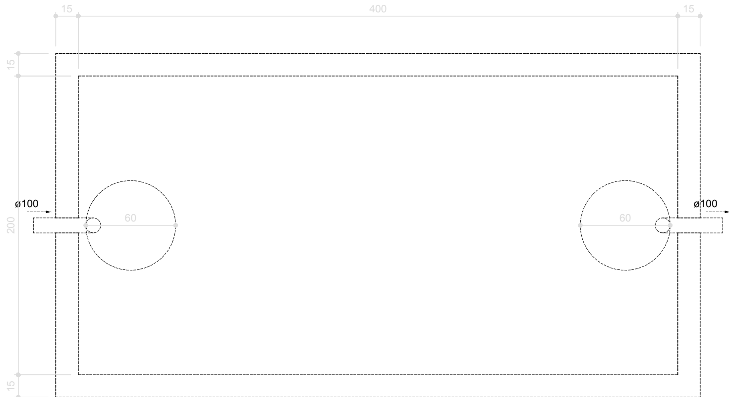
CORTE 1 - TANQUE ANAERÓBIO Escala 1:25
