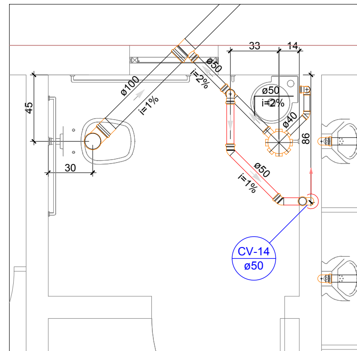
DETALHE S13 Escala 1:25
