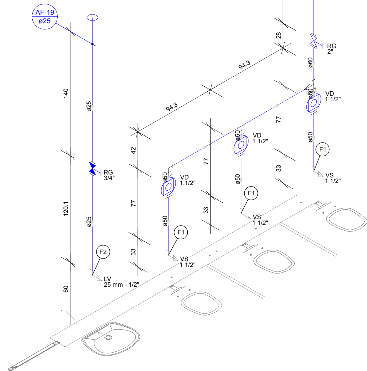
DETALHE H15 Escala 1:25
