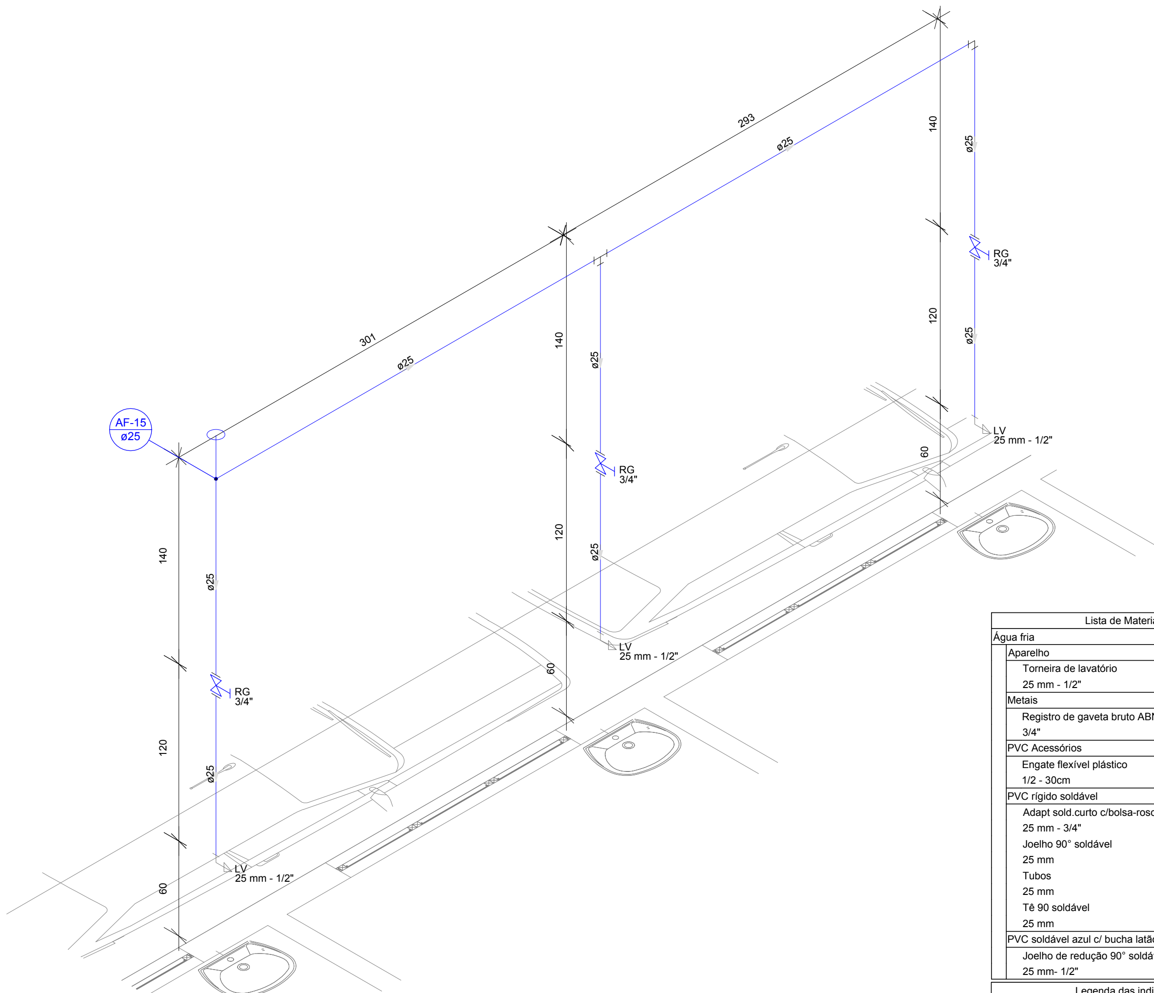
DETALHE H11 Escala 1:25
