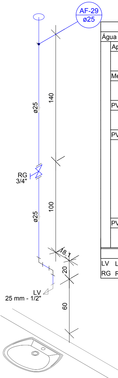
DETALHE H20 Escala 1:25
