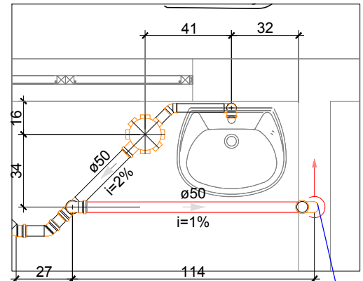
DETALHE S7 Escala 1:25
