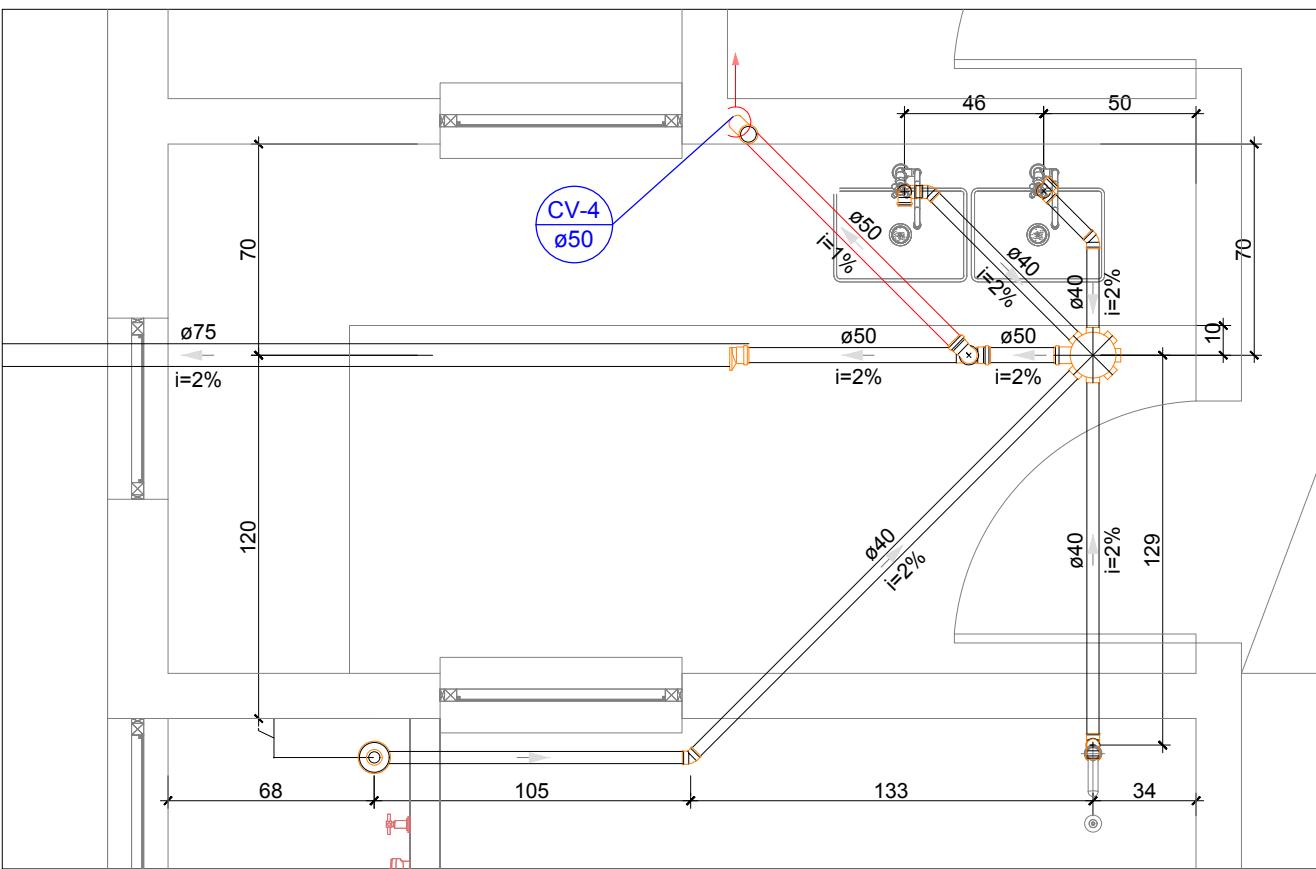
DETALHE S4 Escala 1:25
