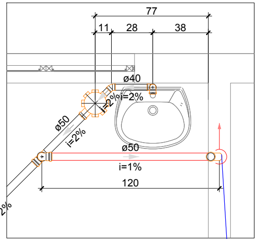
DETALHE S6 Escala 1:25
