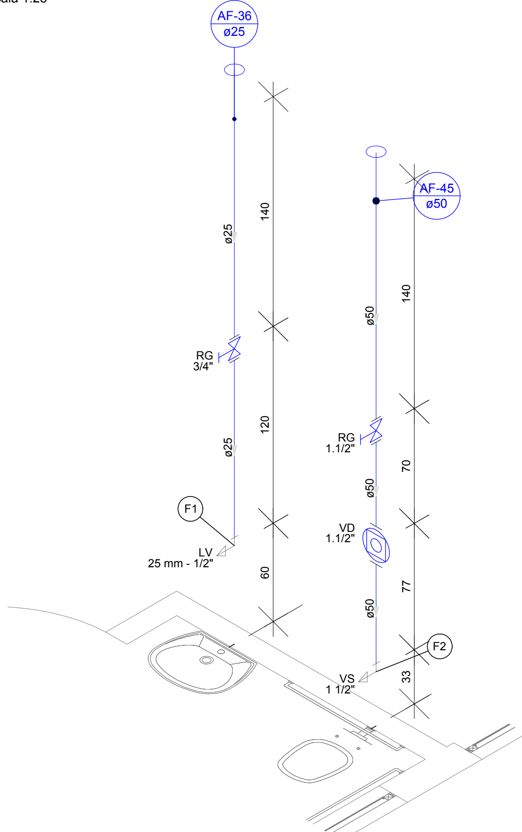
DETALHE H23 Escala 1:25
