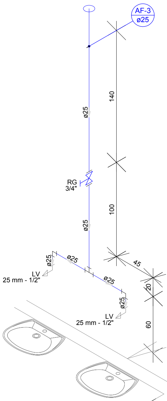
DETALHE H3 Escala 1:25
