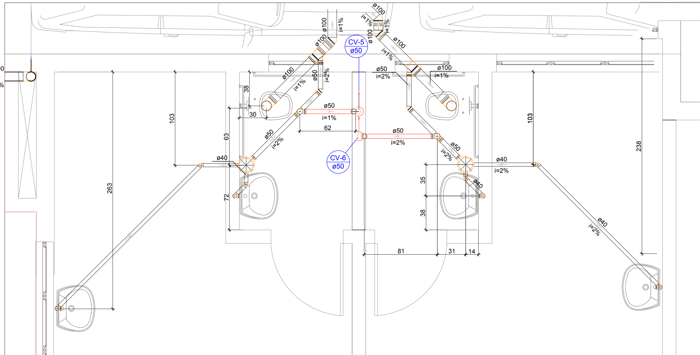
DETALHE S5 Escala 1:25
