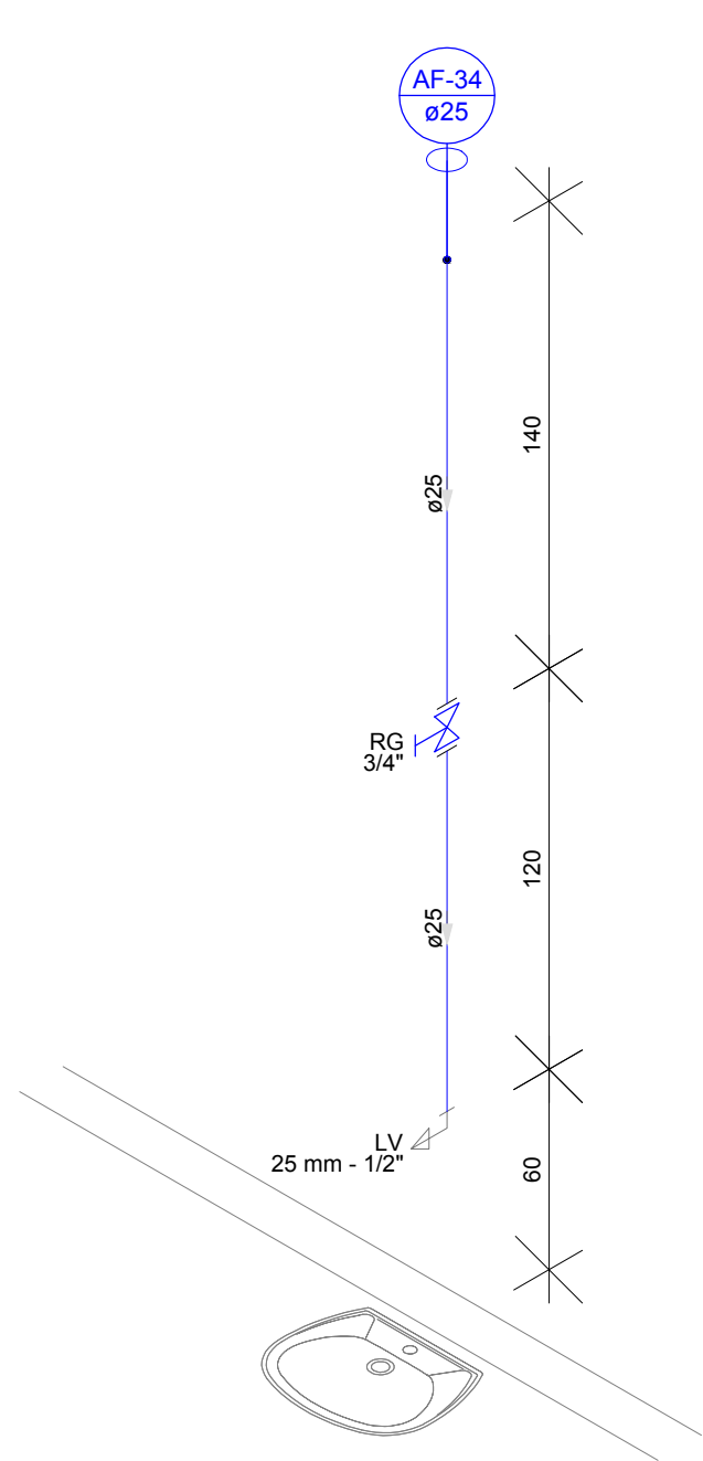
DETALHE H24 Escala 1:25
