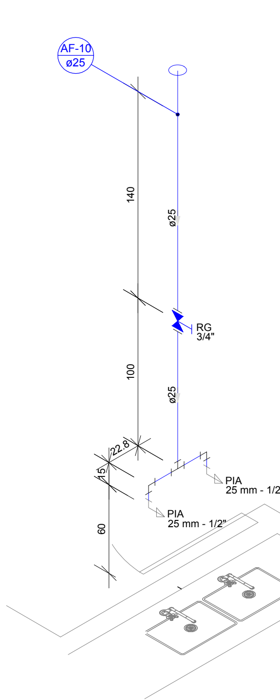
DETALHE H7 Escala 1:25
