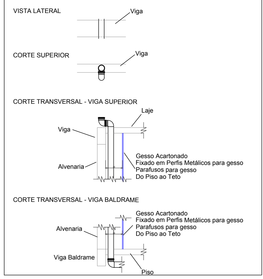
DETALHE DA MOCHETA S/ escala
