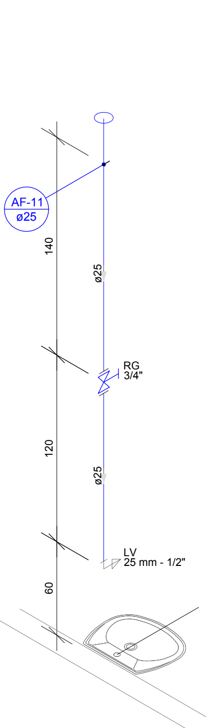
DETALHE H8 Escala 1:25
