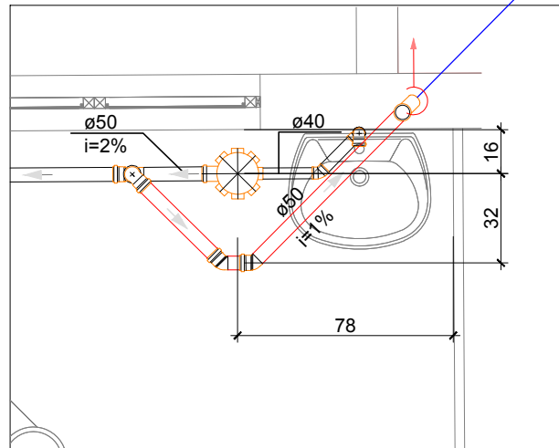
DETALHE S10 Escala 1:25
