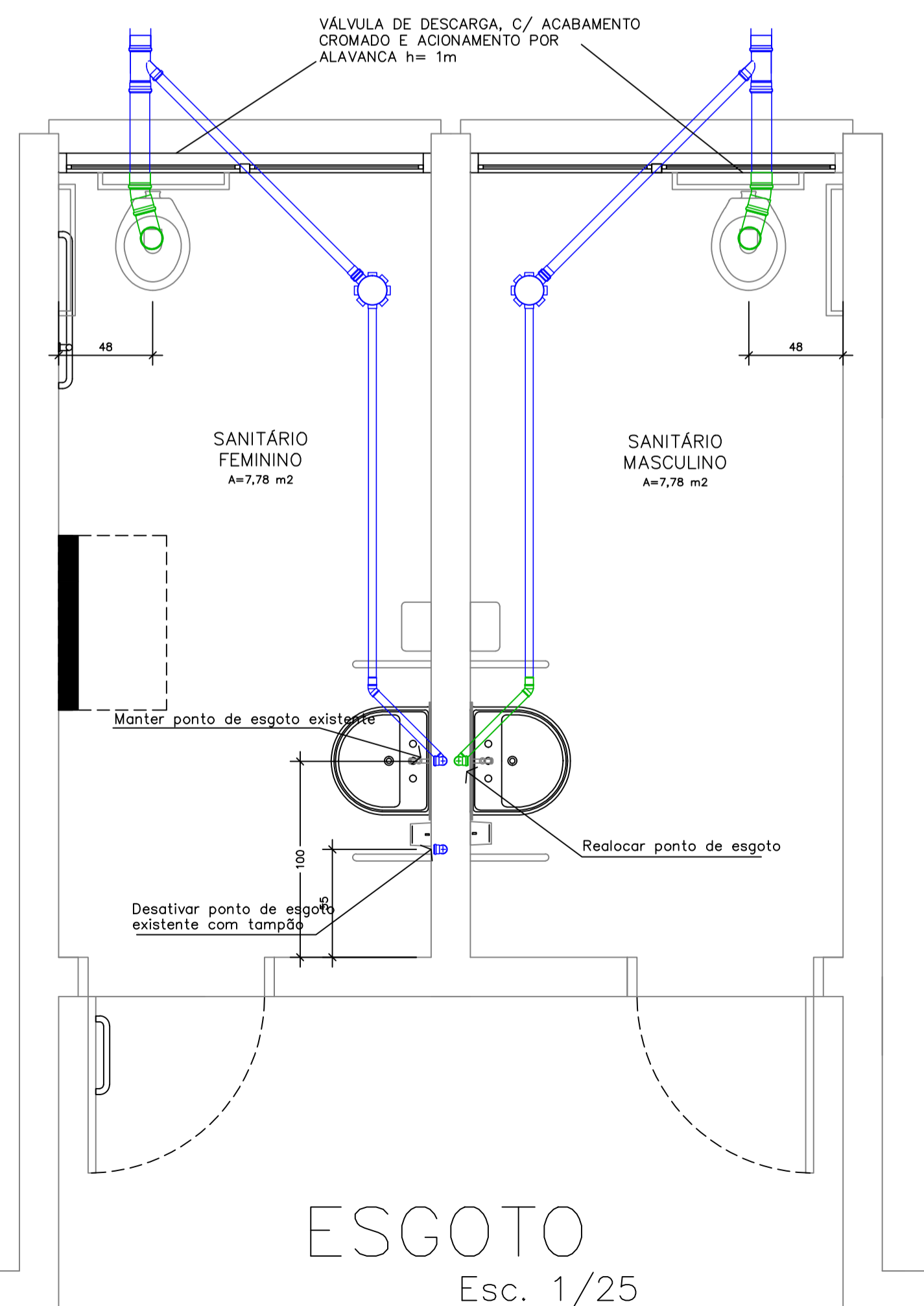
ISOMÉTRICO Escala 1/25
