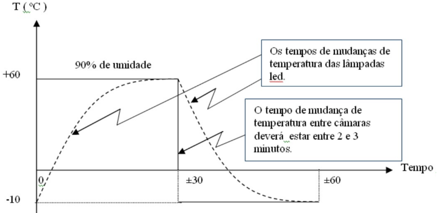
Figura 1: Ciclo de temperatura.
