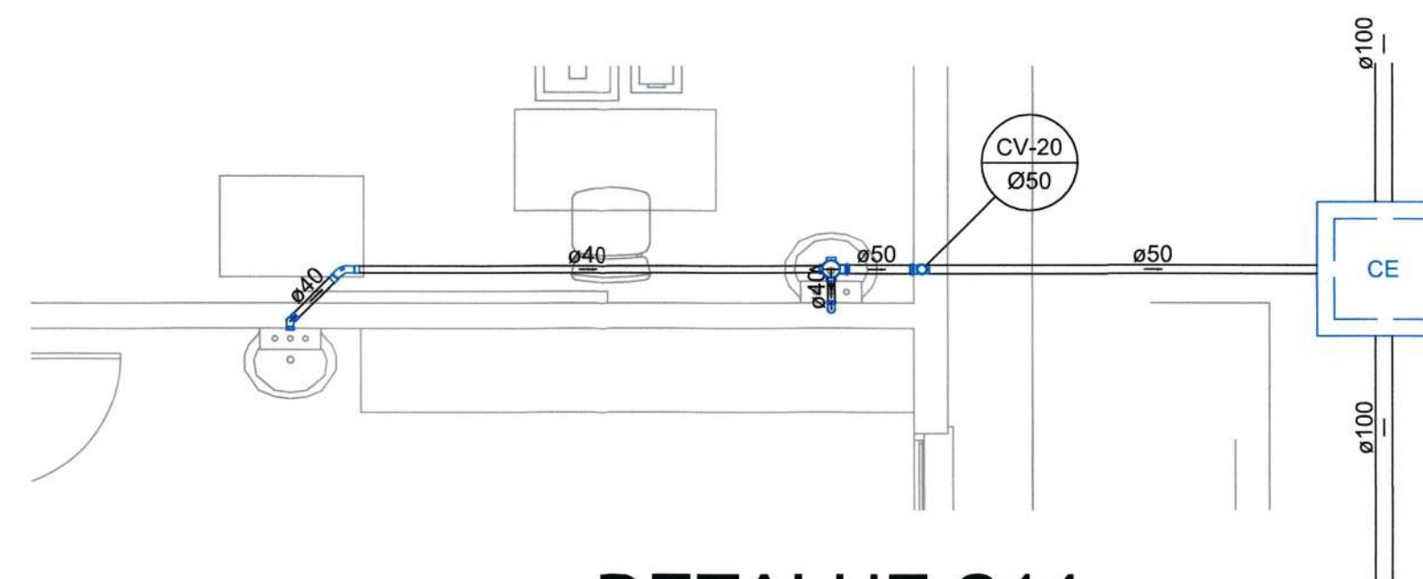
DETALHE S14
