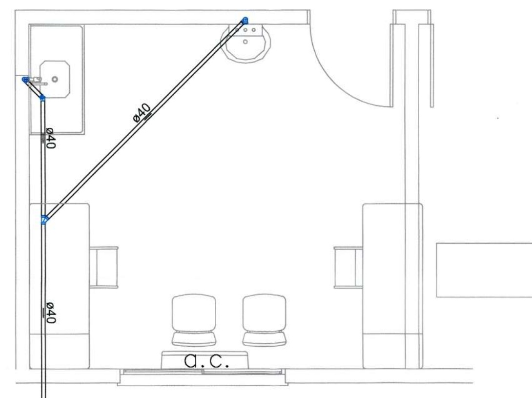
DETALHE S10
