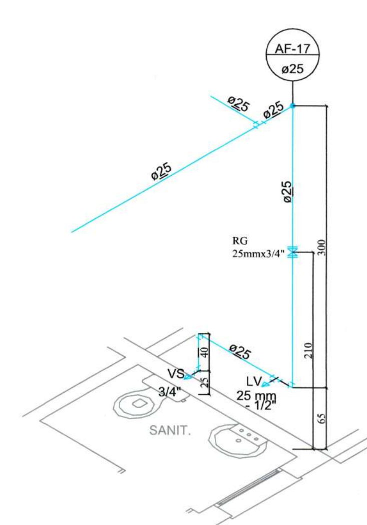
DETALHE H23
