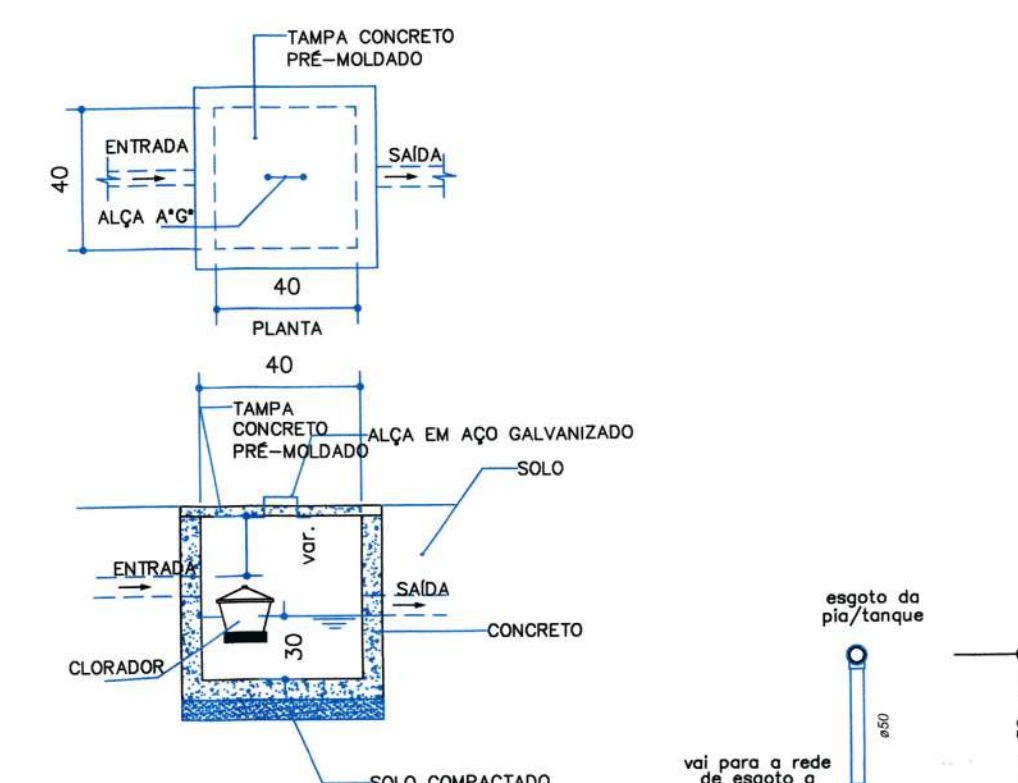
DETALHE CLORADOR ESC. 1/25
