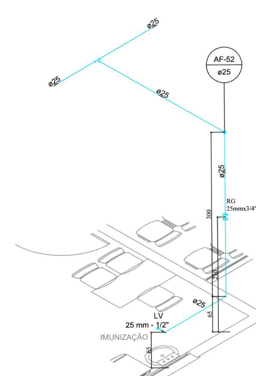
DETALHE H12
