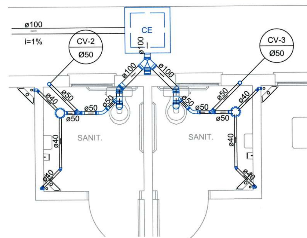
DETALHE S1
