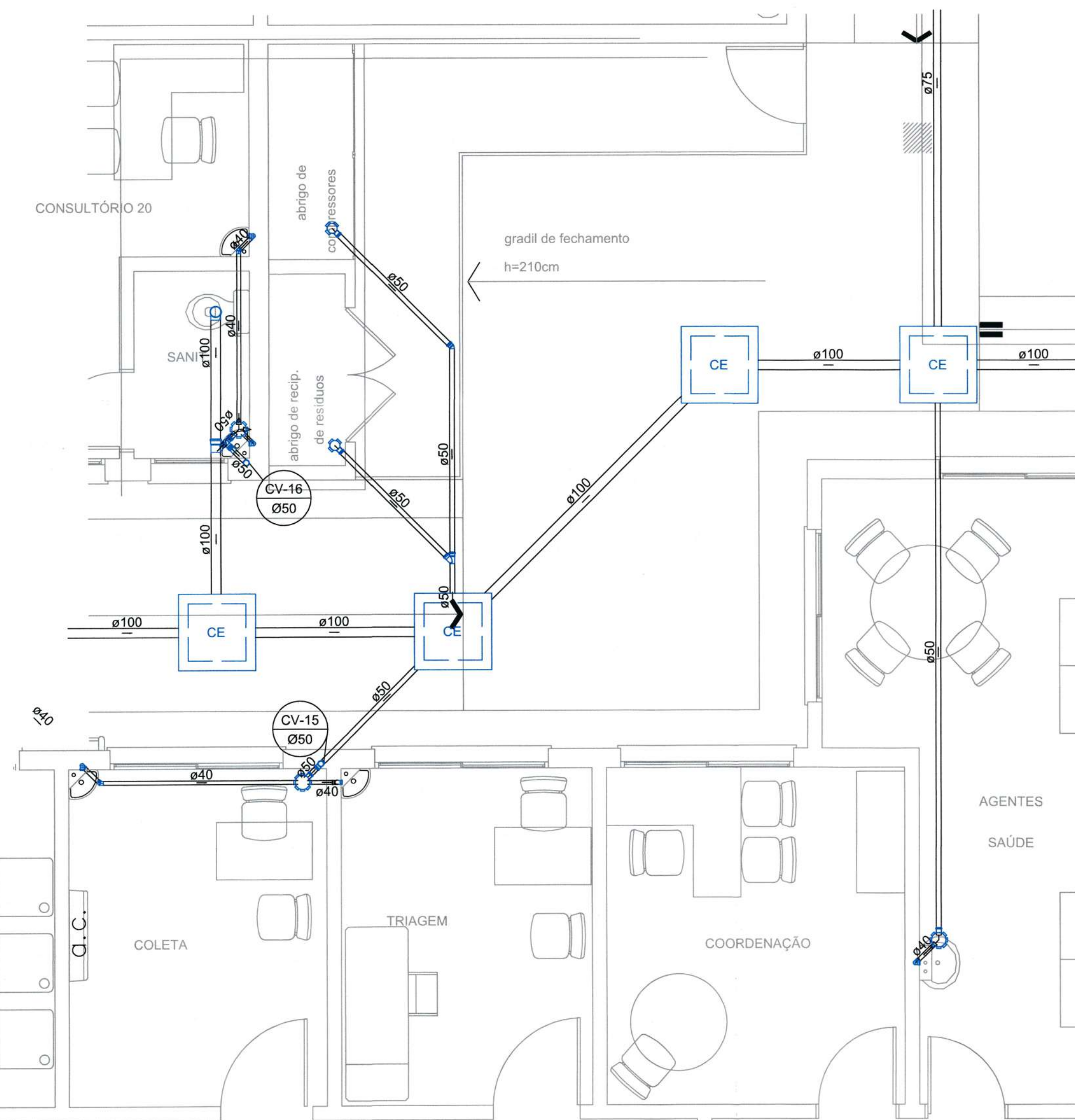
DETALHE S12
