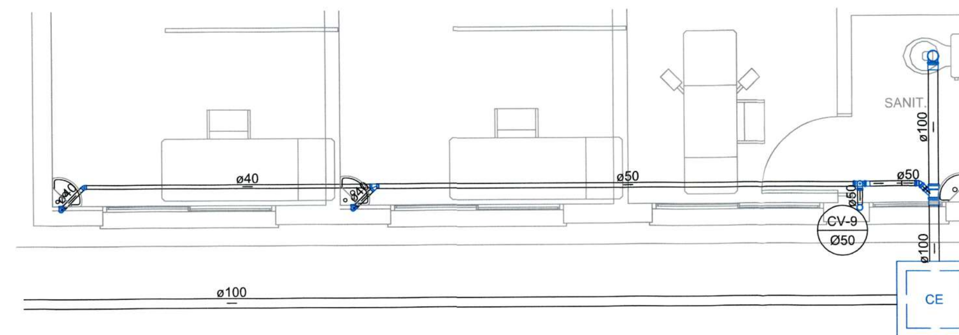
DETALHE S7
