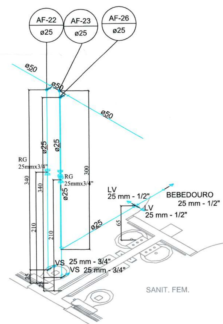
DETALHE H6
