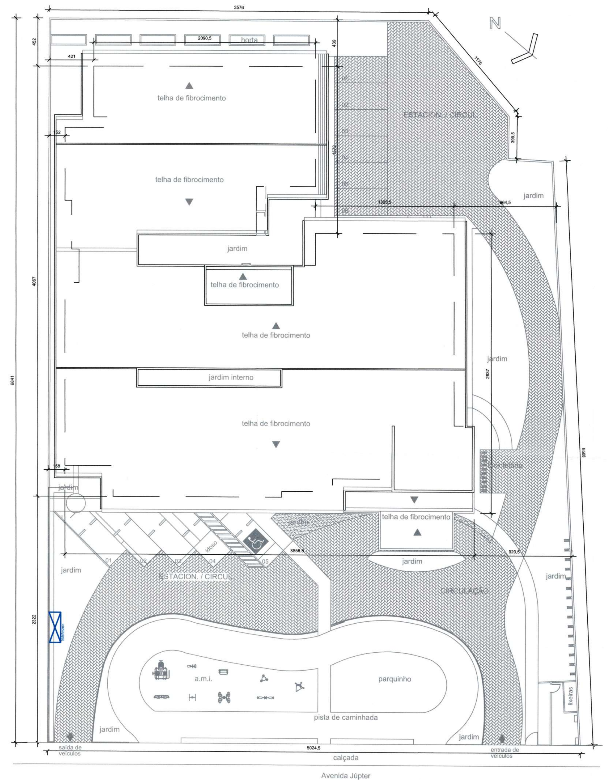
IMPLANTAÇÃO Escala 1/200
