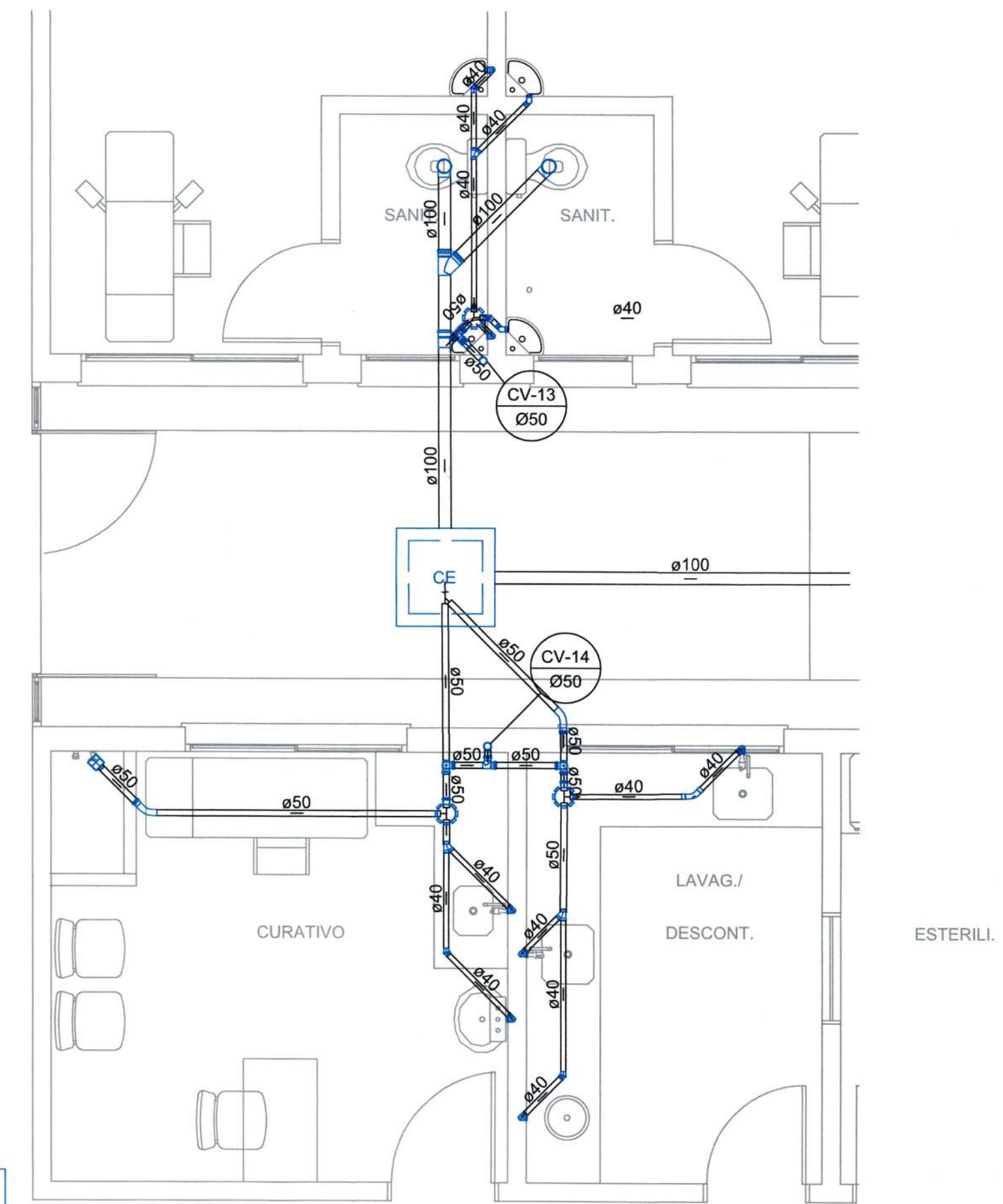
DETALHE S11
