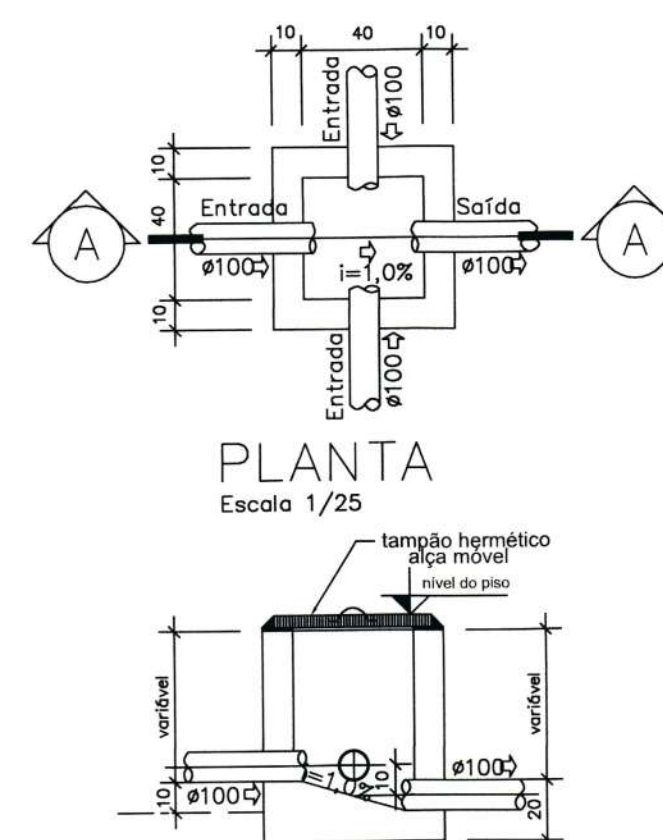
CAIXA DE INSPEÇÃO E PASSAGEM Escala 1/20
