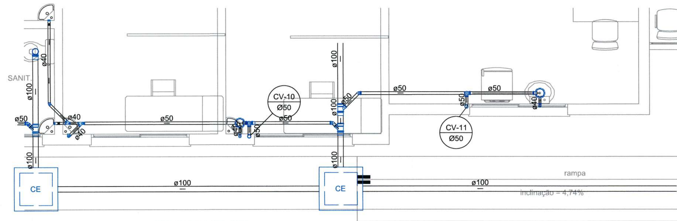
DETALHE S8
