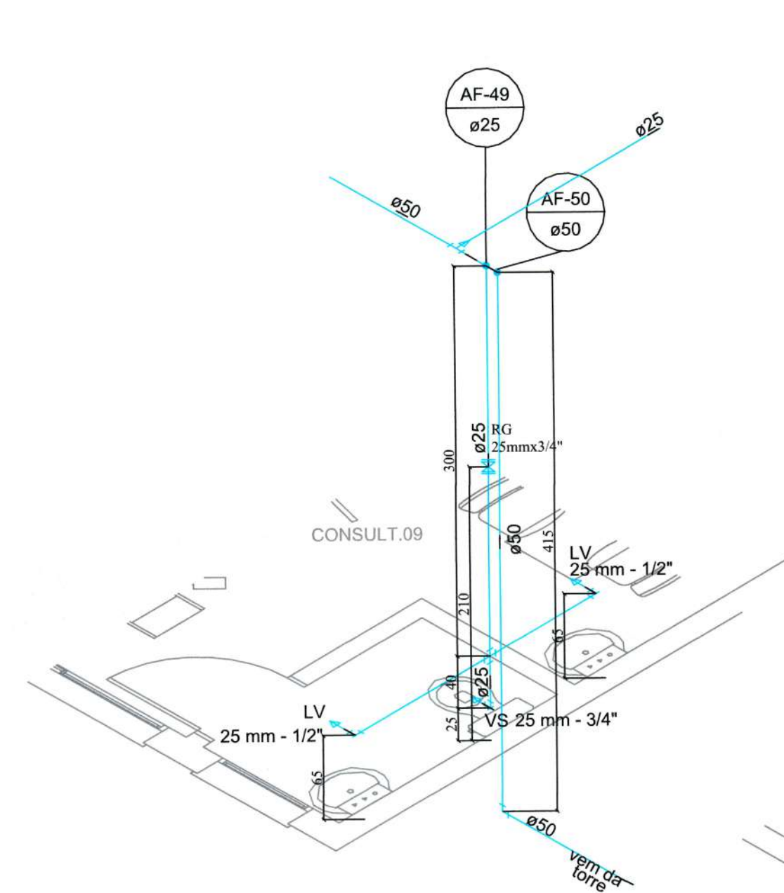
DETALHE H9
