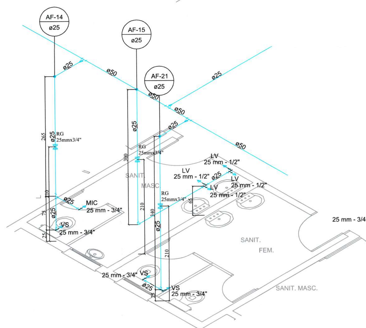
DETALHE H5
