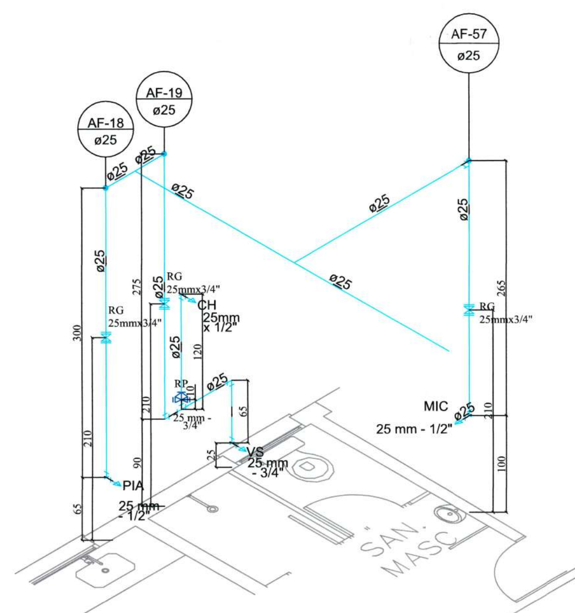
DETALHE H20
