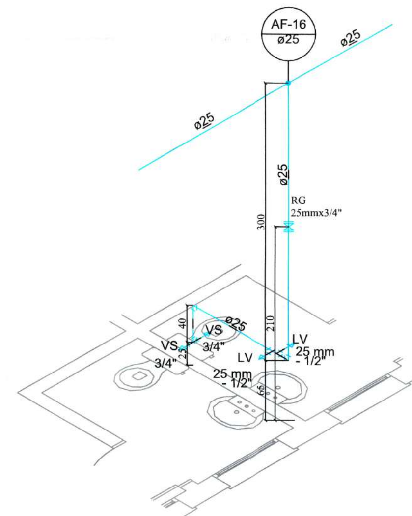
DETALHE H22
