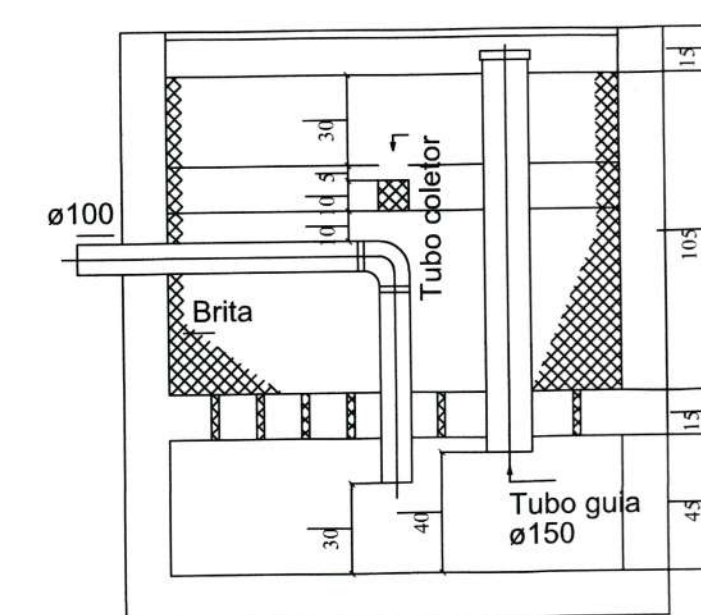
FILTRO ANAERÓBIO CORTE - ESC. 1:25
