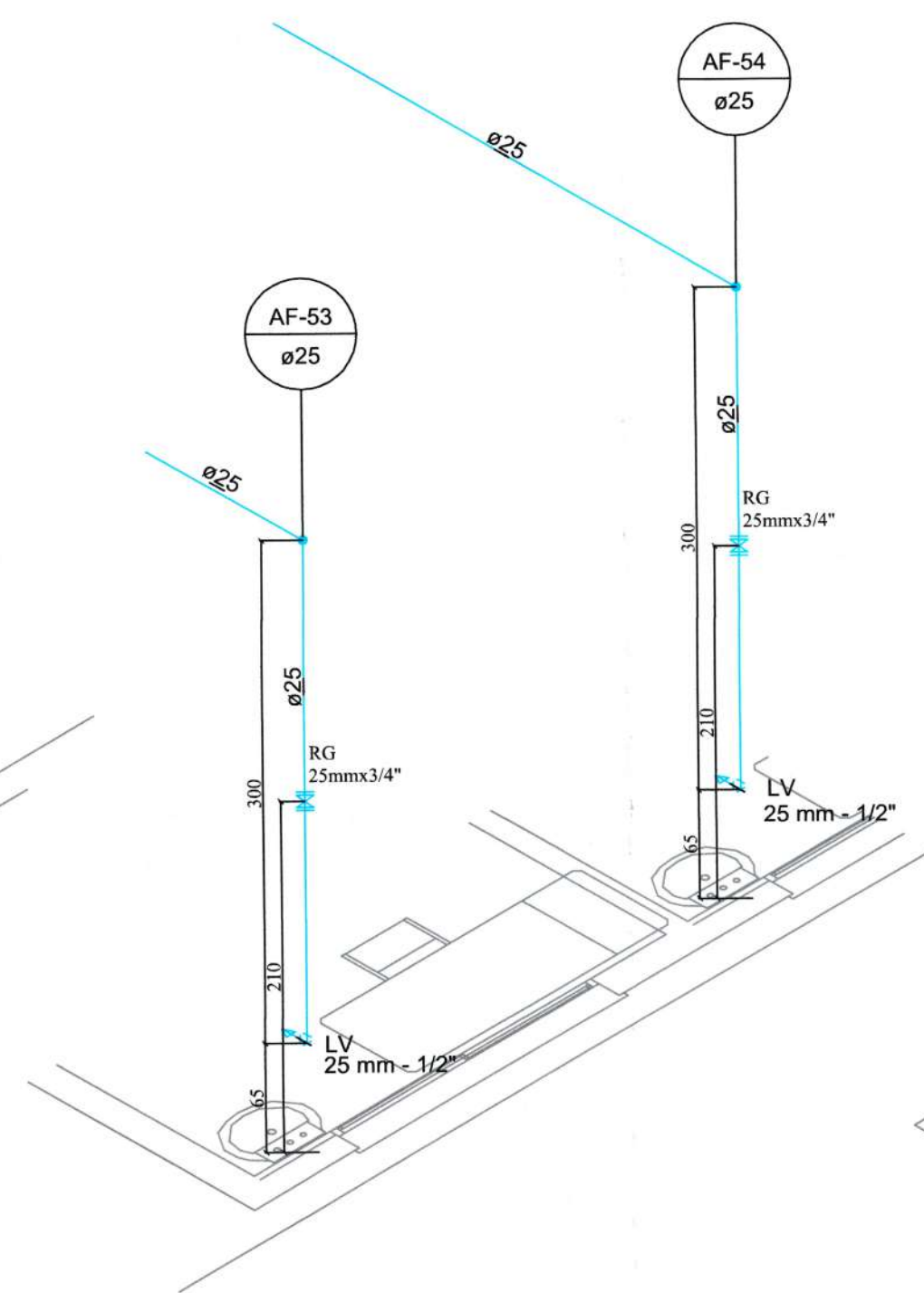
DETALHE H10
