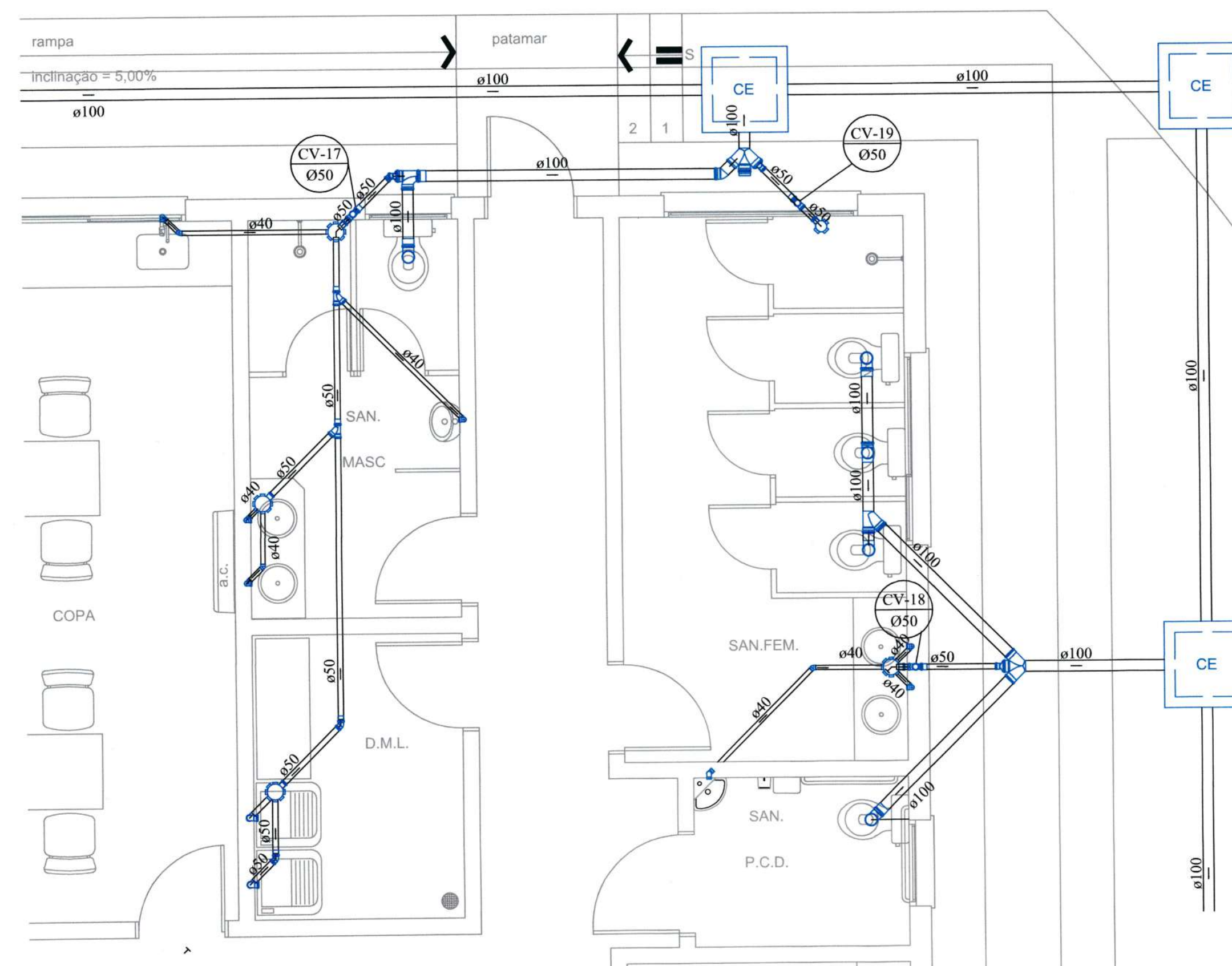
DETALHE S13
