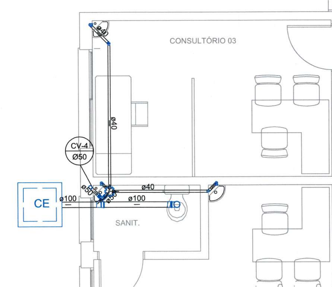
DETALHE S3
