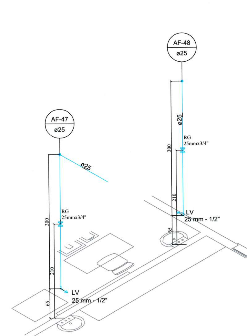
DETALHE H13
