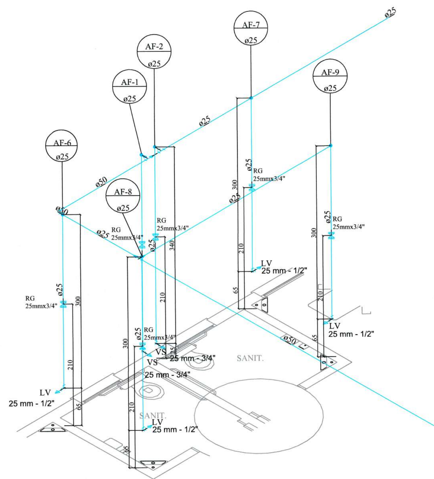
DETALHE H1
