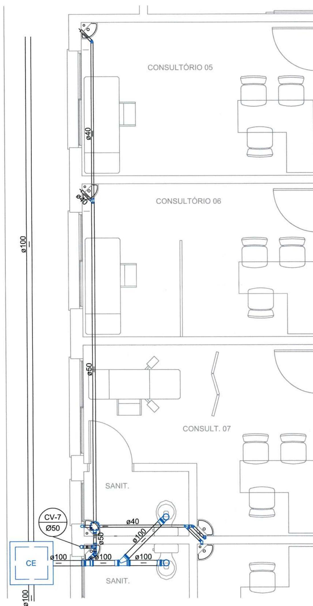
DETALHE S5 OBS.: INCLINAÇÃO MÍNIMA=1%
