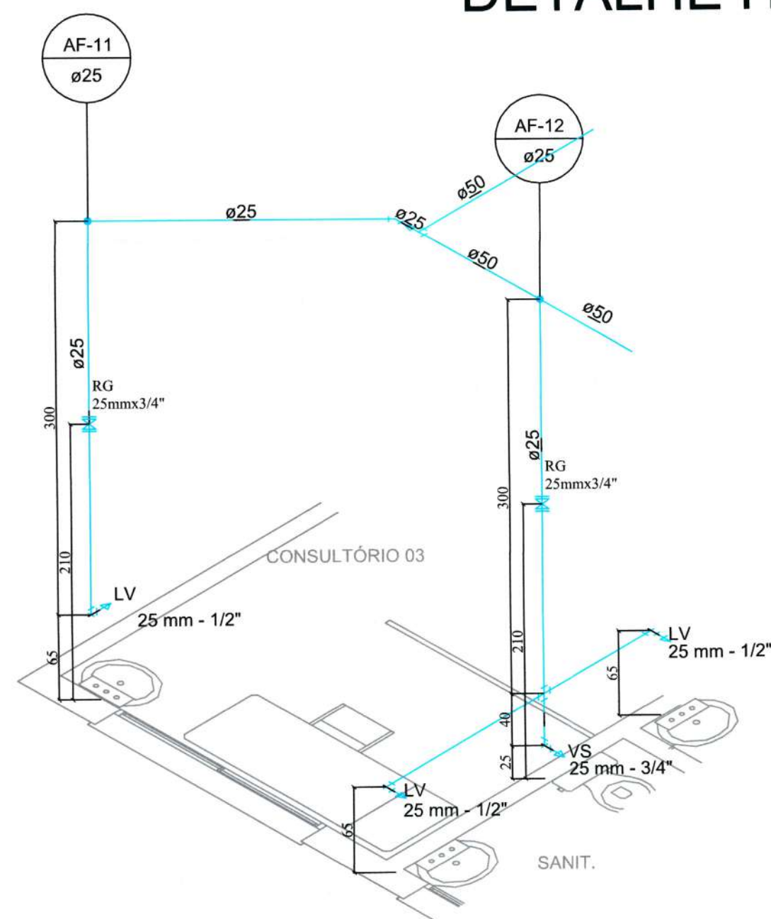
DETALHE H4
