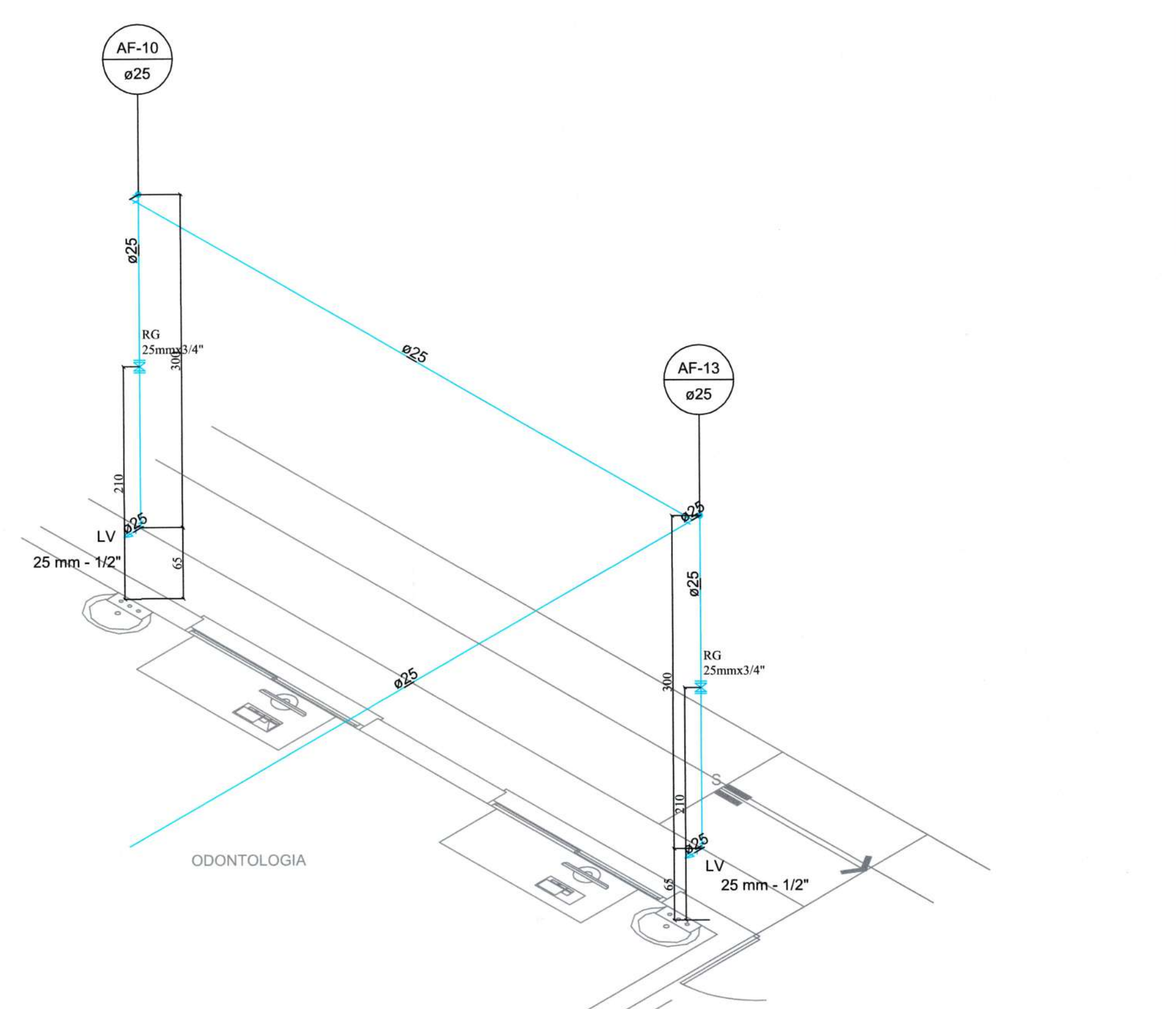
DETALHE H3
