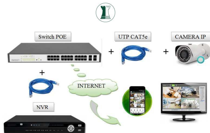
Figura 06 - Sistema CFTV
