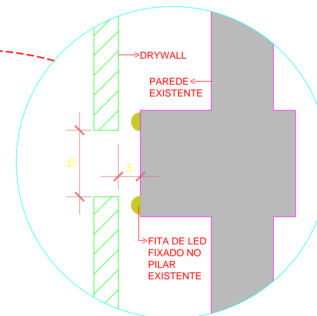
Detalhe de iluminação por LED escala 1:5
