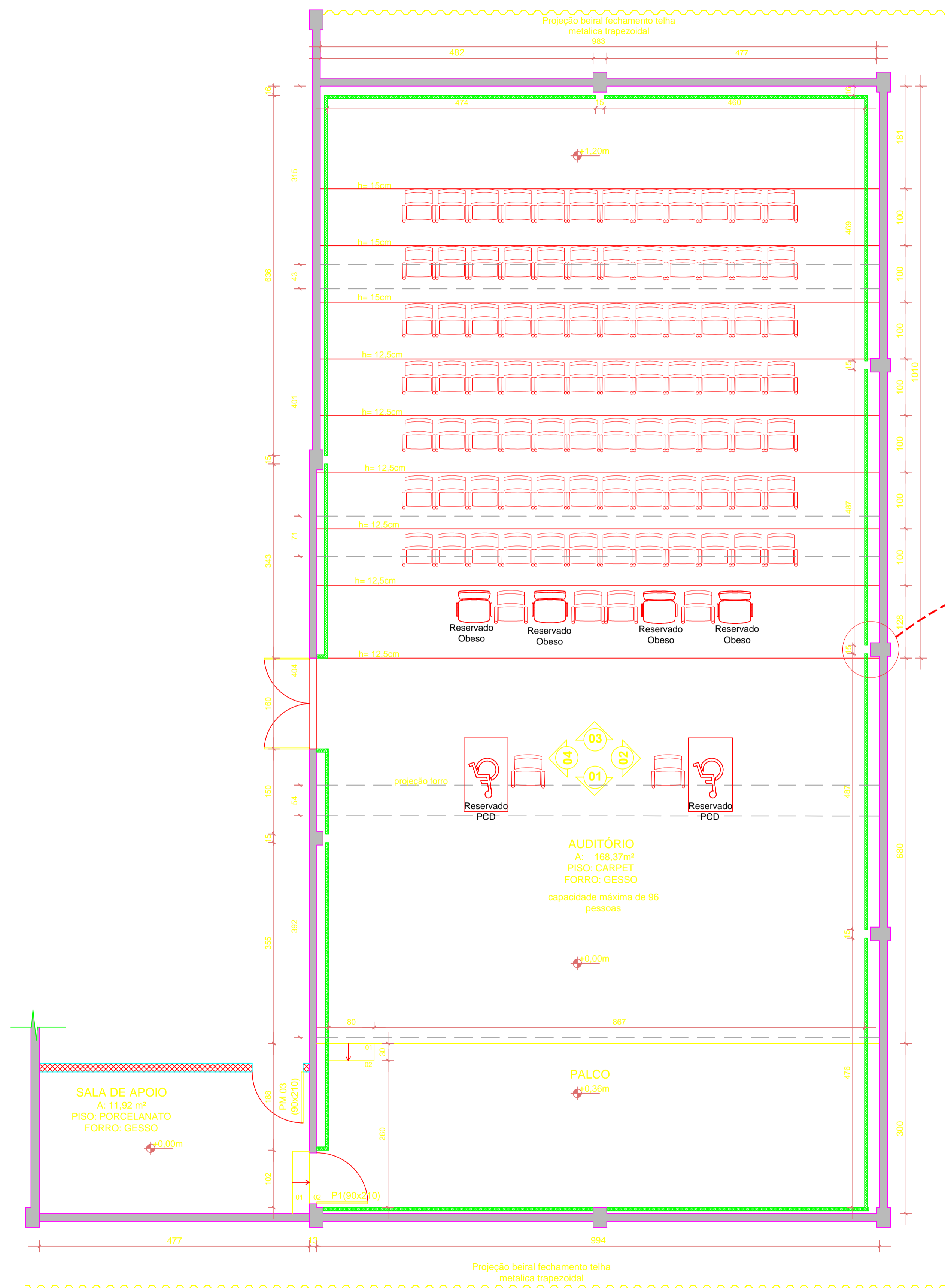
PLANTA BAIXA - AUDITÓRIO escala 1:50
