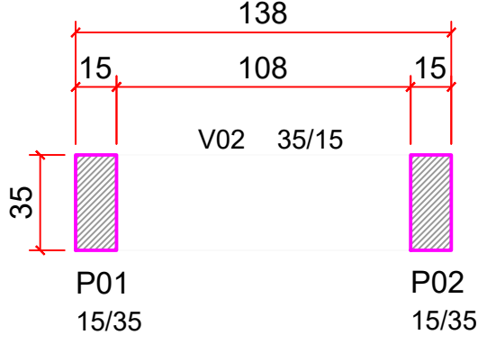
COBERTURA - MURETA ESC.: 1/25
