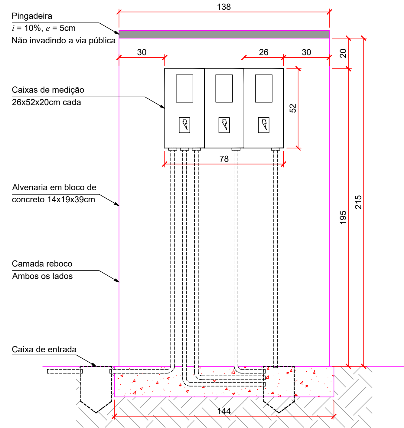
VISTA - MURETA ESC.: 1/15
