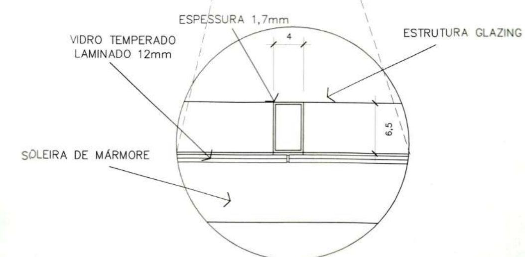
DETALHAMENTO - MONTANTE DA ESTRUTURA GLAZING Escala 1/5
