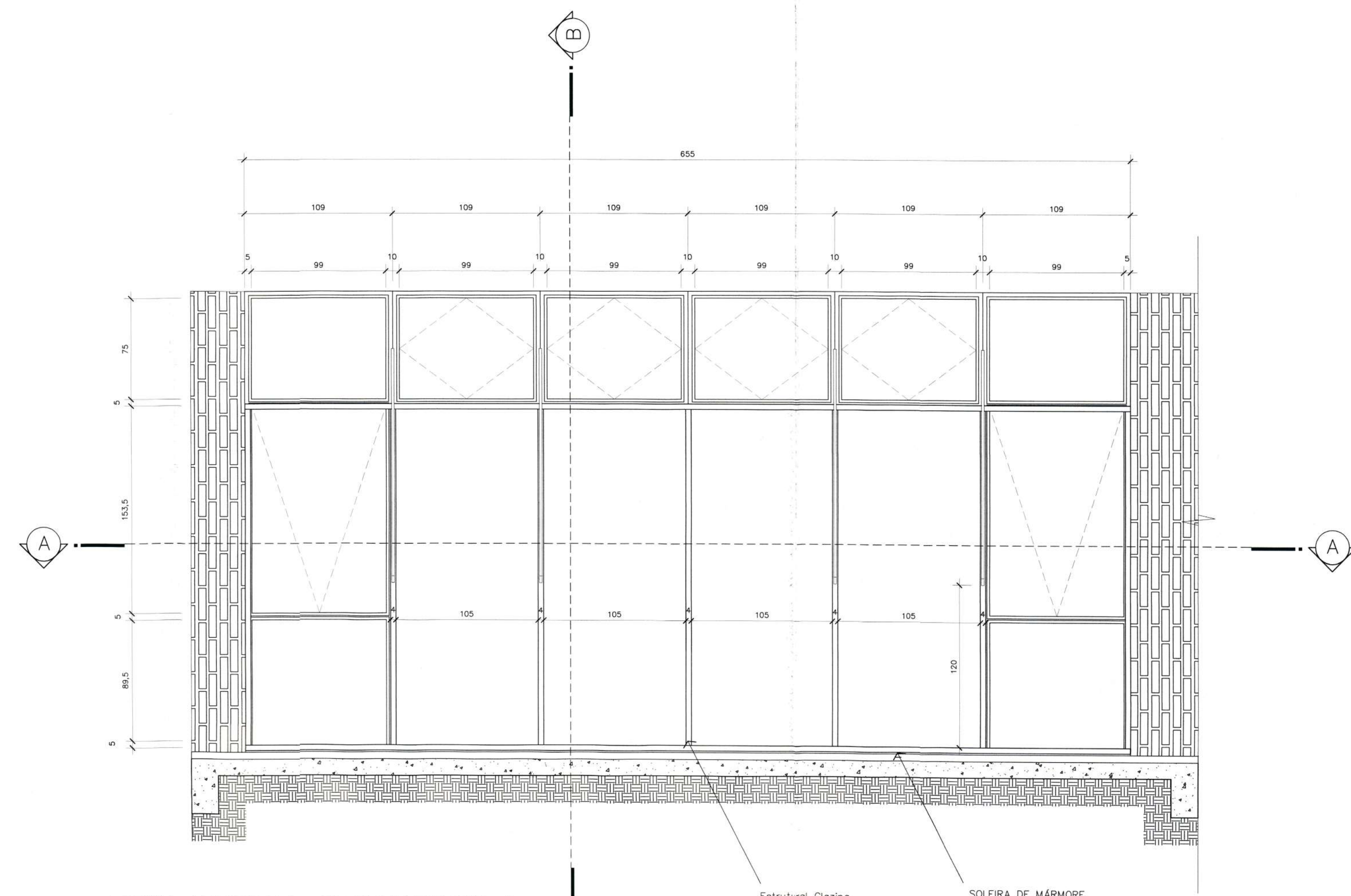
VISTA INTERNA-FECHAMENTO 1 Escala 1/25
