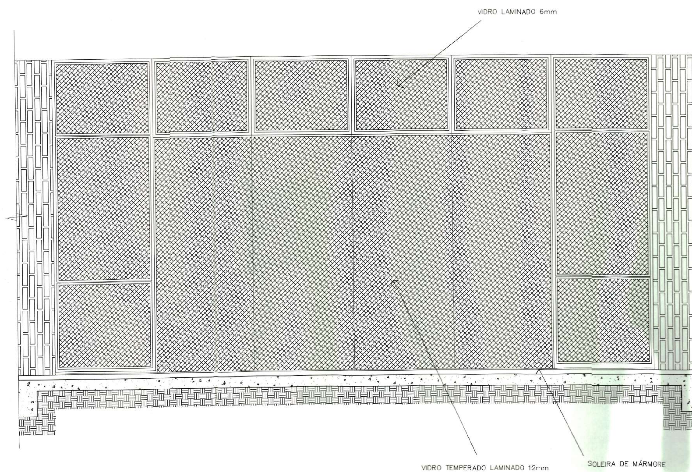
VISTA EXTERNA-FECHAMENTO 1 Escala 1/25
