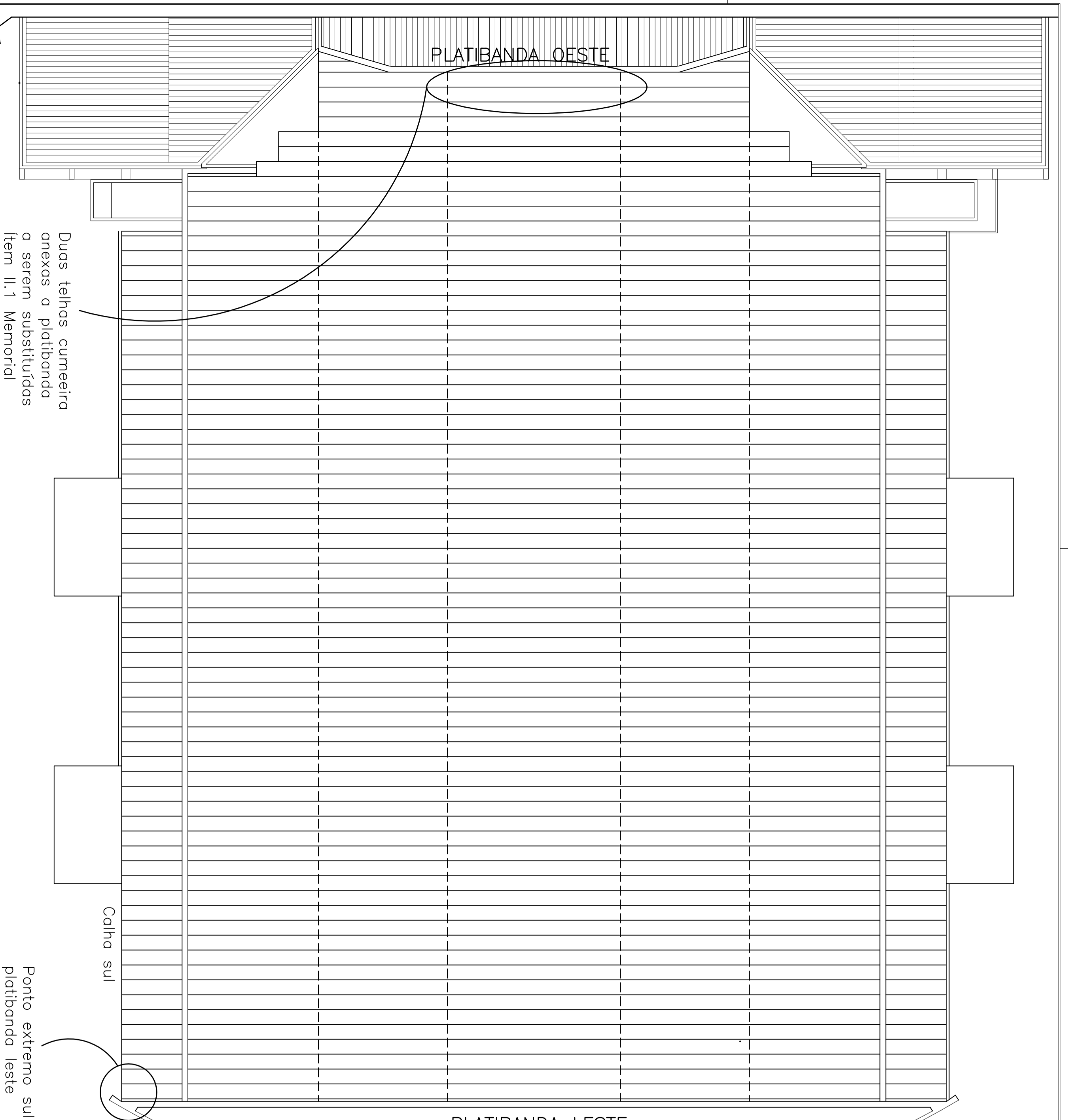
Vista superior Telhado 1:200
