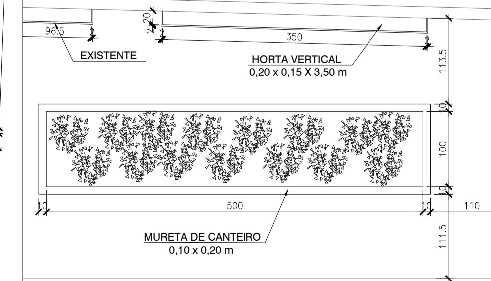
DET. DE HORTA ESC: 1:50
