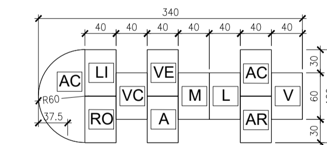
DET. AMARELINHA ESC 1:50
