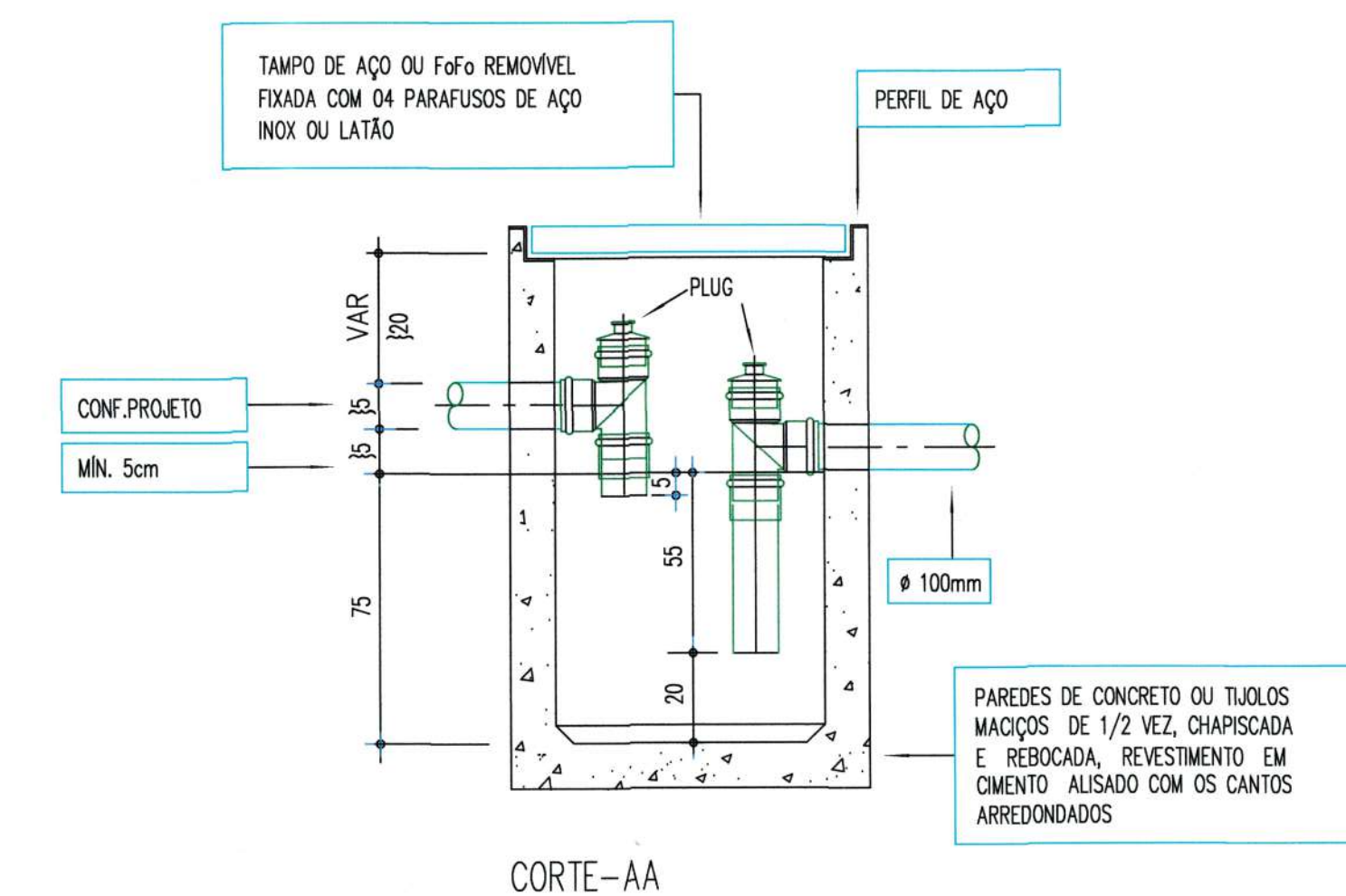
DETALHE DA CAIXA RETENTORA DE GORDURA SEM ESCALA
