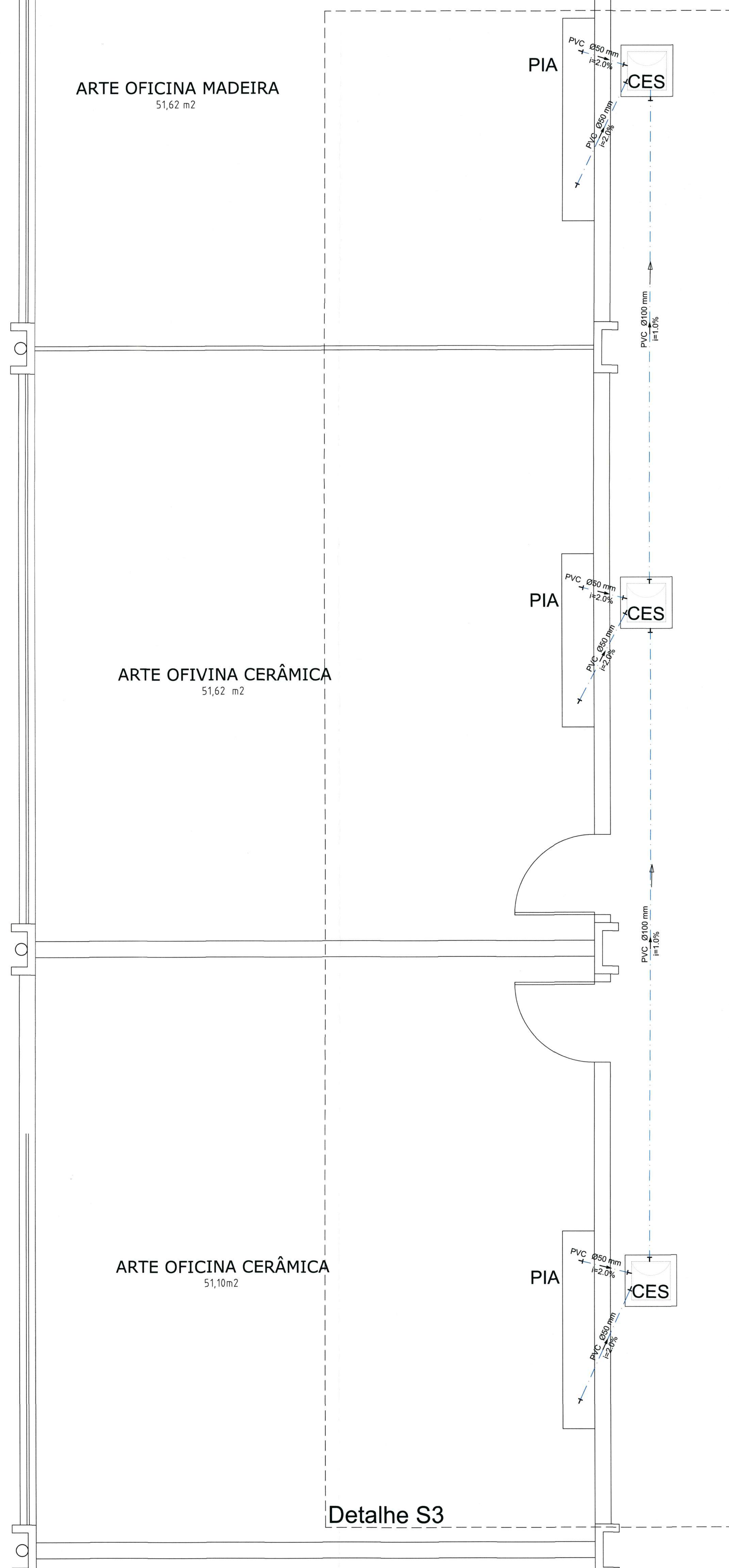
PLANTA DE IMPLANTAÇÃO - CAPTAÇÃO DE ESGOTOS Escala 1:25
