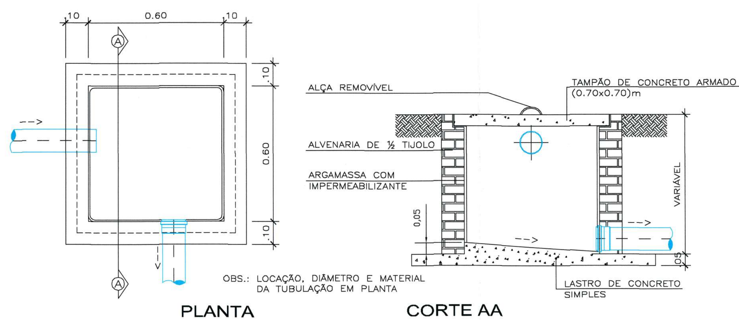
DETALHE CAIXA PASSAGEM E INSPEÇÃO (CP) Escala 1:25
