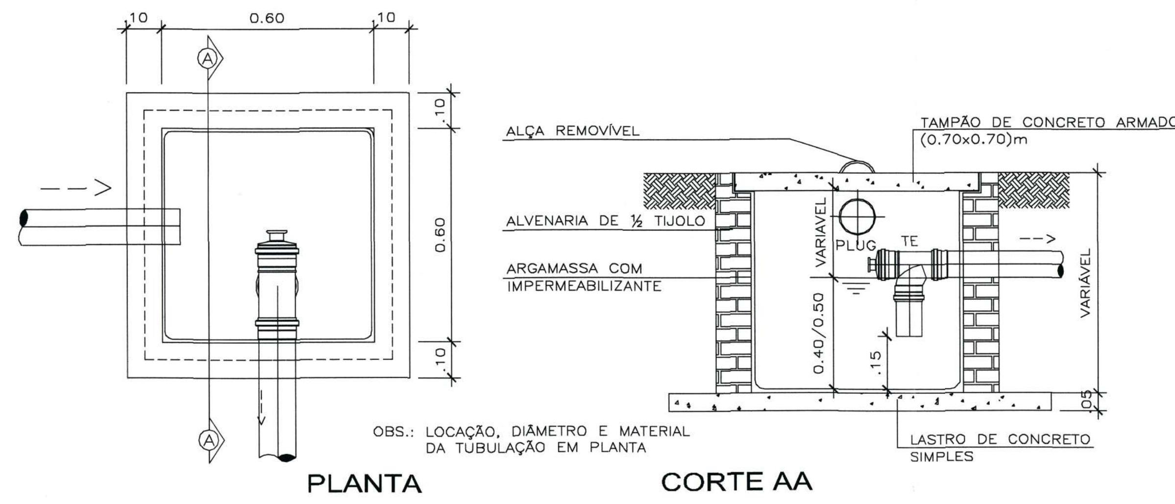
DETALHE CAIXA SIFONADA (CES) Escala 1:25
