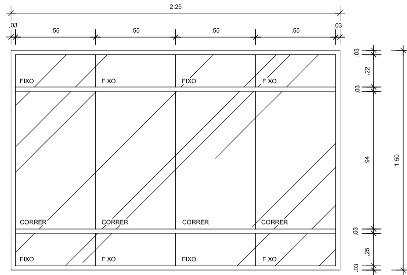
J01 225x150 Janelas - Salas Vidro Incolor 4mm Escala 1 1:25
