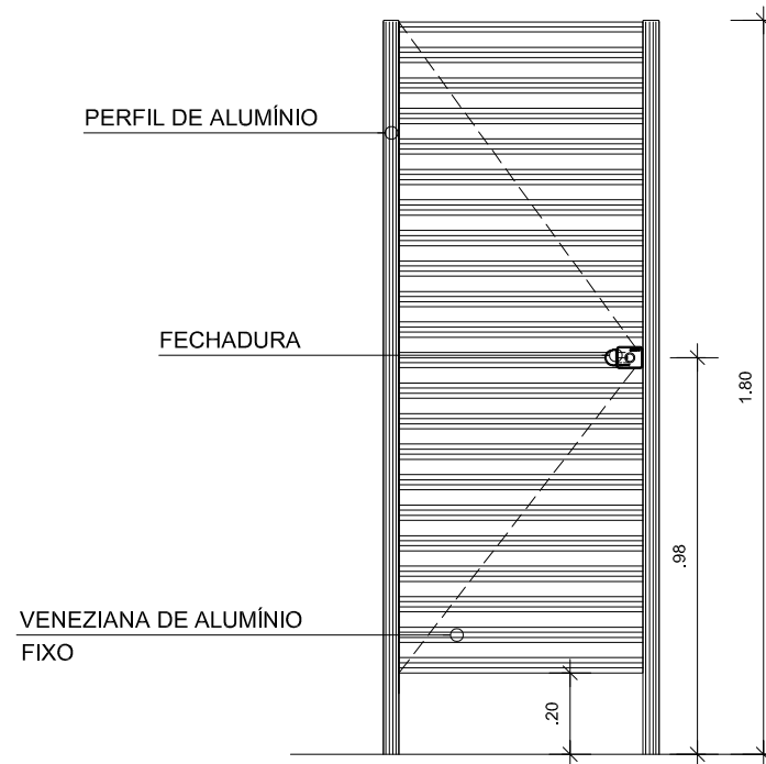
P03 60x160 Veneziana em Alumínio - Cabine dos banheiros Pintura eletrostática cor branca Escala 1 1:20
