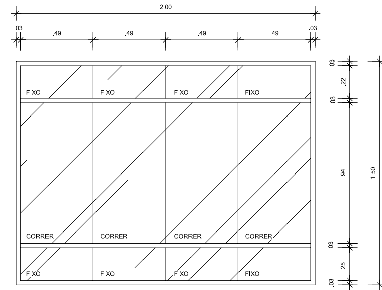
J02 200x150 Janelas - Salas Vidro Incolor 4mm Escala 1 1:25
