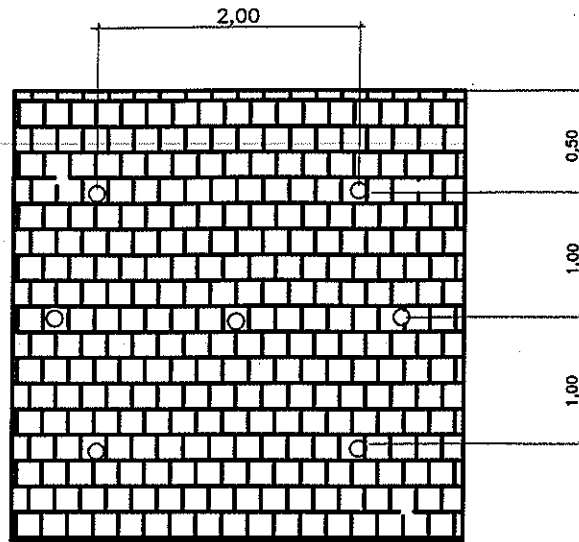
VISTA FRONTAL SISTEMA DRENAGEM BARBACANS
