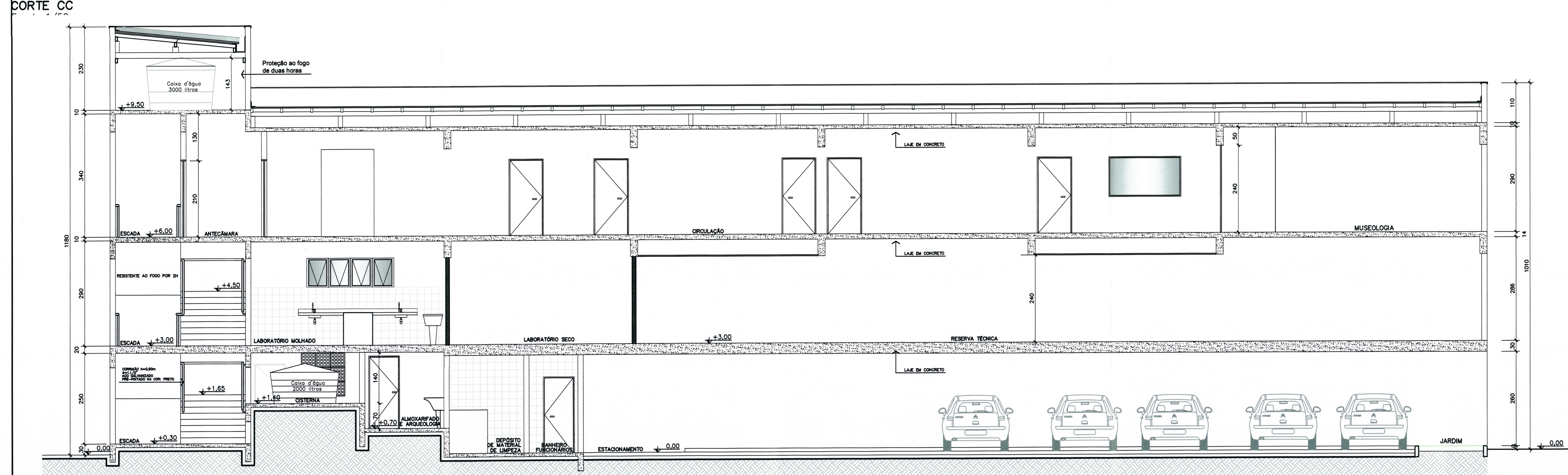
CORTE DD Escala 1/50
