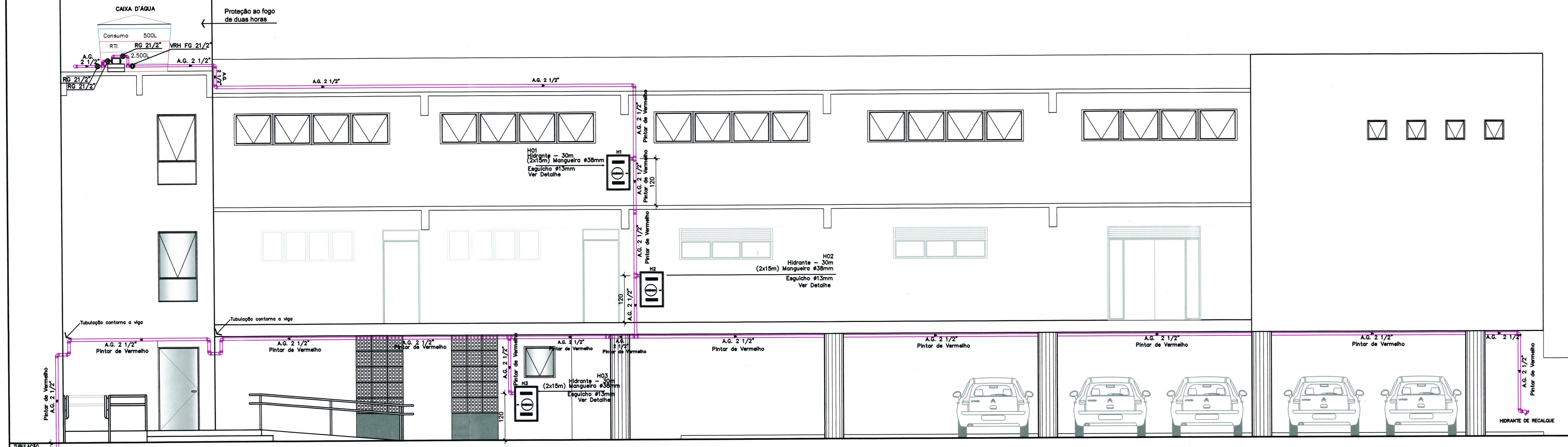
CORTE COM OS HIDRANTES Escala 1/50
