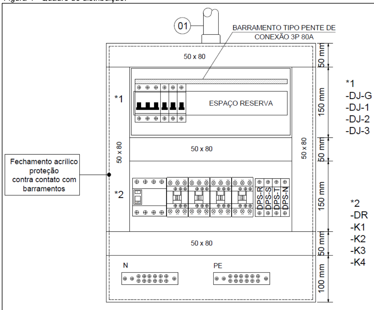
Figura 4 - Quadro de distribuição.
