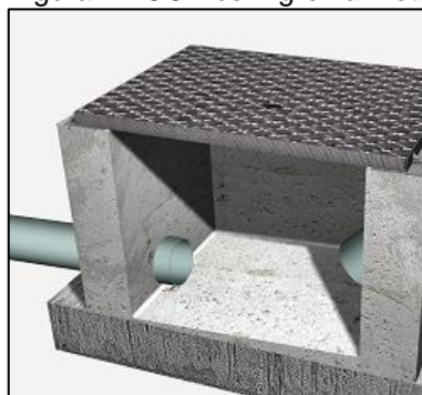
Figura 2 - CCP com grelha metálica.
