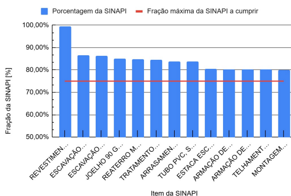
Figura 2 - Dados da Tabela 3 apresentados em forma gráfica.
