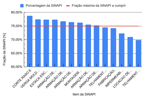
Figura 1 - Dados da Tabela 2 apresentados em forma gráfica.
