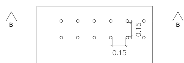
DETALHE DO FUNDO FALSO ESCALA - SEM ESCALA
