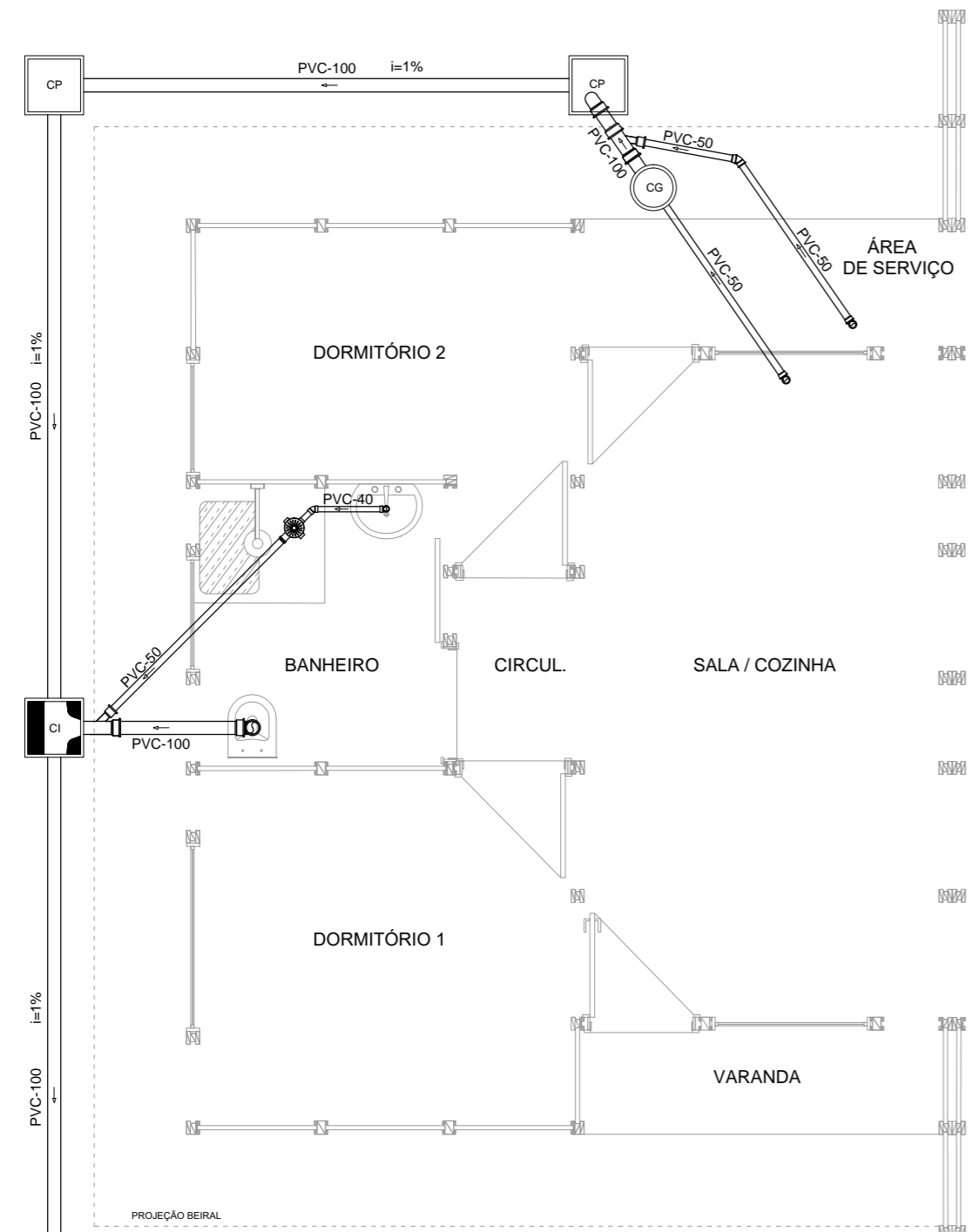
PLANTA BAIXA - PROJETO SANITÁRIO DA UNIDADE ACESSÍVEL ESCALA 1:50
