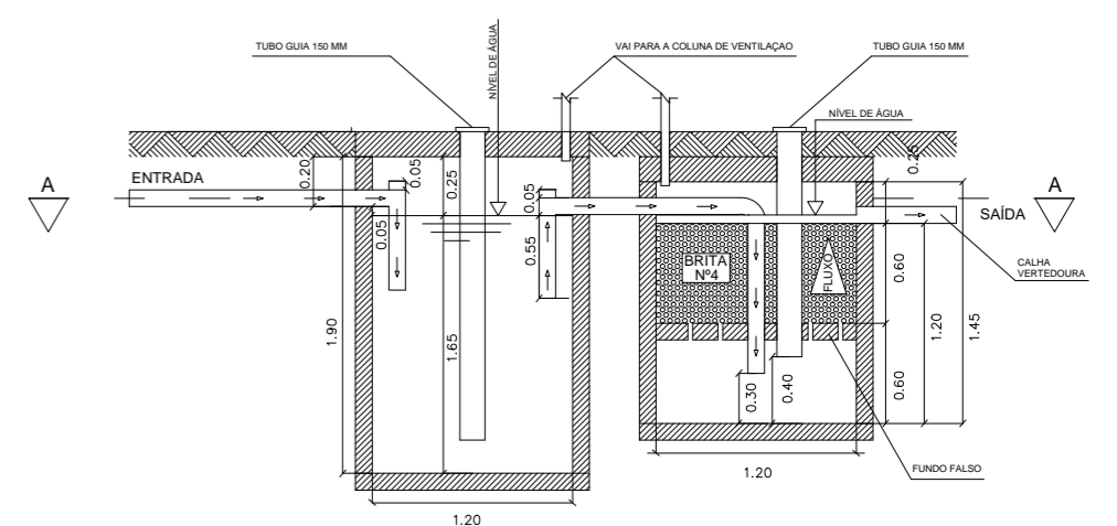
SEÇÃO TRANSVERSAL - DETALHE DA FOSSA SÉPTICA / FILTRO ANAERÓBICO ESCALA - SEM ESCALA
