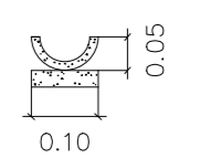
PERFIL DA CALHA VERDEDOURA ESCALA - SEM ESCALA
