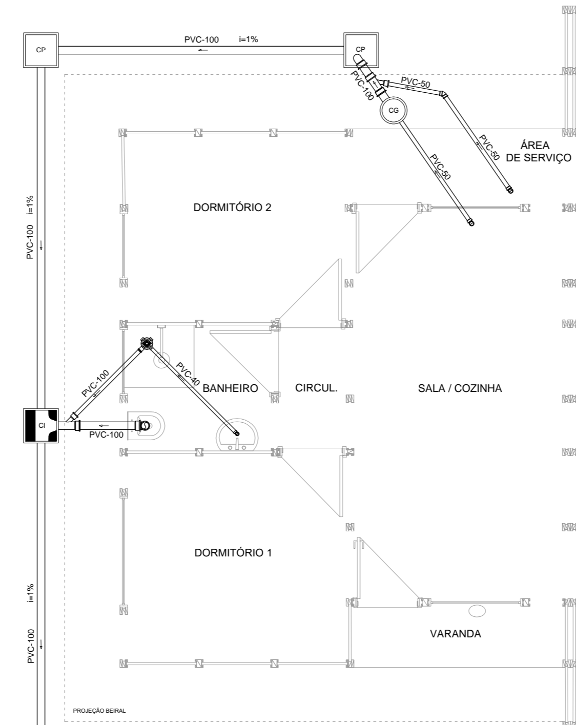
PLANTA BAIXA - PROJETO SANITÁRIO DA UNIDADE ISOLADA ESCALA 1:50
