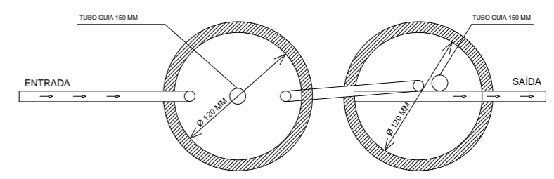
CORTE A - A - DETALHE DA FOSSA SÉPTICA / FILTRO ANAERÓBICO ESCALA - SEM ESCALA
