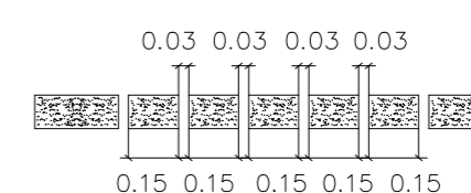
CORTE B - B - DETALHE DA FOSSA SÉPTICA / FILTRO ANAERÓBICO ESCALA - SEM ESCALA
