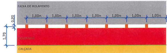
DETALHE G LINHA DE MARCAÇÃO DE CICLOFAIXA PARA CRUZAMENTO
