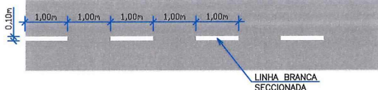
DETALHE D LINHA SIMPLES CONTÍNUA AMARELA
