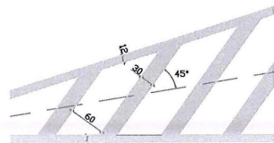
DETALHE DO ZEBRADO P/ PROTEÇÃO DO ESTACIONAMENTO
