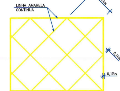
DETALHE DA MARCAÇÃO DE ÁREA DE CONFLITO
