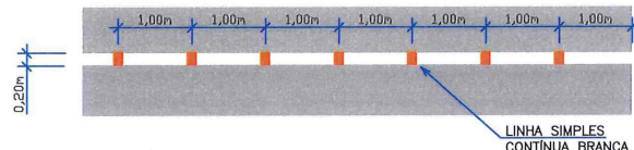
DETALHE G LINHA DE MARCAÇÃO DE CICLOFAIXA PARA CRUZAMENTO
