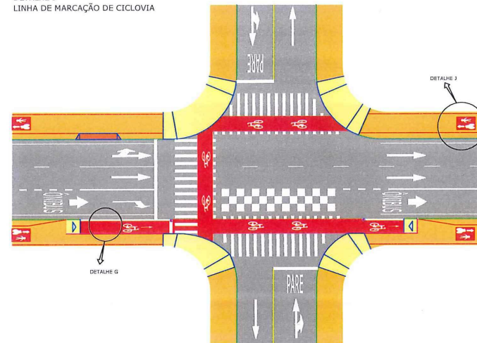
DETALHE I LINHA DE MARCAÇÃO DE CICLOVIA
