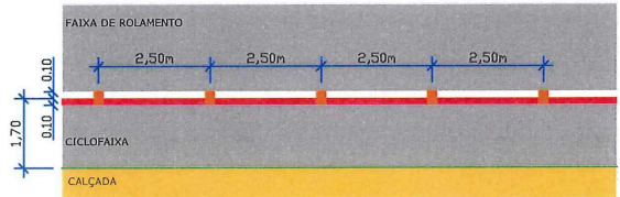
DETALHE H MARCAÇÃO DE CICLOFAIXA AO LONGO DA VIA
