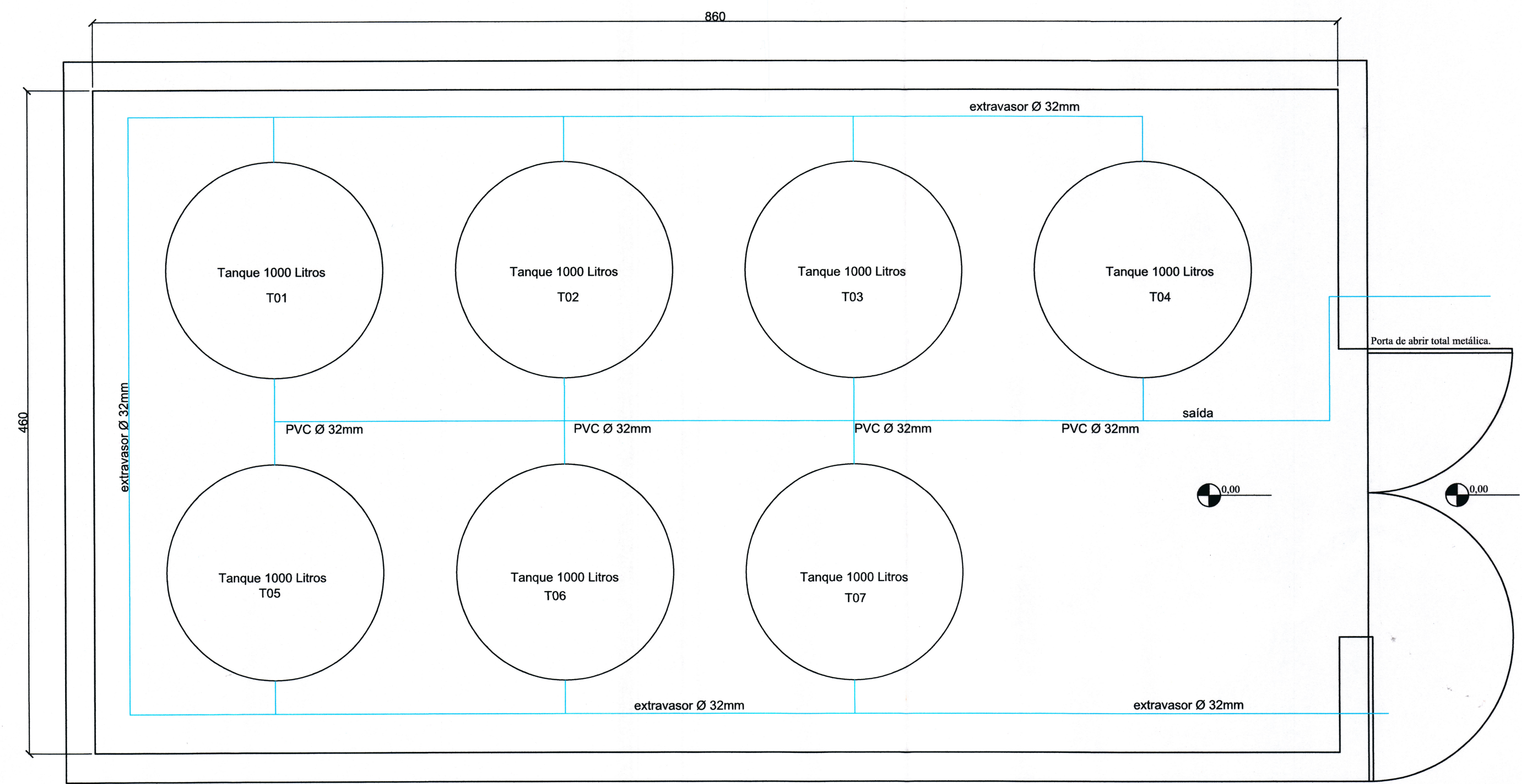
Planta baixa distribuição tanques esc. 1:25
