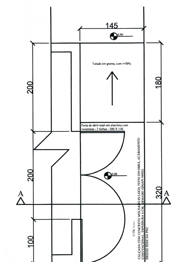
Planta baixa área externa porta de acesso esc. 1:50
