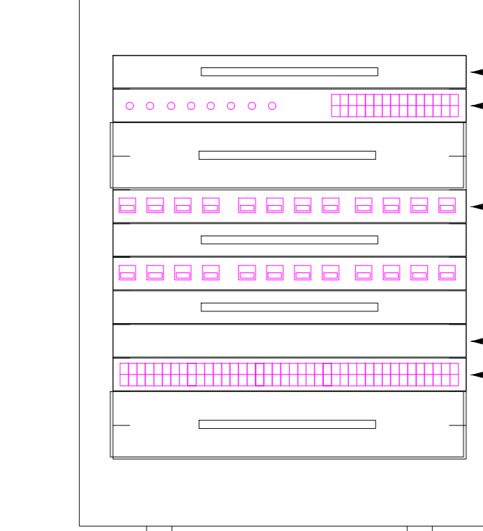
Plano de face do rack (BD1)
