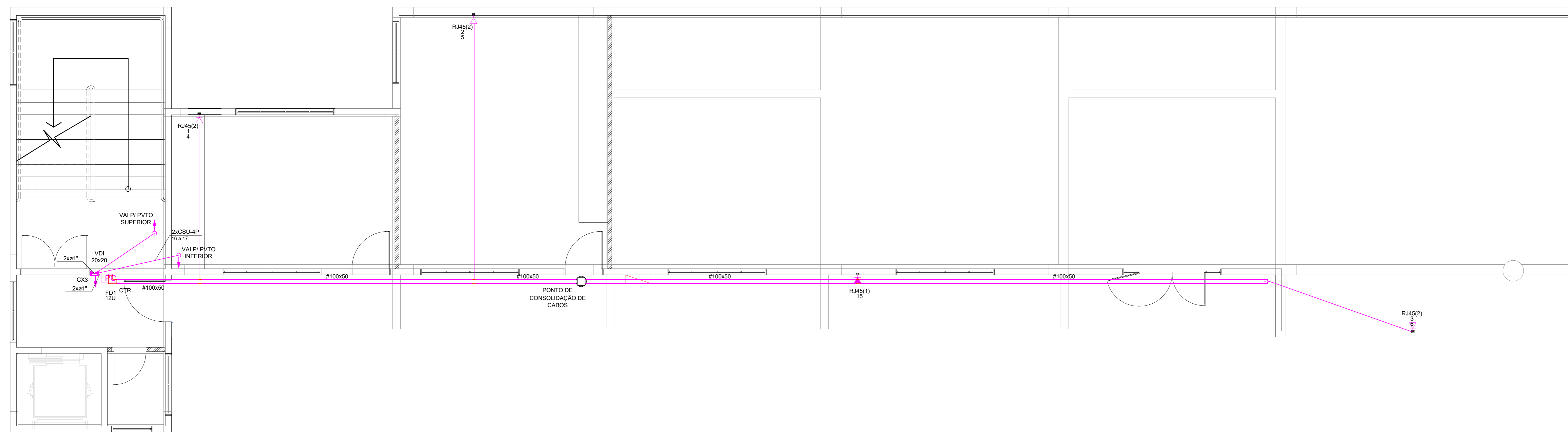
PLANTA BAIXA CABAMENTO ESTRUTURADO PRIMEIRO PVTO
