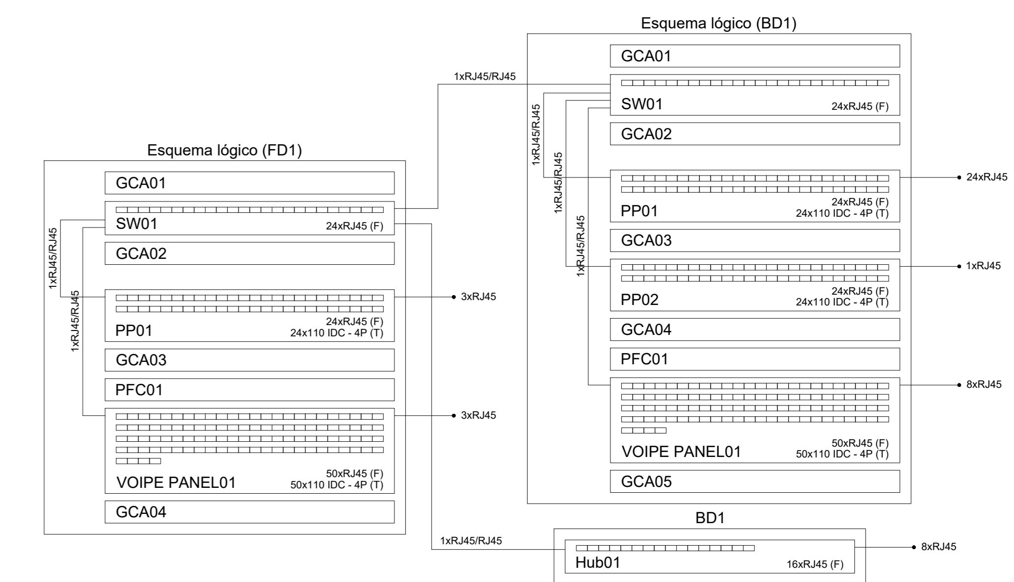
DETALHE ESQUEMA LÓGICO ESCALA 1:50
