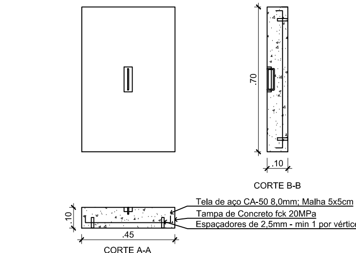
TAMPA DE CONCRETO 01 ESC. 1:20
