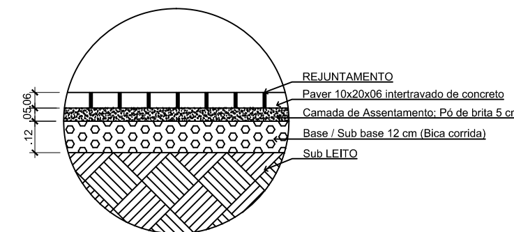
DETALHE DO PAVIMENTO (CALÇADA) ESC. 1:20
