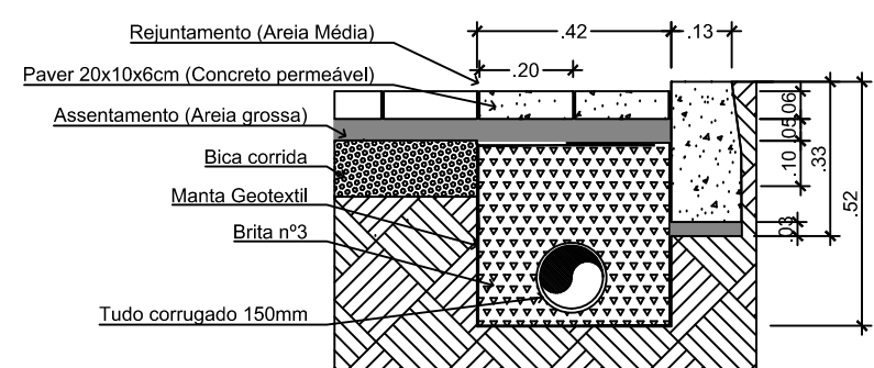
VALA DE DRENAGEM ESC. 1:20
