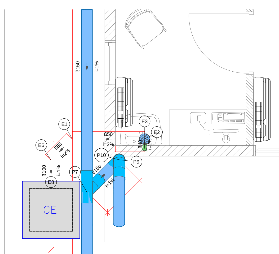
Detalhe Sanitário -4 Escala 1:25
