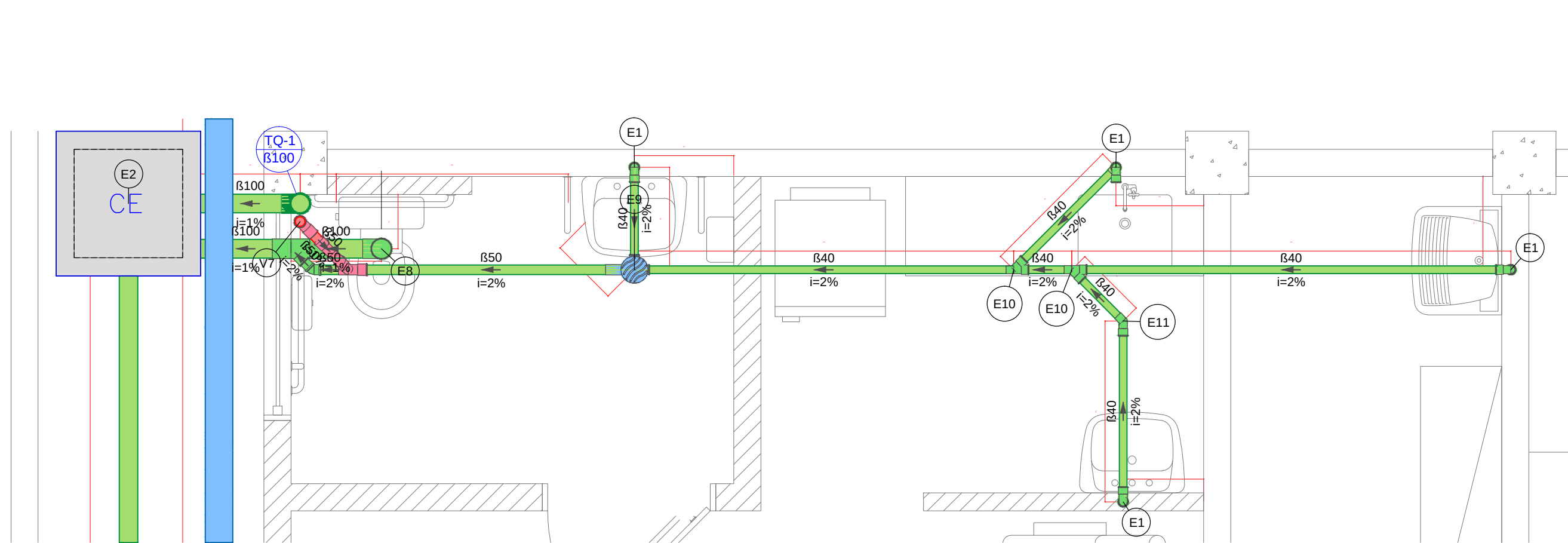
Detalhe Sanitário -1 Escala 1:25
