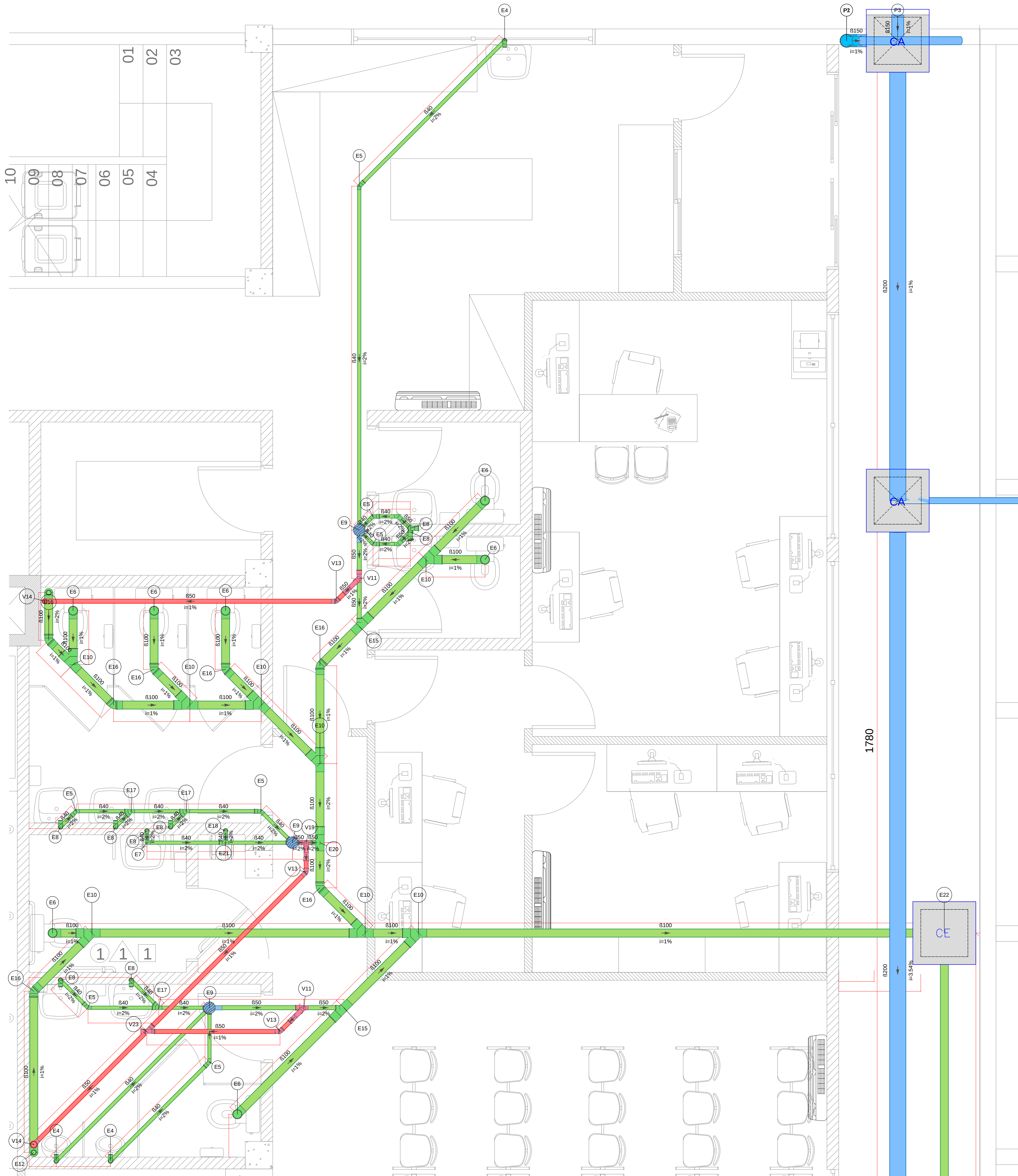
Detalhe Sanitário -2 Escala 1:25
