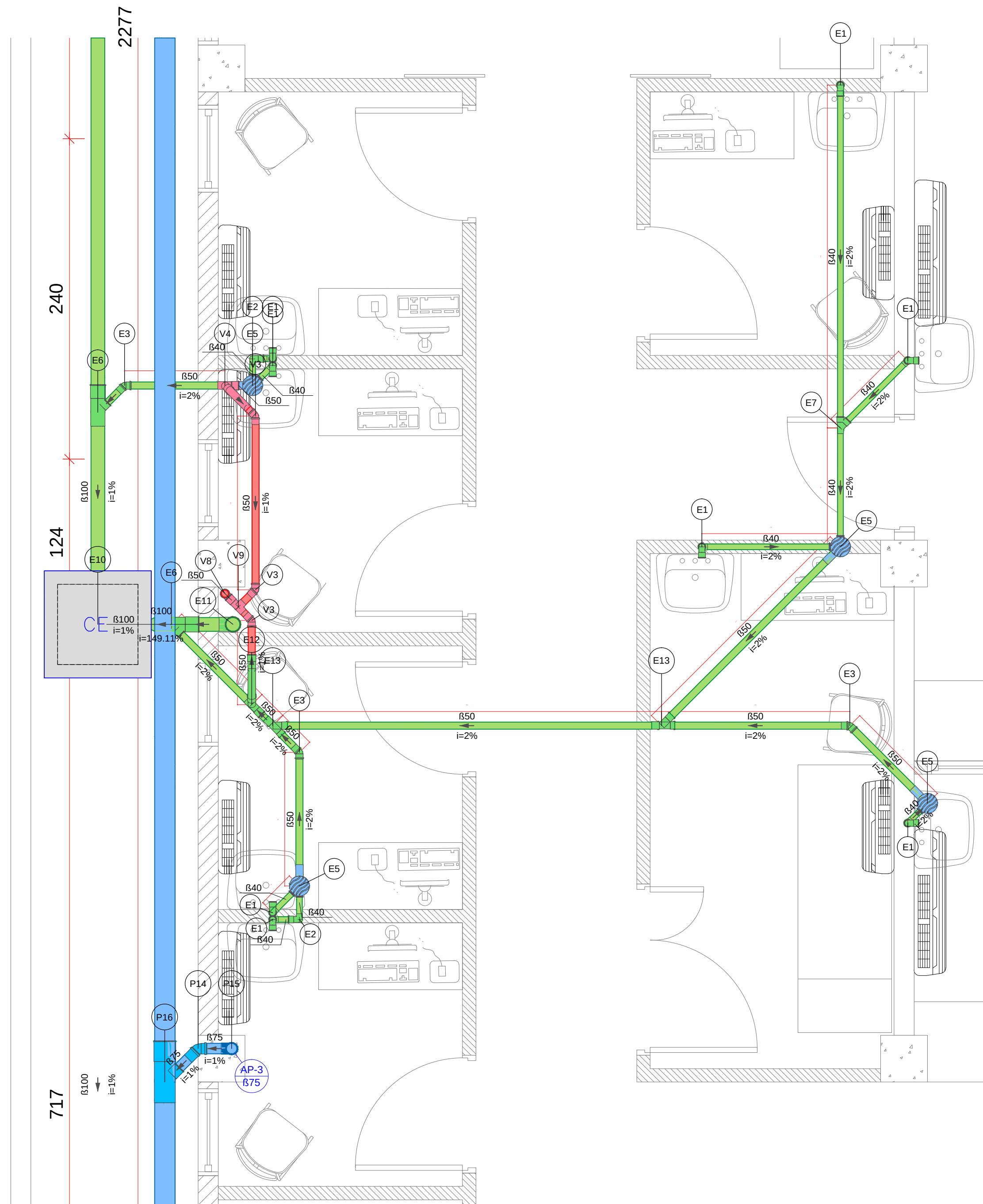
Detalhe Sanitário -3 Escala 1:25
