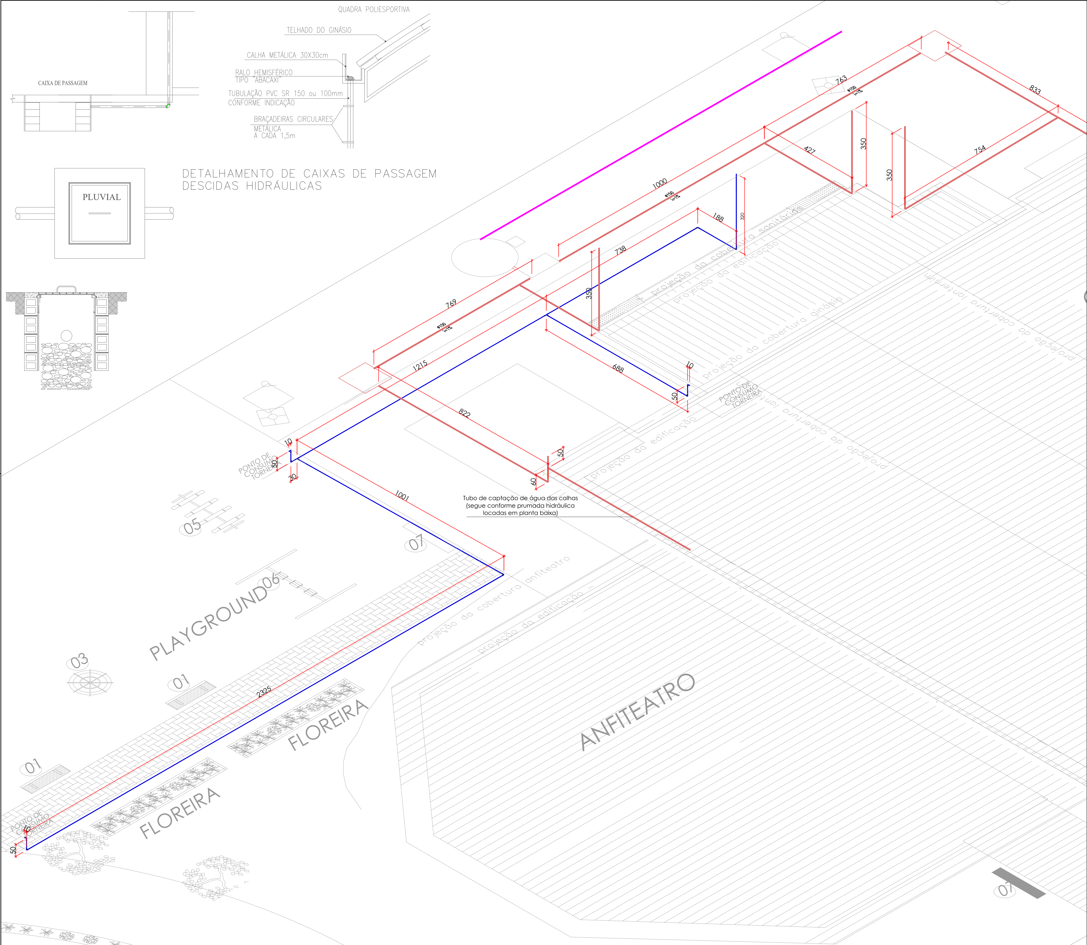
PLANTA DE REAPROVEITAMENTO DE ÁGUA DA CHUVA ESCALA: 1:100
