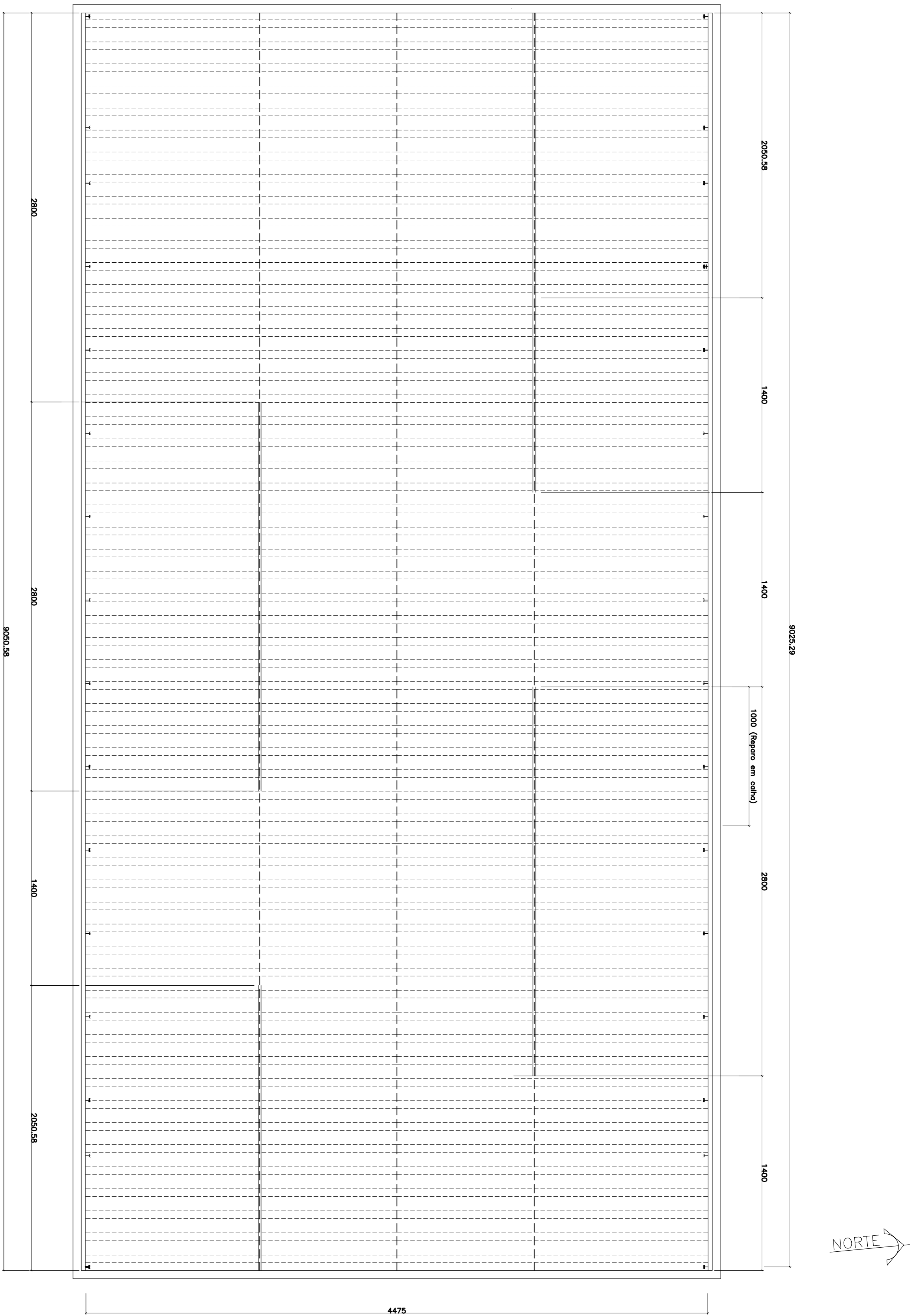
Vista superior Telhado Mapeamento troca manta 1:200
