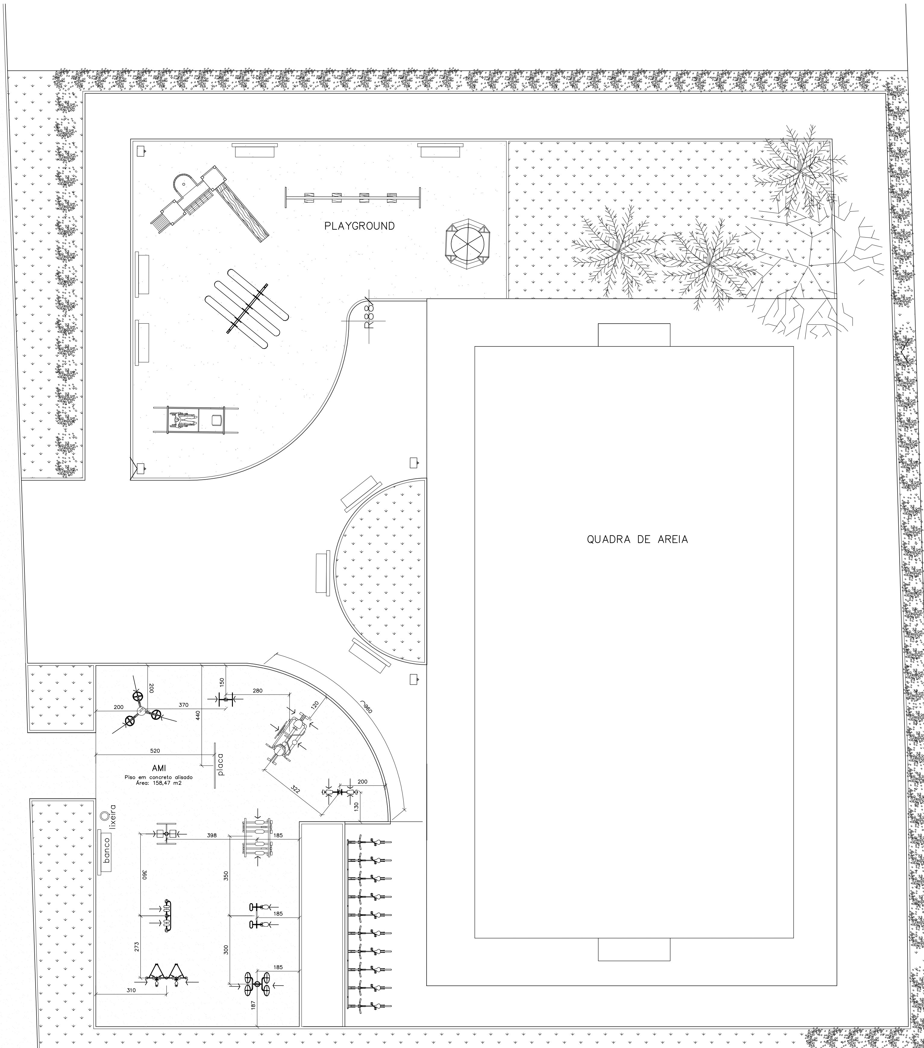
IMPLANTAÇÃO Escala 1/100
